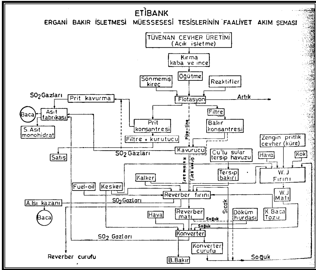
Şema 1 – Eİİ Müessesesi Tesislerinin Faaliyet Akım Şeması ( Etiabank Bülteni dergisinden alınmıştır.)
