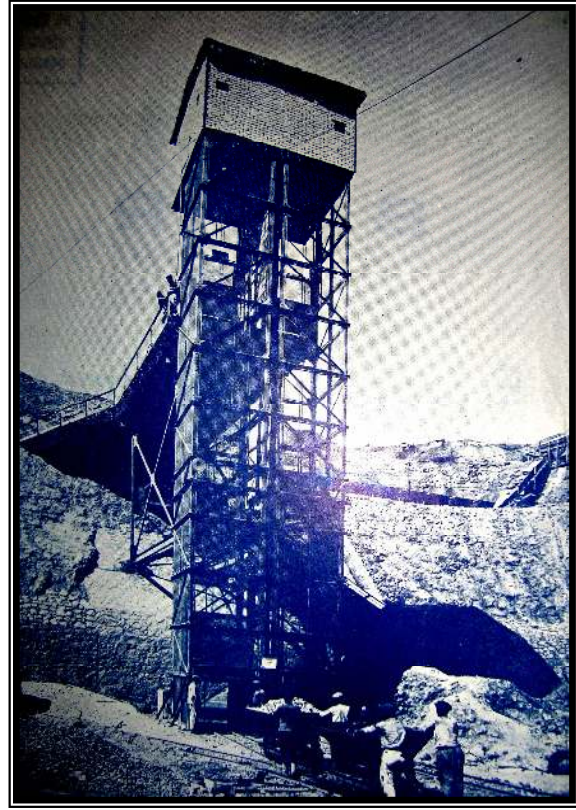
Resim 5 – Vagonların taşınması için yaptırılan asansör (Bakır 1949 adlı eserden alınmıştır.)
