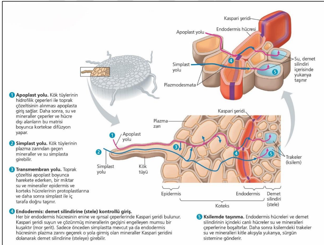
Şekil 2.1. Kökte mineral ve suyun yanal taşınımına (Urry vd., 2022).
