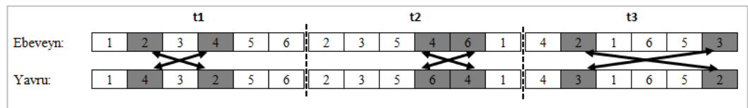
Şekil 5.11. Mutasyon operatörü
