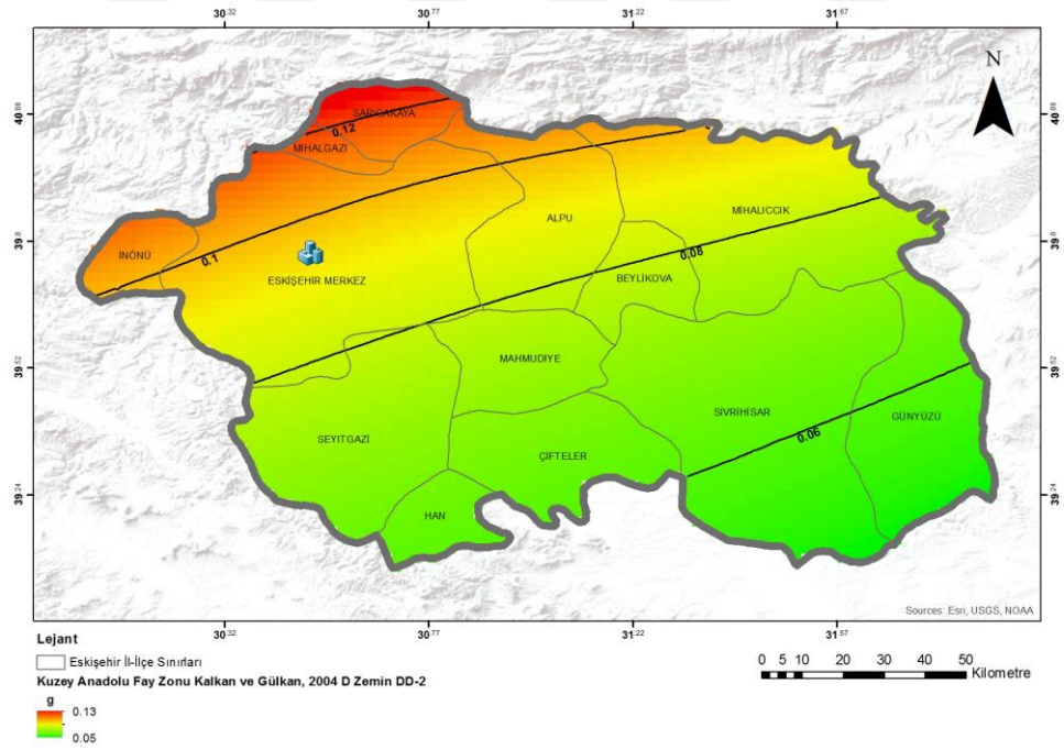
Şekil 6.15. KAFZ Kalkan ve Gülkan, (2004) azalim ilişkisi D zemin sınıfına göre STA haritası (DD-2, 50 yılda %10 aşılma olasılığı ve 475 yıllık tekrarlanma periyodu)
