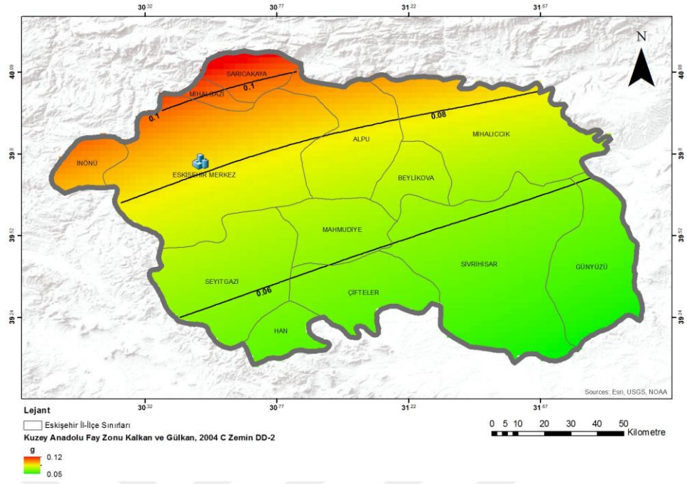
Şekil 6.14. KAFZ Kalkan ve Gülkan, (2004) azalim ilişkisi C zemin sınıfına göre STA haritası (DD-2, 50 yılda %10 aşılma olasılığı ve 475 yıllık tekrarlanma periyodu)
