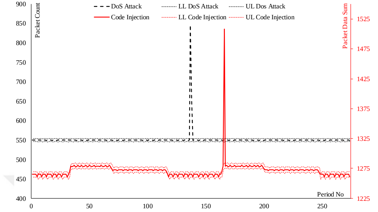
Şekil 5.12. Program 3 - Anomali tespiti
