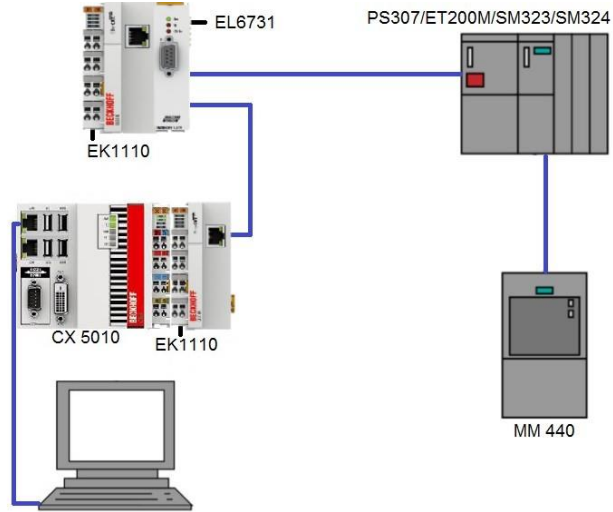
Şekil 6.1 Test ortamı – 1
