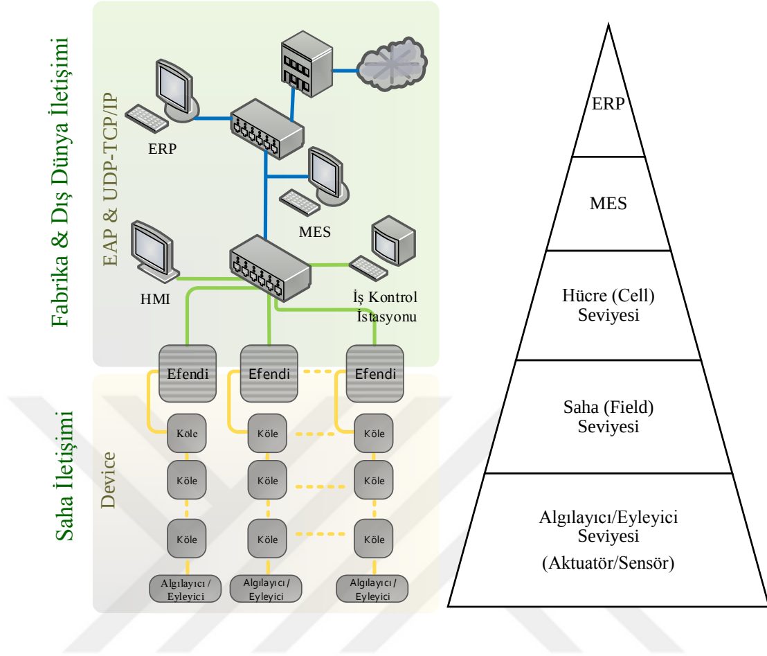
Şekil 2.1. Tüm seviyelerde EtherCAT
