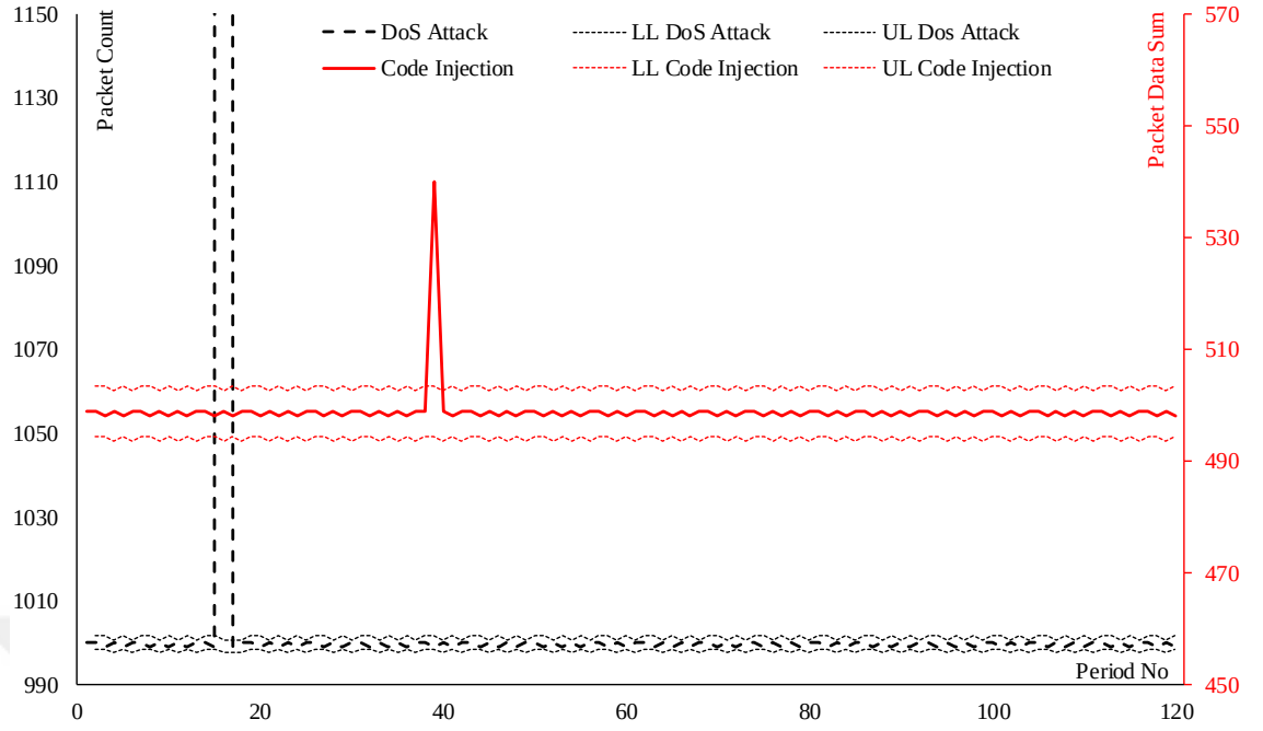
Şekil 5.10. Program 1 - Anomali tespiti
