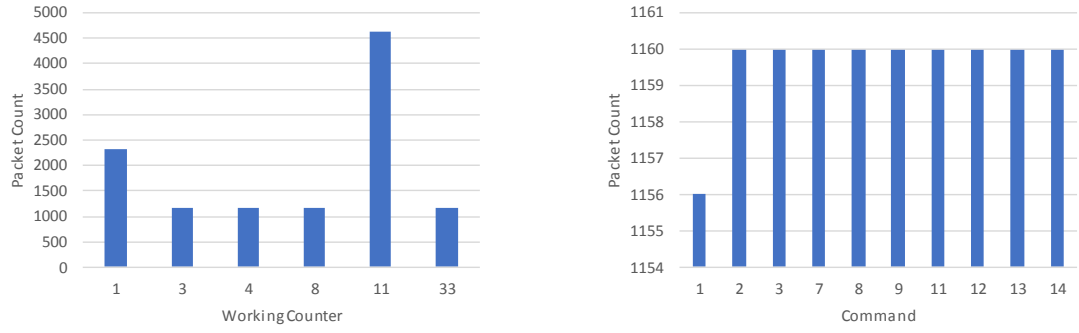
Şekil 3.7. Paket sayısı - WKC grafiği ve Paket sayısı - CMD grafiği
