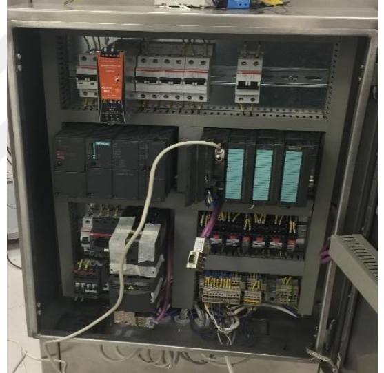
Şekil 6.1 Test ortamı – 1
