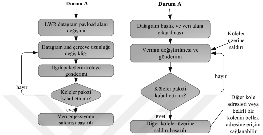
Şekil 3.12. (a) Veri enjeksiyonu saldırı akışı, (b) Köle istasyonlar üzerine saldırı akışı
