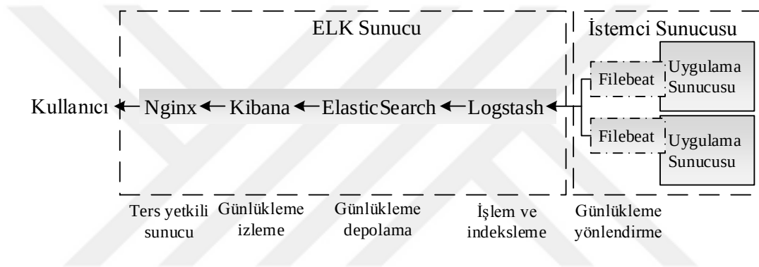
Şekil 4.6. ELK istemci-sunucu entegrasyonu
