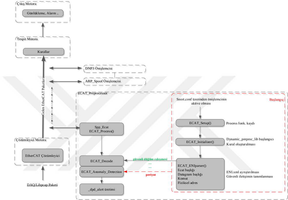
Şekil 5.14. ECAT önışlemcisinde periyodun kullanılması
