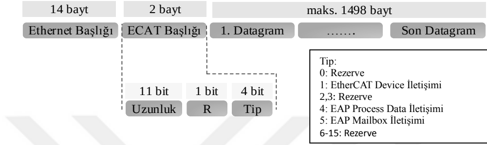
Şekil 2.2. EtherCAT başlığı
