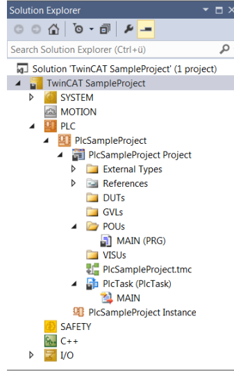
Şekil 4.3. TwinCAT3 proje yapısı
