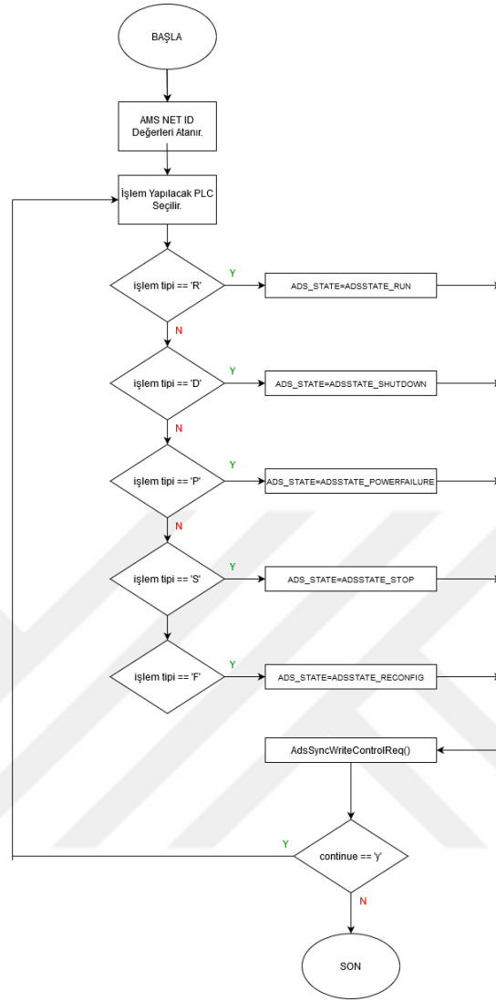
Şekil 3.4. PLC cihaz durum değişimi akış diyagramı
