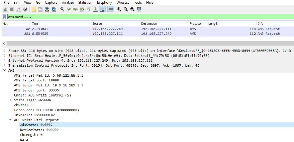
Şekil 3.9. AMS ağ paketi içeriği (CmdId=5)
