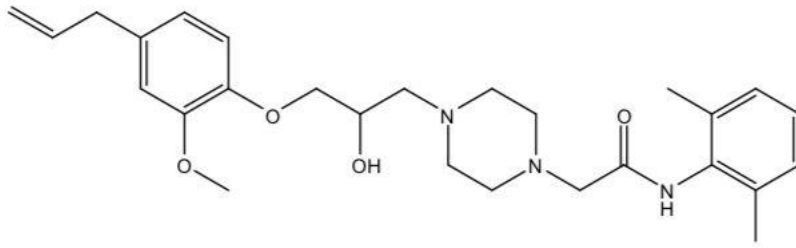
Şekil 5.3. 2-(4-(3-(4-alil-2-metoksifenoksi)-2-hidroksi)propil)piperazin-1-il)-N-(2,6-dimetilfenil)asetamid sentezi
