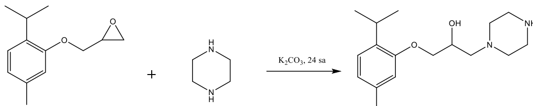
Şekil 3.6. Timol eklentili oksiranın piperazinle açılma reaksiyonu
