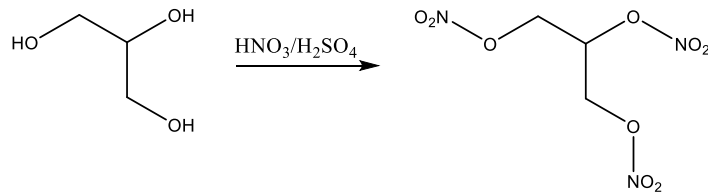
řekil 2.2. Nitrogliserin sentez reaksiyonu [8]
