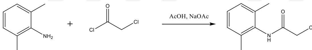
Şekil 3.7. 2-kloro-N-(2,6-dimetilfenil) asetamit eldesi
