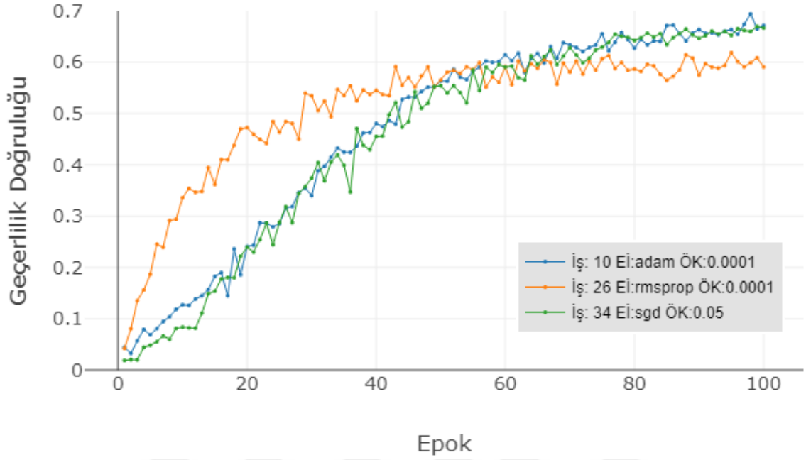
Şekil 3.24. Her bir eniyileme fonksiyonunun ulaştığı en yüksek başarıım
