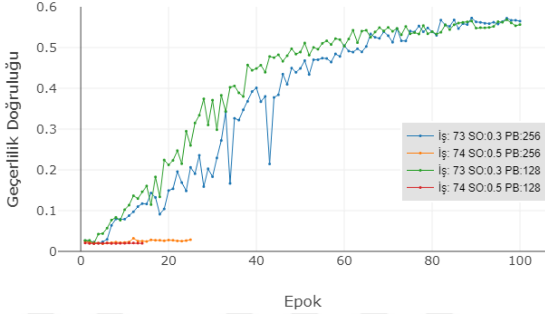
Şekil 3.19. 74. eğitimin seyreltme oranı hariç tüm parametreleri aynı olan eğitimle kıyaslanması
