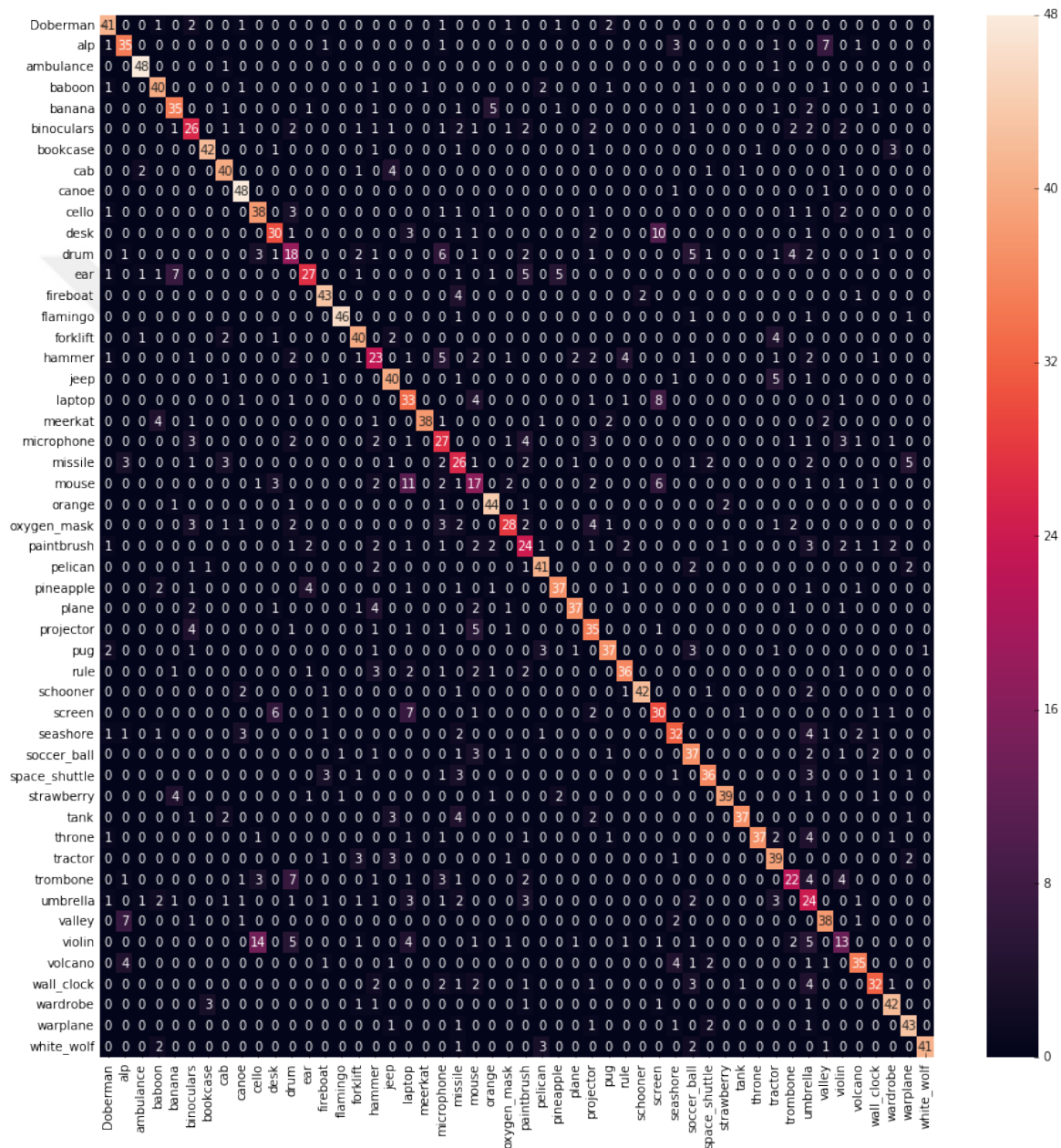
Şekil 4.2 Hata matrisi
