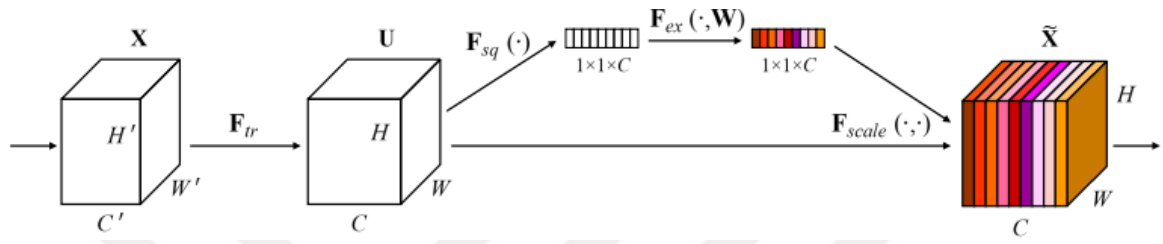
Şekil 2.37. Squeeze-and-Excitation blokları [56]
