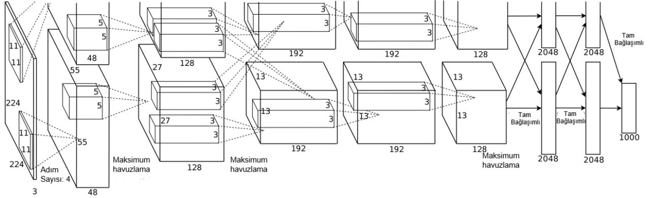
Şekil 2.30. AlexNet ağı [48]
