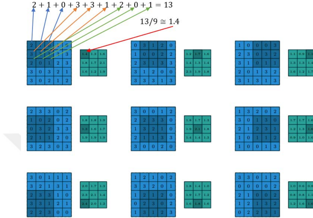
Şekil 2.21. Ortalama havuzlama örneği
