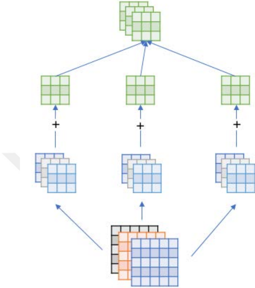
Şekil 2.19. İki adet girdiye üç farklı filtre uygulanması örneği
