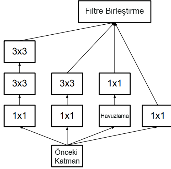
Şekil 2.35. Inception V3 ağı
