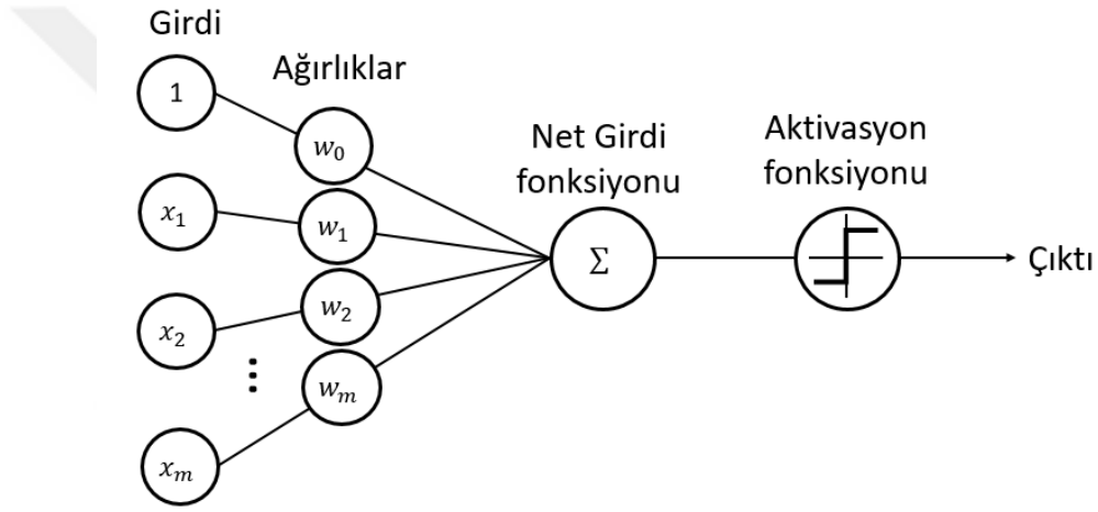
Şekil 2.1. Rosenblatt'a göre perseptron modeli
