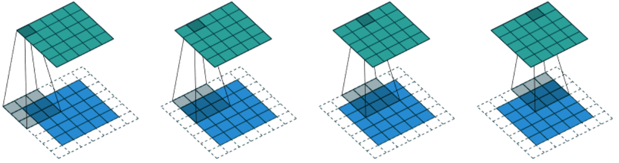
Şekil 2.24. Yarım (Aynı) dolgulu evrişim örneği [43]
