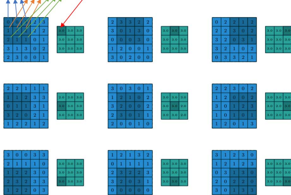
Şekil 2.20. Maksimum havuzlama örneği
