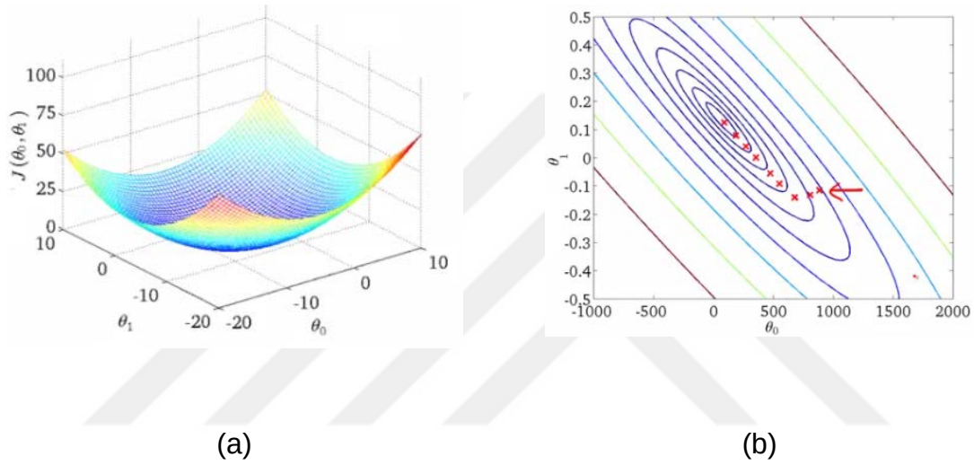
Şekil 2.5. Konveks fonksiyonun yüzey grafiği [11]
