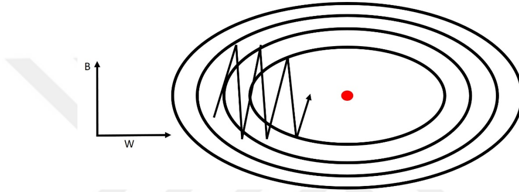
Şekil 2.12. RMSprop salınımı
