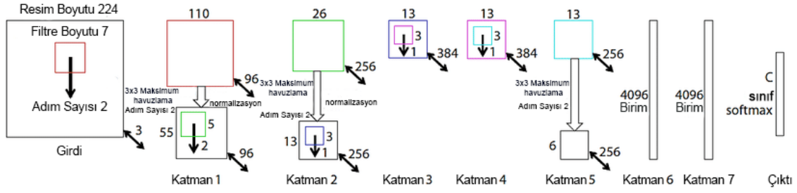
Şekil 2.31. ZFNet ağı
