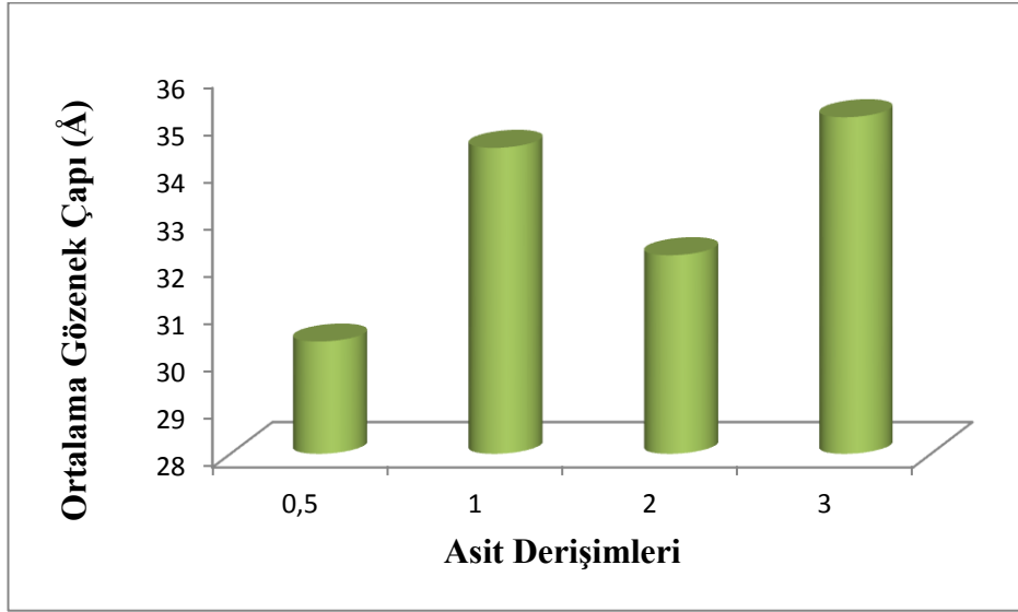
Şekil 7.20. Silis kumundan sentezlenen silika aerojellerde kullanılan asit derişiminin artmasıyla ortalama gözenek çap deęiřimi
