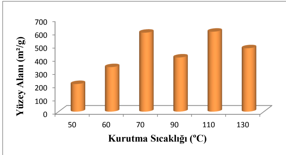
Şekil 7.3. Silis kumundan sentezlenen silika arojelde kurutma sıcaklığının artmasıyla yüzey alanının değişimi
