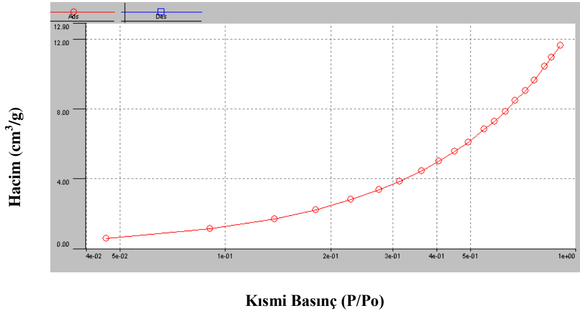
Şekil E1.7. Kurutma sıcaklığı 60 °C olan feldspattan sentezlenen F2 numunesinin izoterm eğrisi
