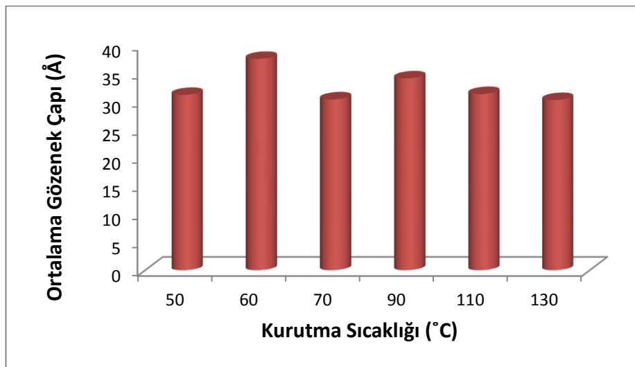
Şekil 7.4. Silis kumundan sentezlenen silika arojelde kurutma sıcaklığının artmasıyla ortalama gözenek çap değişimi
