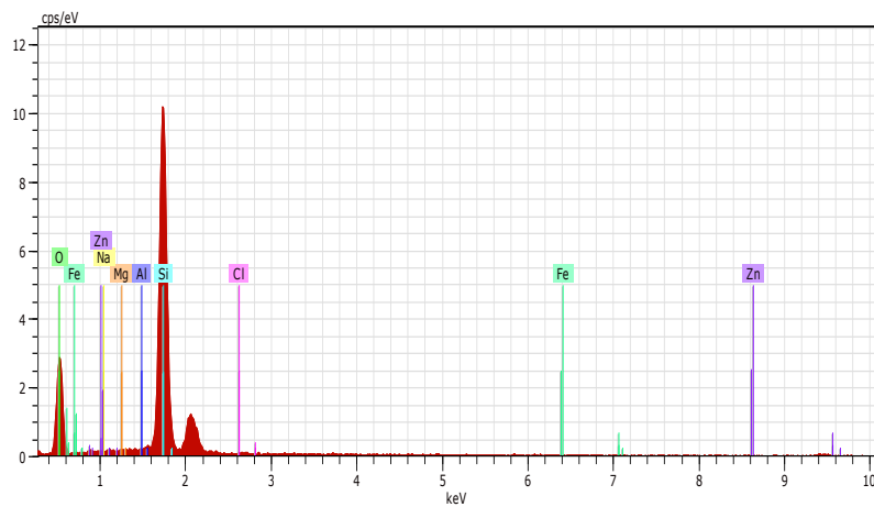
Şekil E2.7. Ürel ortamda sentezlenen MSÜ4 numunesinin EDS sonucu
