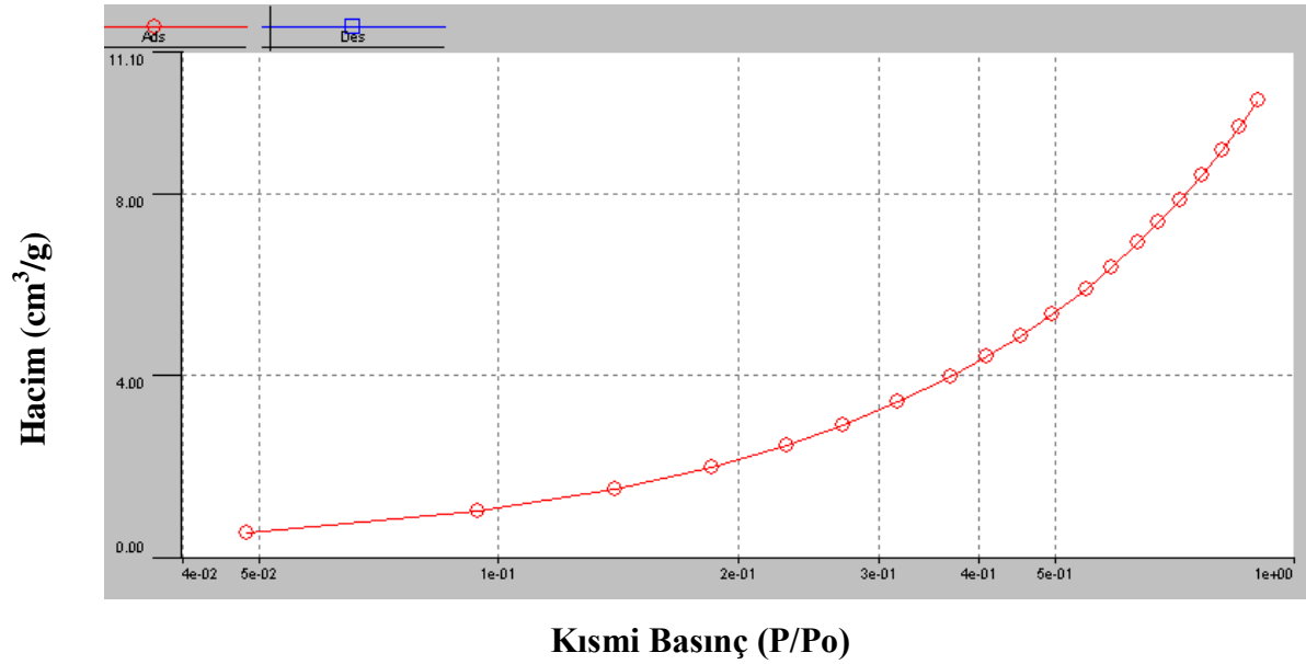
Şekil E1.32. Üresiz ortamda 0,8 ml HNO 3 kullanılarak sentezlenen MS4 numunesinin izoterm eğrisi
