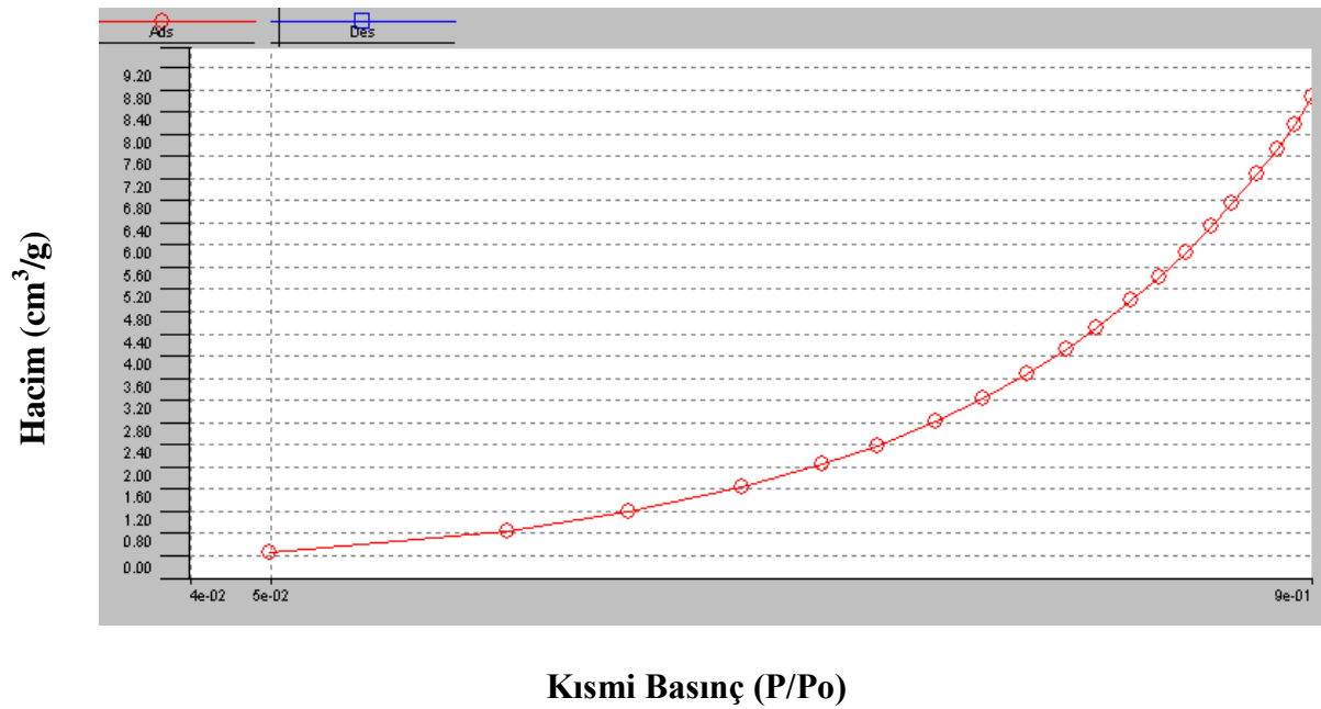
Şekil E1.9. Kurutma sıcaklığı 90 °C olan feldspattan sentezlenen F4 numunesinin izoterm eğrisi
