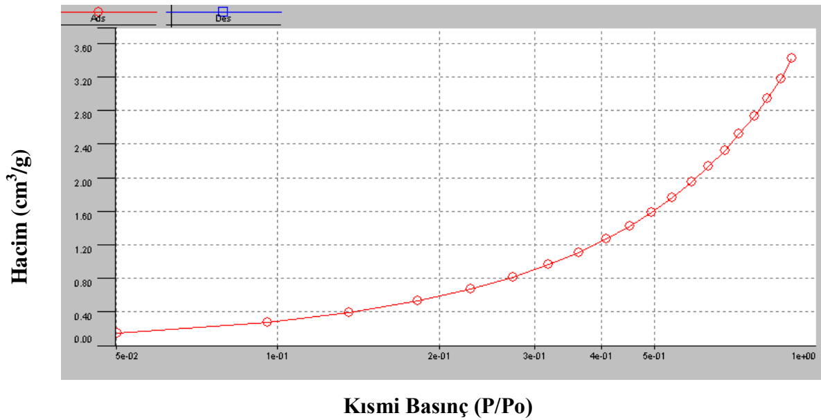
Şekil E1.32. Üresiz ortamda 1,2 ml \text{HNO}_3 kullanılarak sentezlenen MS6 numunesinin izoterm eğrisi
