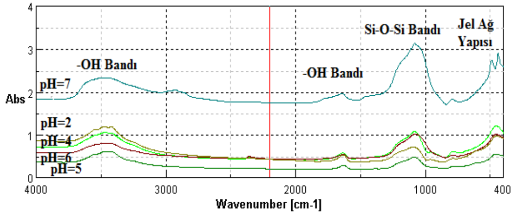
Şekil 7.9. Silis kumundan pH değiştirilerek elde edilen silika aerojellerinin FTIR spektrumları
