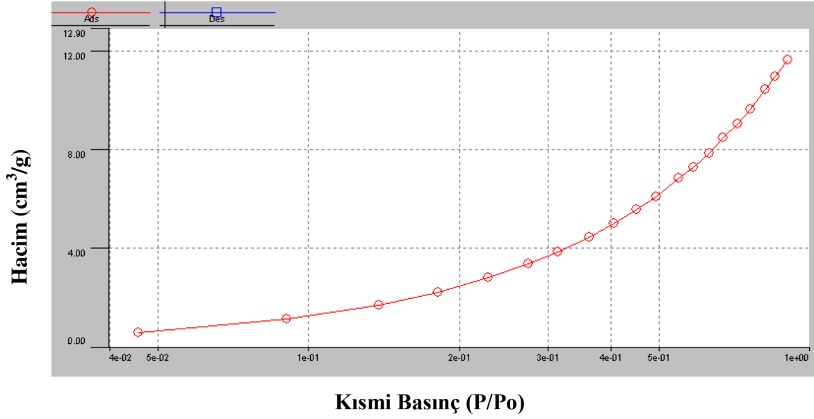
Şekil E1.32. Üresiz ortamda 1,0 ml \text{HNO}_3 kullanılarak sentezlenen MS5 numunesinin izoterm eğrisi
