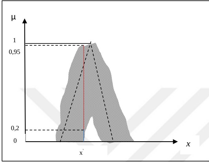
Şekil 3.4. Aralıklı bulanık küme
