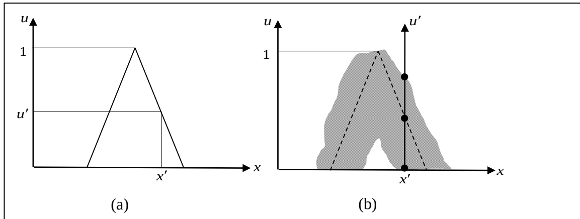
Şekil 3.5. (a) Üçgensel Tip-1 üyelik fonksiyonu (b) Bulanıklaştırılmış Üçgensel Tip-1 üyelik fonksiyonu
