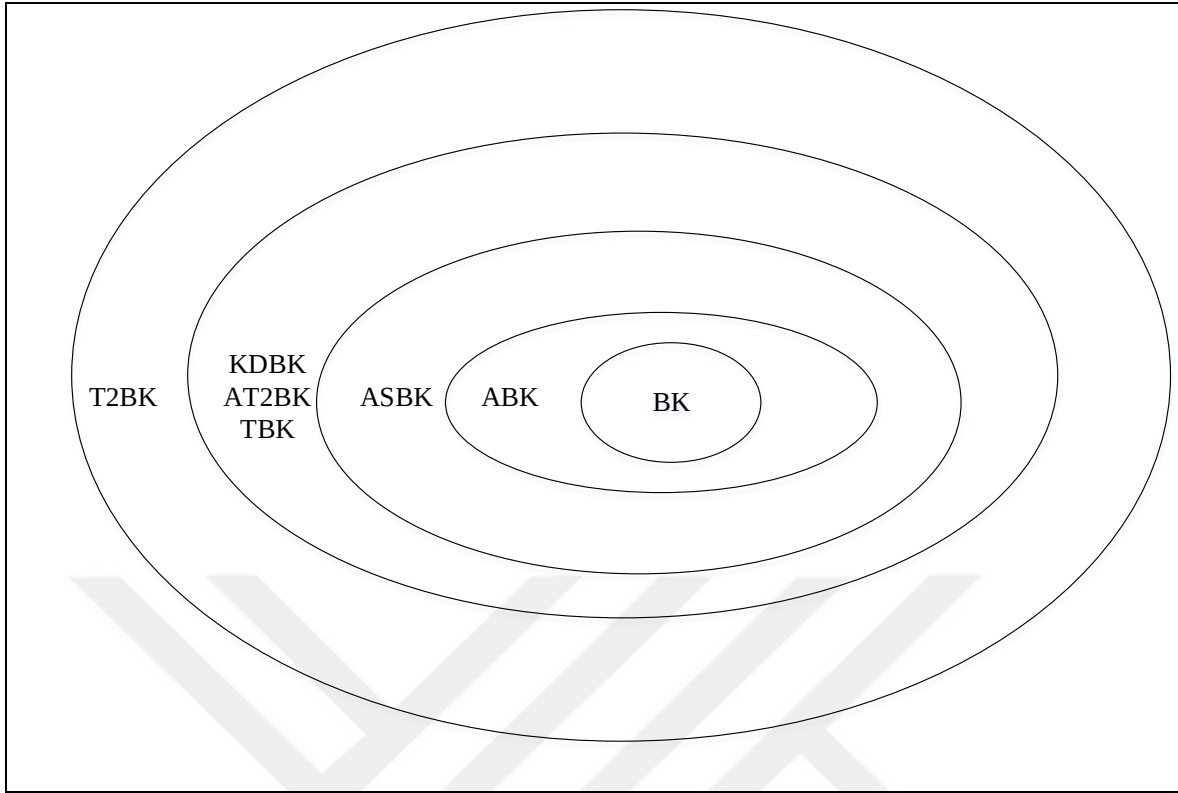
Şekil 3.14. Bulanık küme tipleri arasındaki bağlantı
