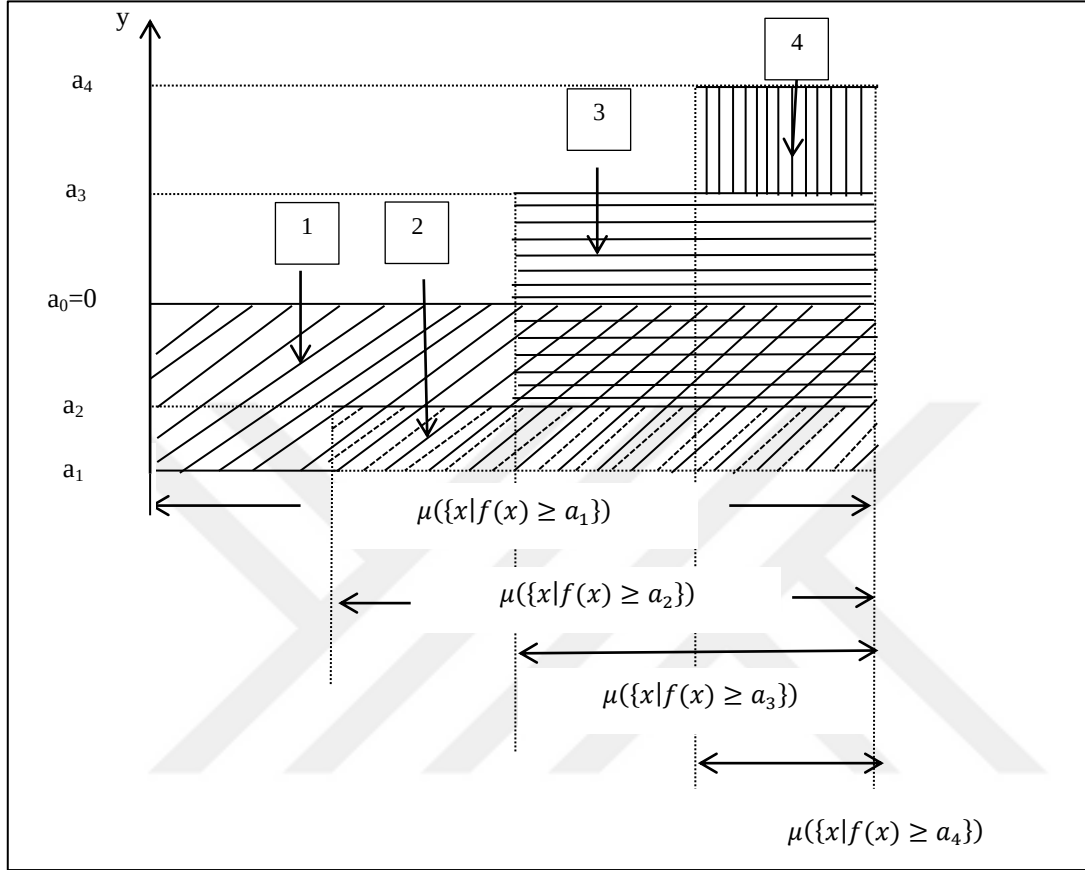
Şekil 4.4. f fonksiyonunun integrali
