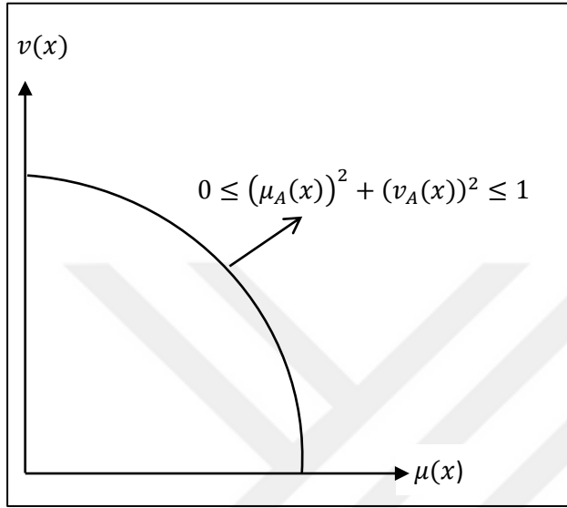
Şekil 3.9. Pisagor bulanık küme
