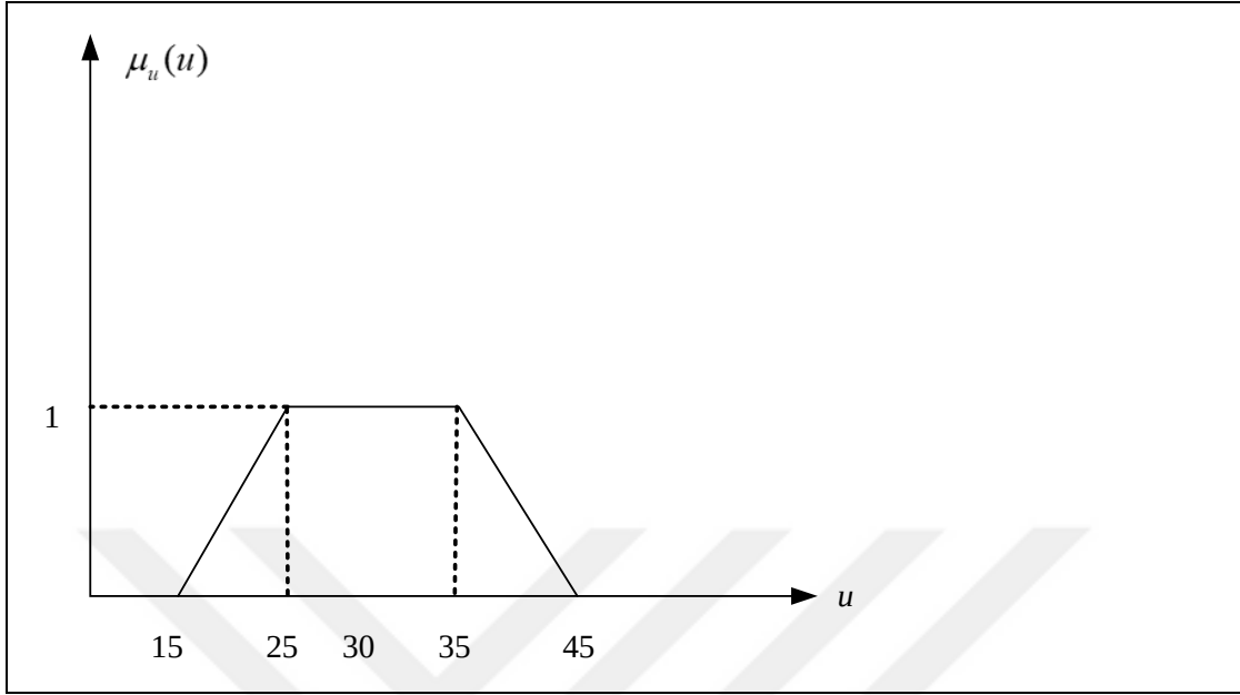
Şekil 2.6. Gen\u00e7 bulanık kümesi
