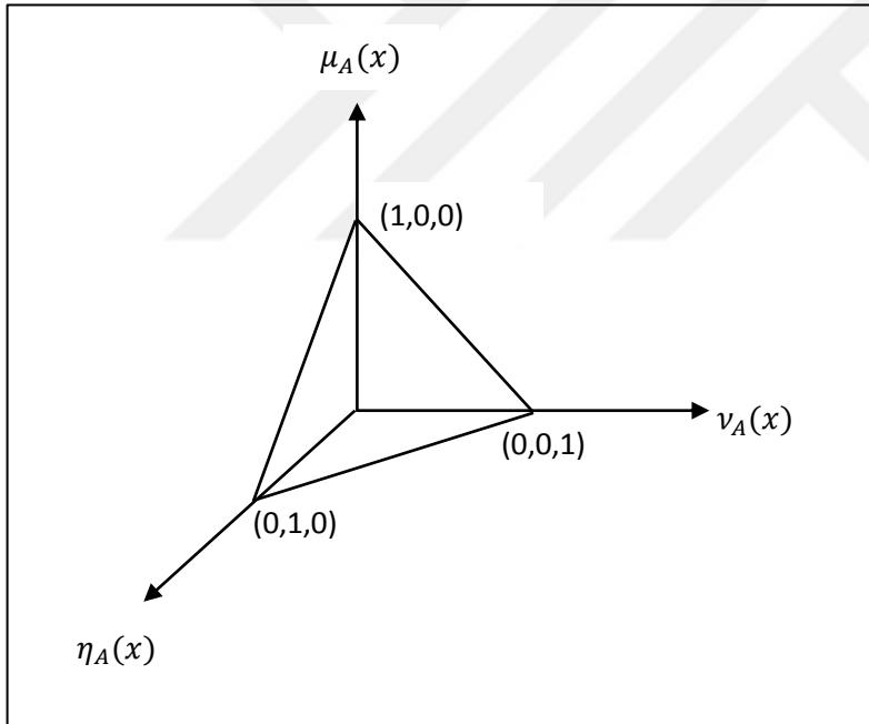
Şekil 3.10. Görüntü bulanık küme
