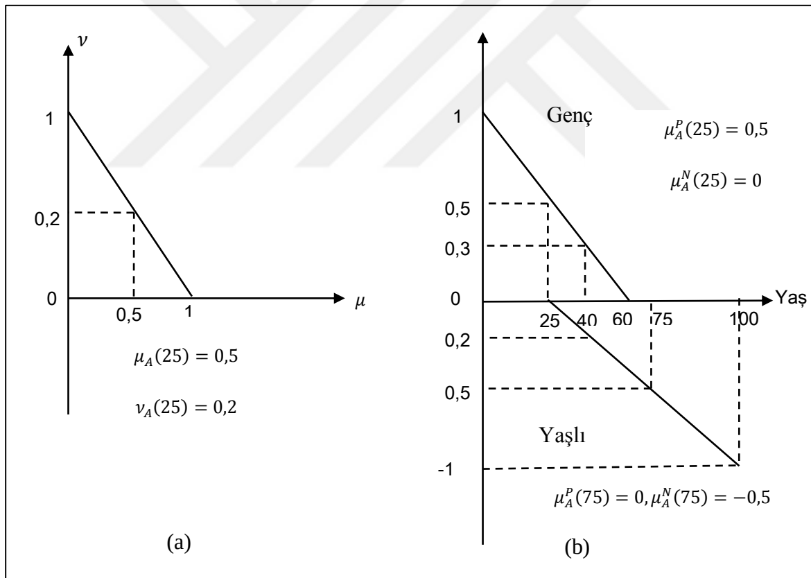
Şekil 3.11 (a) 25 değerinin SBK'de gösterimi (b) Gençiki kutuplu bulanık kümesi
