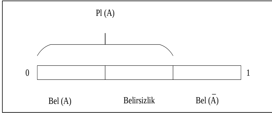
Şekil 2.3. İnanç ve mümkünlik fonksiyonları arasındaki ilişki
