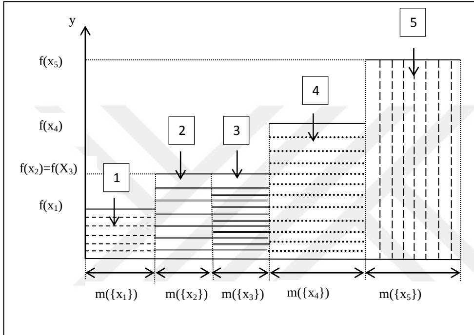
Şekil 4.1. f fonksiyonunun integrali
