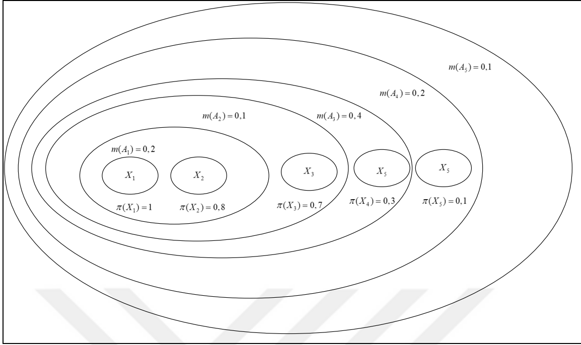
Şekil 2.5. Olabilirlik ölçüsünün iç içe geçmiş odak elemanları
