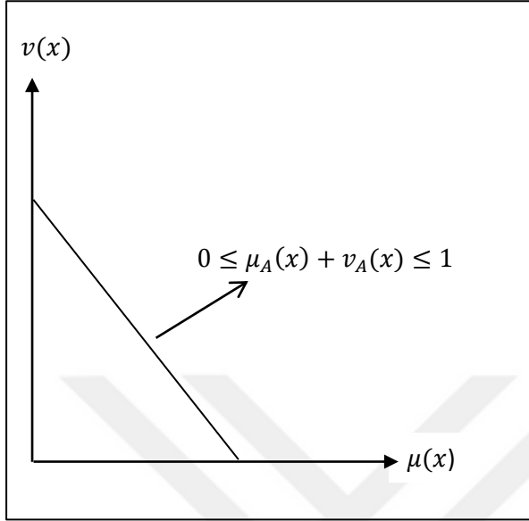
Şekil 3.8. Sezgisel bulanık küme
