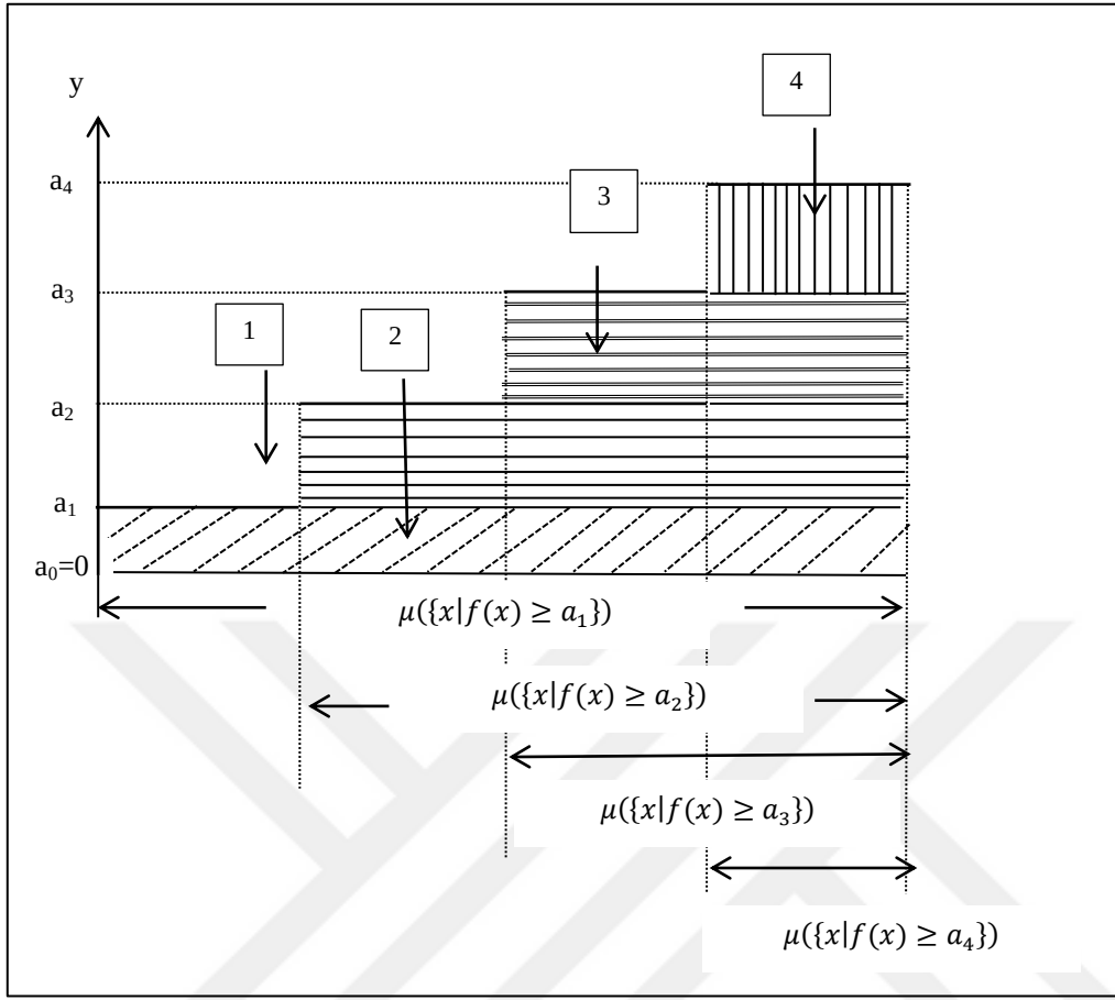
Şekil 4.3. f fonksiyonunun integrali
