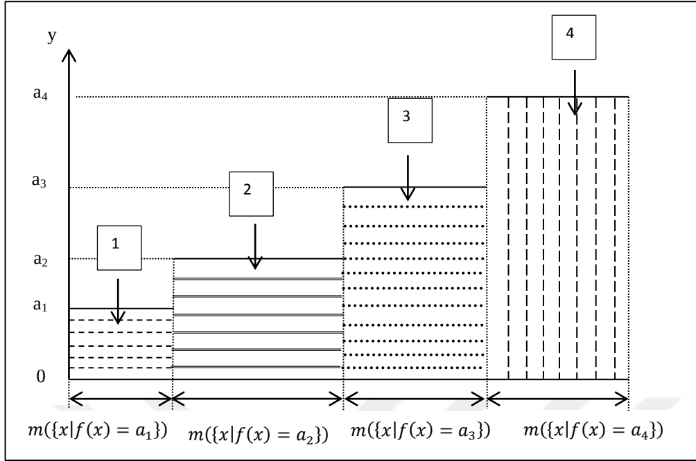
Şekil 4.2. f fonksiyonunun integrali
