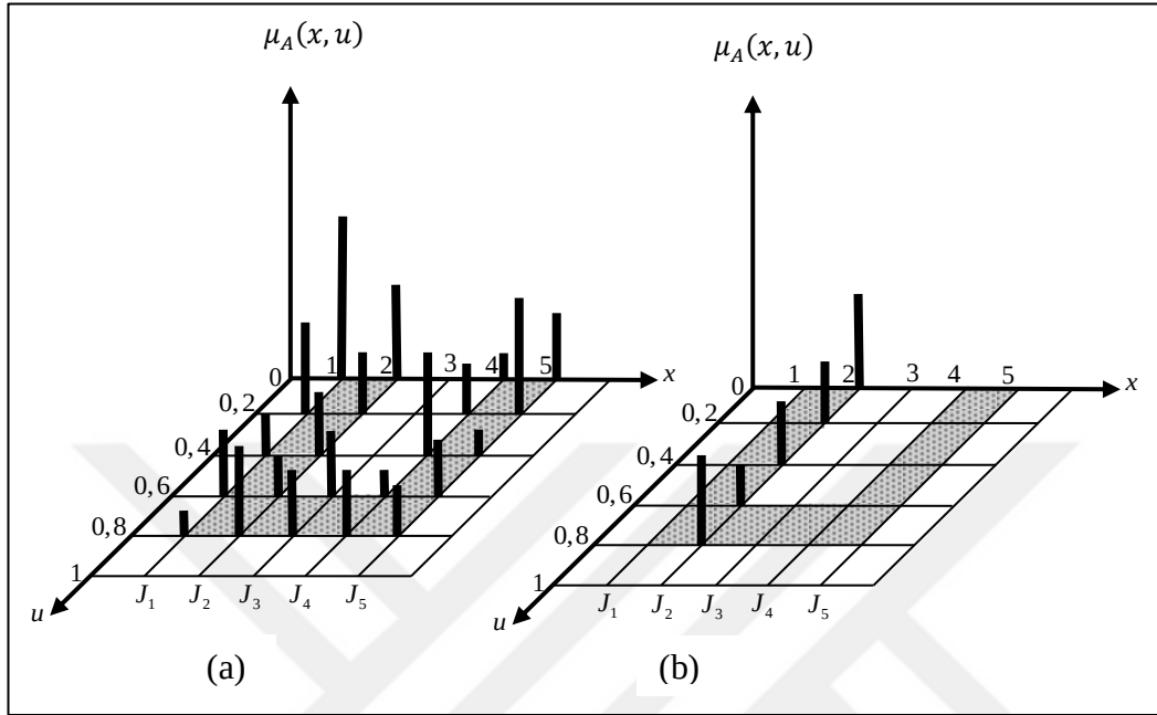
Şekil 3.6. (a) 3 boyutlu tip-2 üyelik fonksiyonu (b) x = 2 noktasında tip-2 üyelik fonksiyonunun dikey kesit gösterimi
