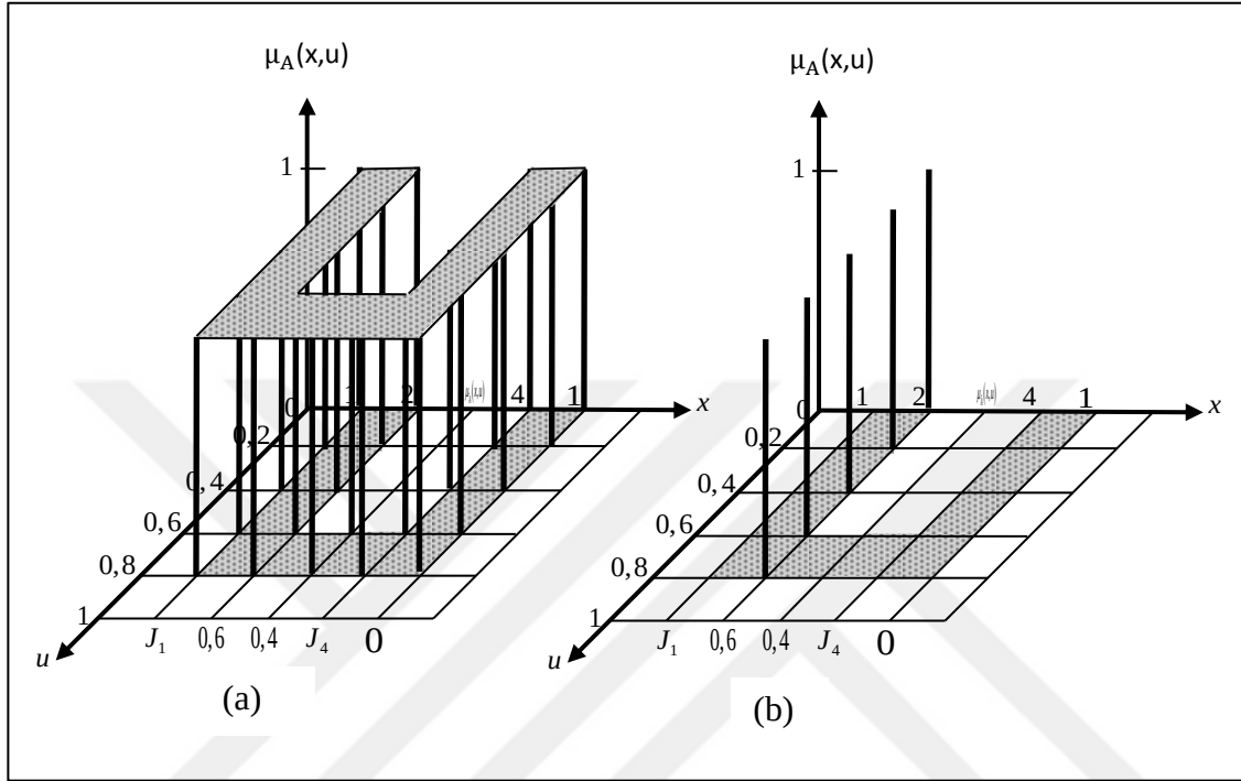
Şekil 3.7. (a) 3 boyutlu aralıklı tip-2 üyelik fonksiyonu (b) x=2 noktasında aralıklı tip-2 üyelik fonksiyonunun dikey kesit gösterimi
