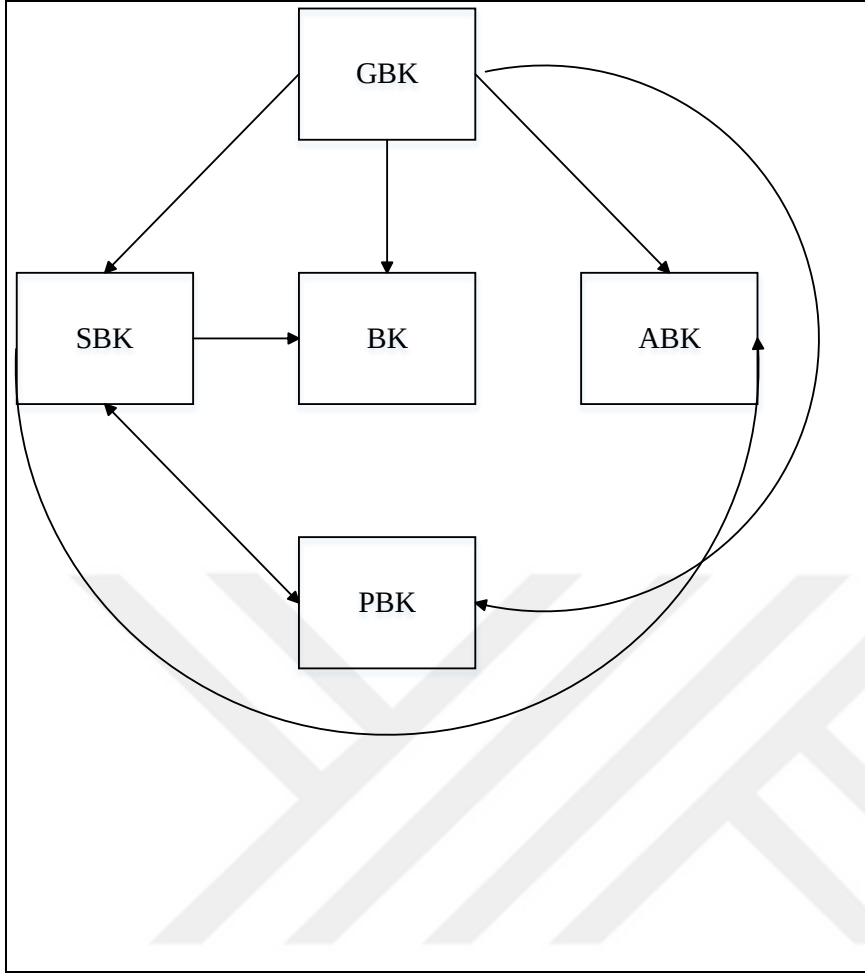
Şekil 3.15. Farklı Kümeler Arasındaki İlişki
