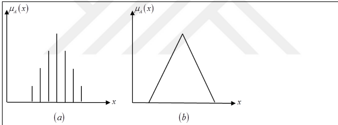
Şekil 3.3. Farklı tipte bulanık kümeler: (a) Kesikli bulanık küme (b) Sürekli bulanık küme
