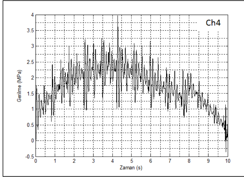
Şekil 5.29 “Double T” farklı birleştirilmiş CTP taşıyıcı kiriş m_L=200\text{kg} için, 4. gerinim ölçerden alınan ölçüm değerlerinin nümerik gerilme-zaman grafiği
