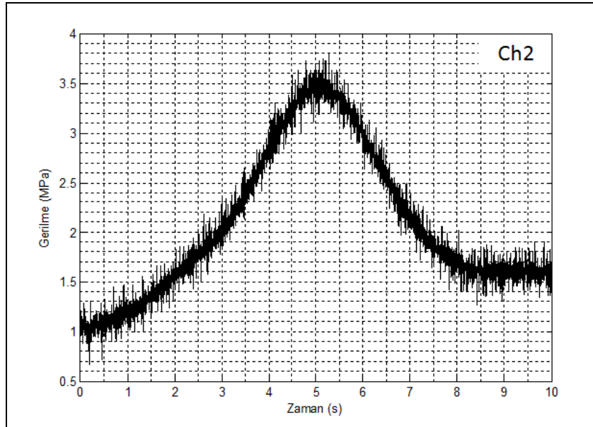
Şekil 5.47 “Double T” farklı birleştirilmiş CTP taşıyıcı kiriş m_L=300\text{kg} için, 2. gerinim ölçerden alınan ölçüm değerlerinin deneysel gerilme-zaman grafiği
