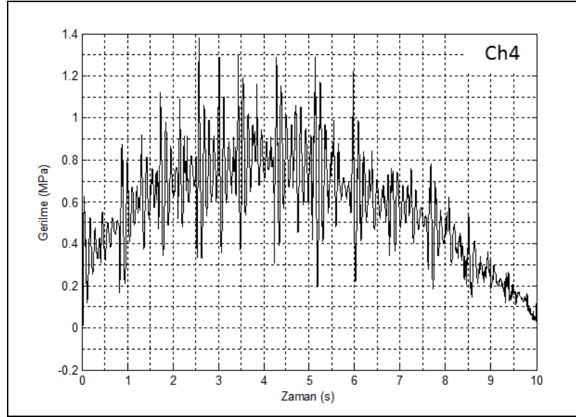
Şekil 5.25 “Double T” farklı birleştirilmiş CTP taşıyıcı kiriş m_L=100\text{kg} için, 4. gerilimölçerden alınan ölçüm değerlerinin nümerik gerilme-zaman grafiği
