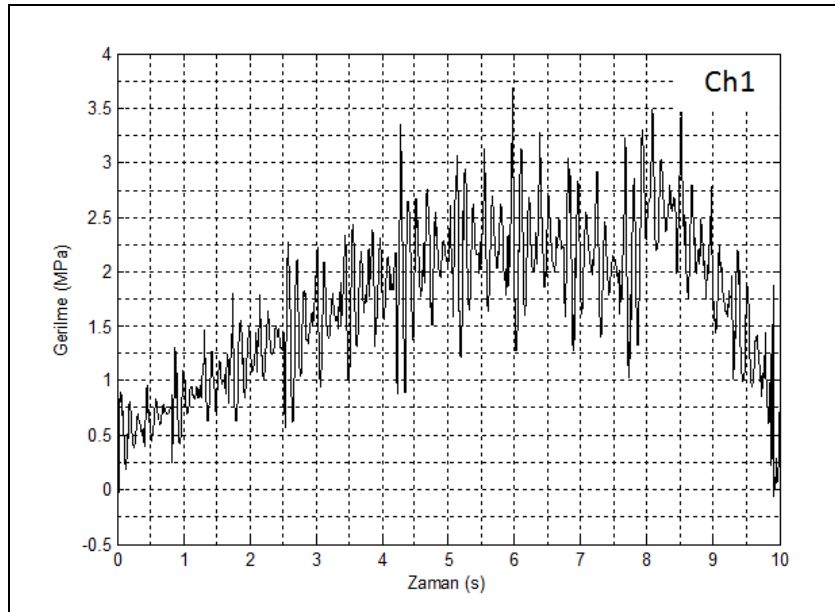
Şekil 5.26 “Double T” farklı birleştirilmiş CTP taşıyıcı kiriş m_L=200\text{kg} için 1. gerilimölçerden alınan ölçüm değerlerinin nümerik gerilme-zaman grafiği
