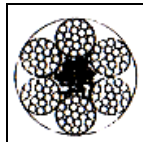
řekil 4.6 DIN3060’a göre 6x19 Std.elik halat kesiti
