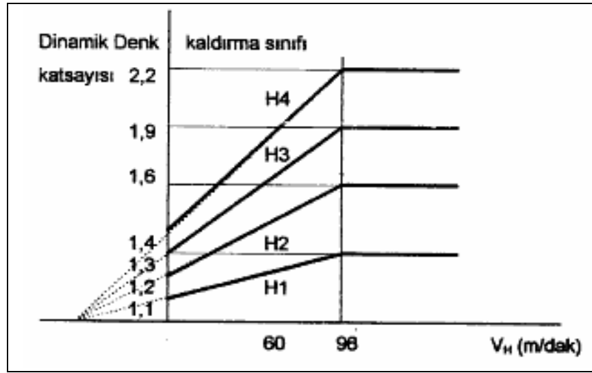
Şekil 3.8 Kaldırma yk katsayıları [DIN 15018 kısım1]
