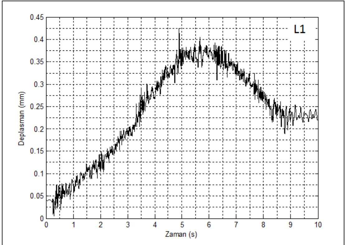
Şekil 5.50 “Double T” farklı birleştirilmiş CTP taşıyıcı kiriş m_L=0\text{kg} için 1 numaralı lazer ölçüm cihazından alınan ölçüm değerleri ile oluşturulan deneyisel deplasman-zaman grafiği
