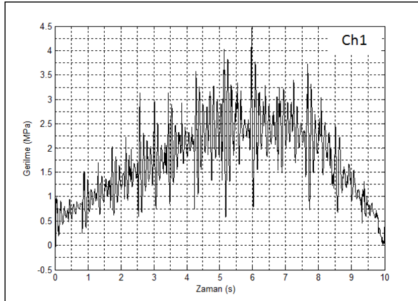
Şekil 5.22 “Double T” farklı birleştirilmiş CTP taşıyıcı kiriş m_L=100\text{kg} için 1. gerinim ölçerden alınan ölçüm değerlerinin nümerik gerilme.-zaman grafiği
