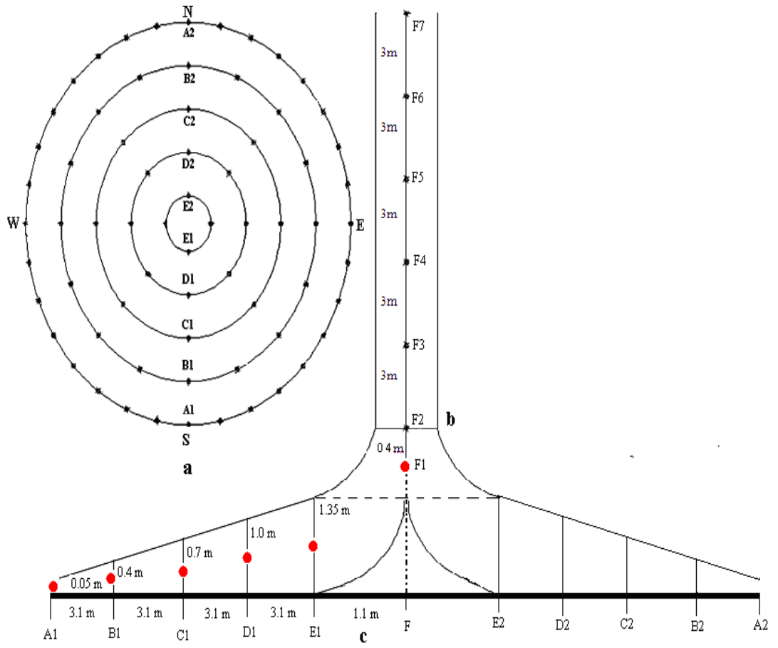
Şekil 3.34 Güneş bacası sisteminde hava hızı ve hava sıcaklıklarının ölçüm noktaları, a: zeminin (asfalt) ölçüm noktaları, b: bacanın merkezinden ölçülen noktalar ve yükseklikleri, c: kolektörün altında ölçüm noktaları ve yükseklikleri [38].
