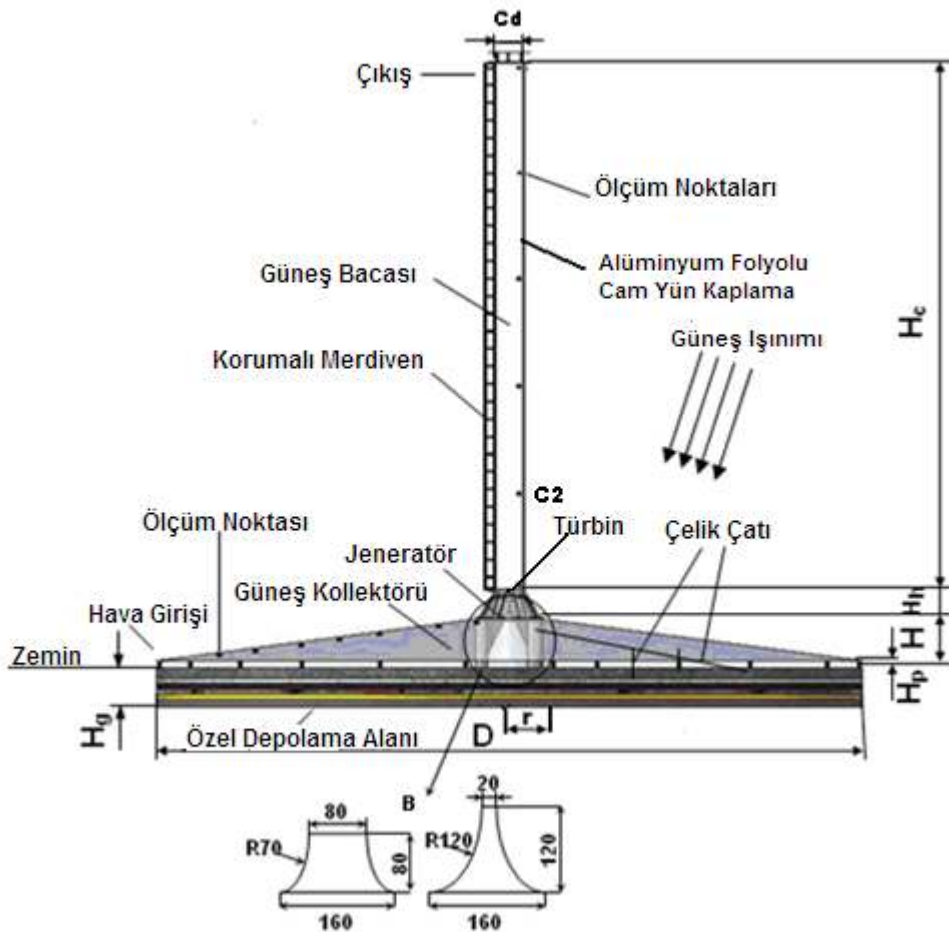
Şekil 3.8 Güneş bacası sisteminin şematik diyagramı [35]
