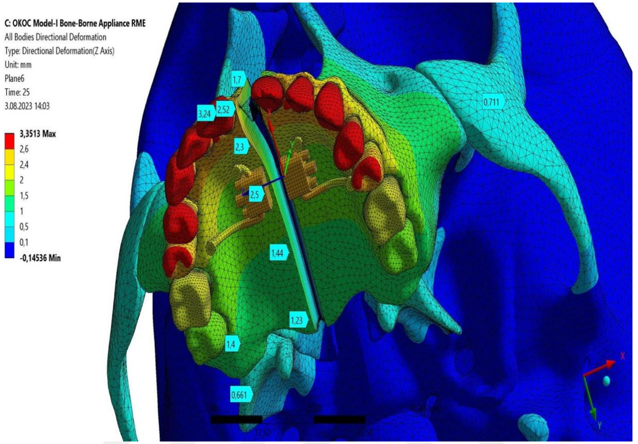
Şekil 17: Model I, z ekseninde (transversal yönde) yer değıştirme (mm) miktarı (Okluzal)
