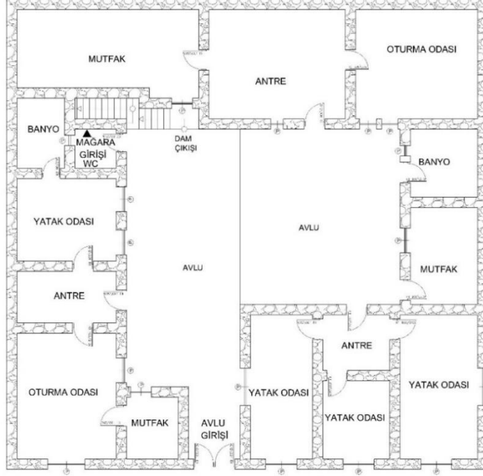
ZEMİN KAT KROKİSİ
