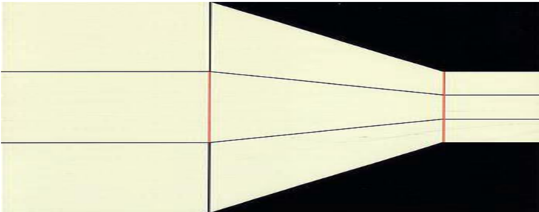
Şekil 3.13. Algıda derinlik ve mesafe ilişkisi, (İleriye 2007: s. 75)
