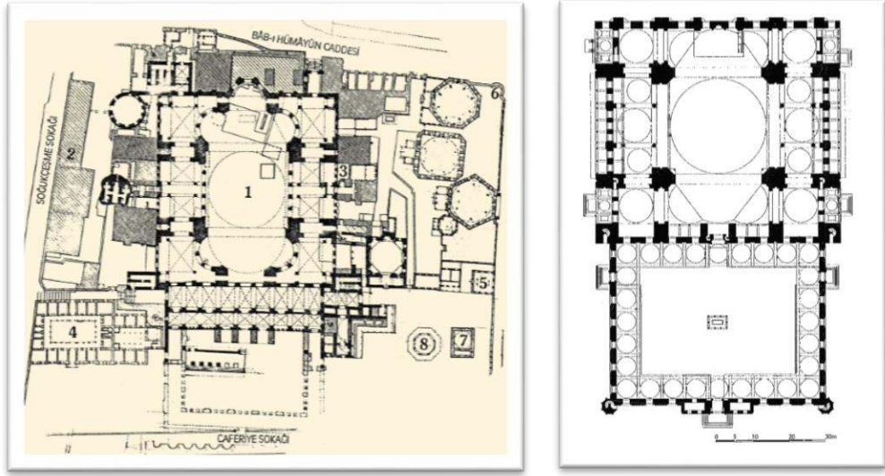
Şekil 3.11. Ayasofya Camii, İstanbul 532-537 ve Süleymaniye Camii, İstanbul 1551-1558 Planları
