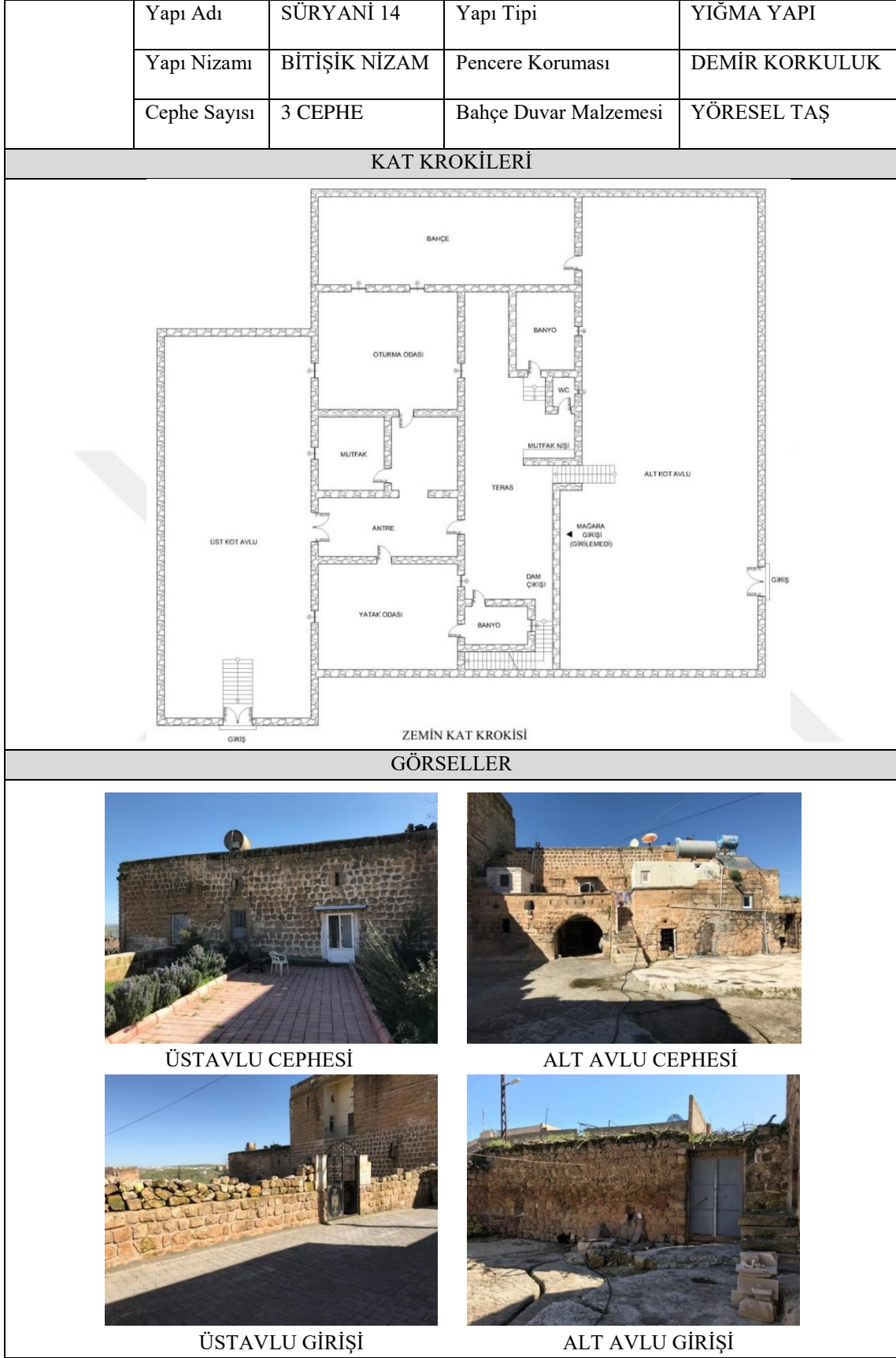
Şekil 4.34. 14 nolu Süryani evi
