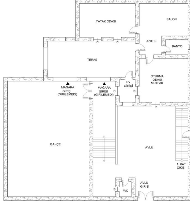
ZEMİN KAT KROKİSİ
