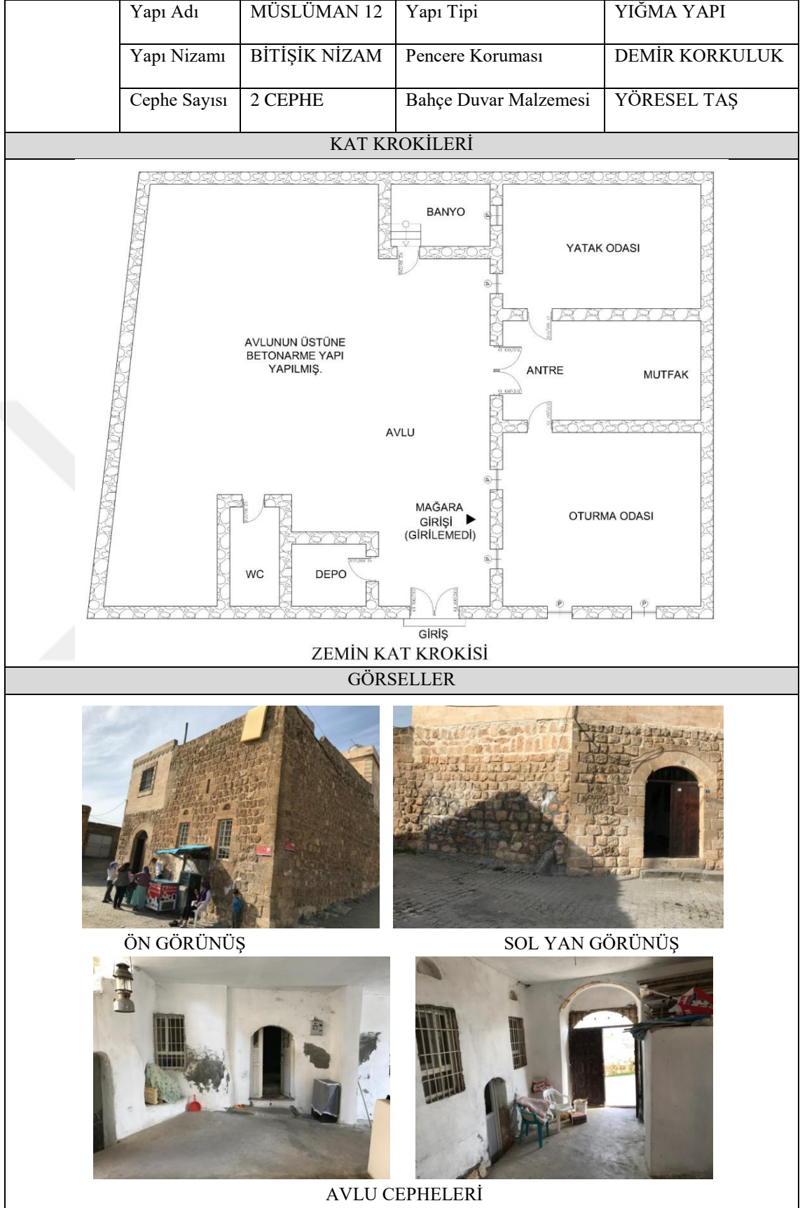
Şekil 4.12. 12 nolu Müslüman evi
