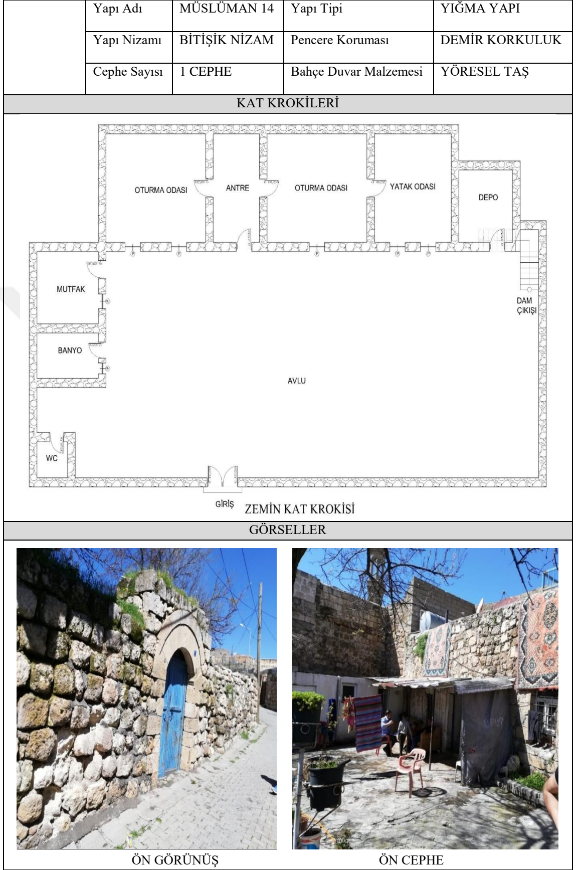
Şekil 4.14. 14 nolu Müslüman evi
