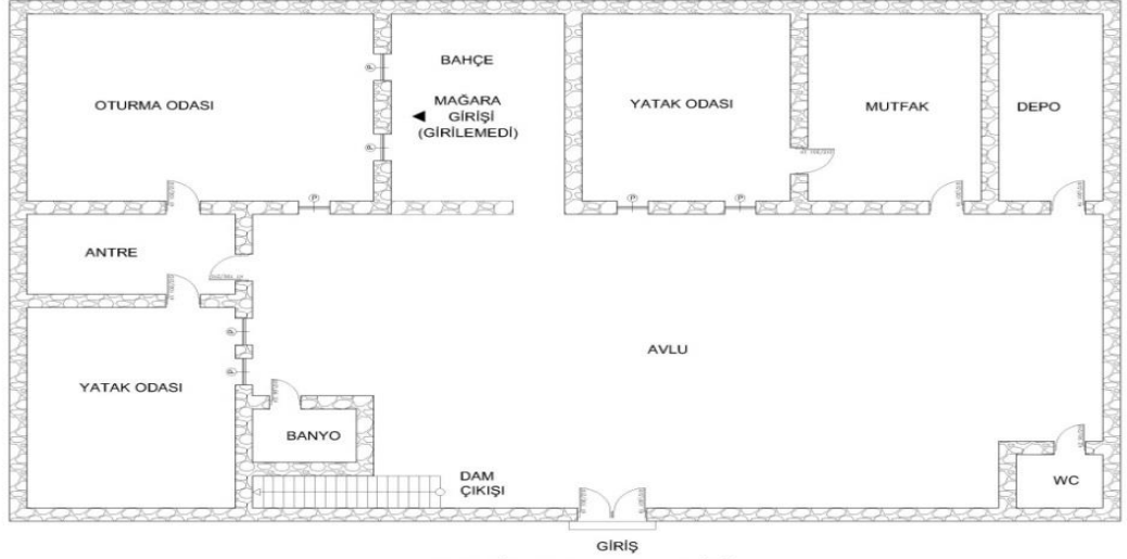
ZEMİN KAT KROKİSİ
