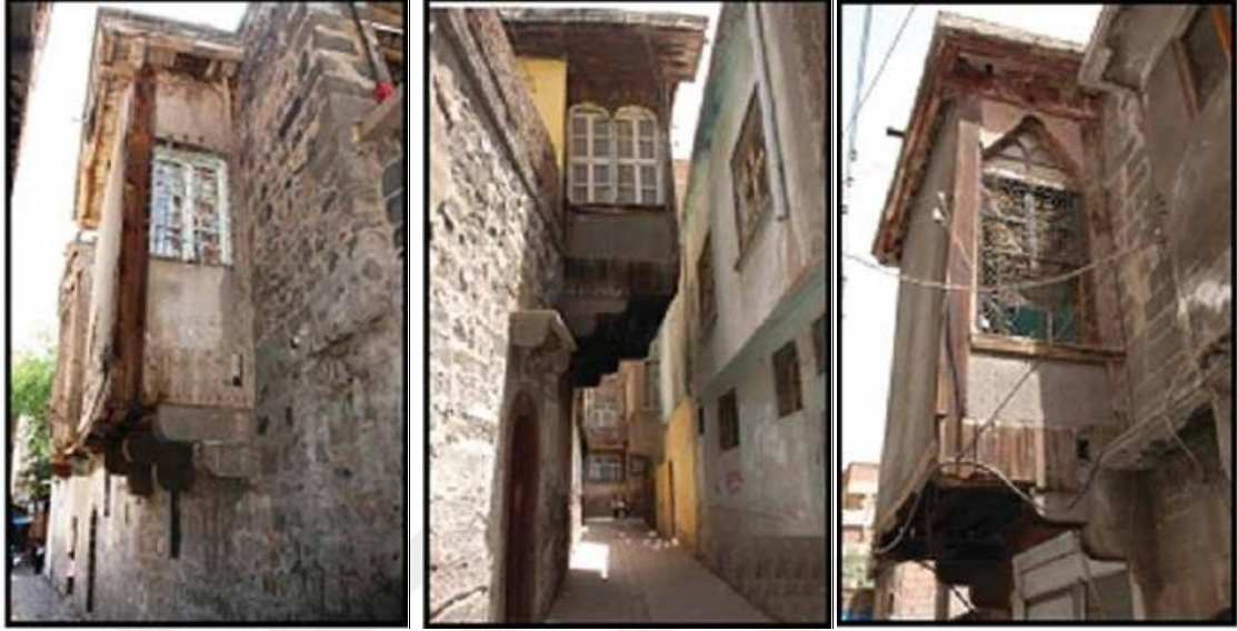
řekil 3.18. Diyarbakır evlerinde ahşap kafesli cumba pencereleri
