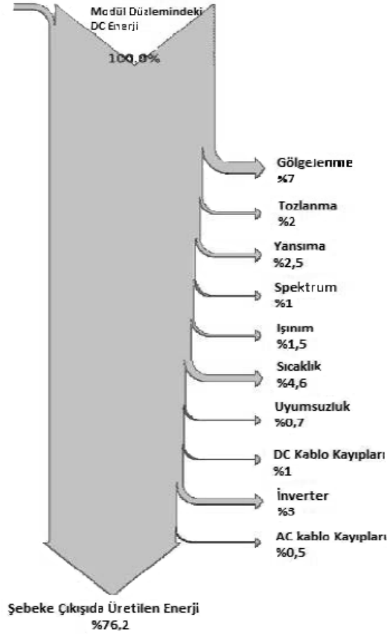
Şekil 2. 13. FV sistemlerde kayıplar (Deniz, 2013)
