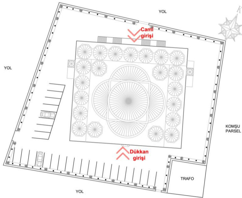
Şekil 3.51 Güzeloba Cami vaziyet planı
