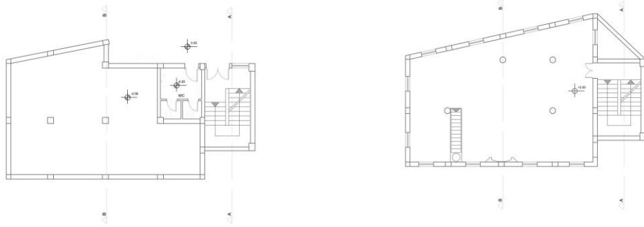
Şekil 3.58. İmam-ı Azam Cami zemin kat planı, 2.50 kot planı
