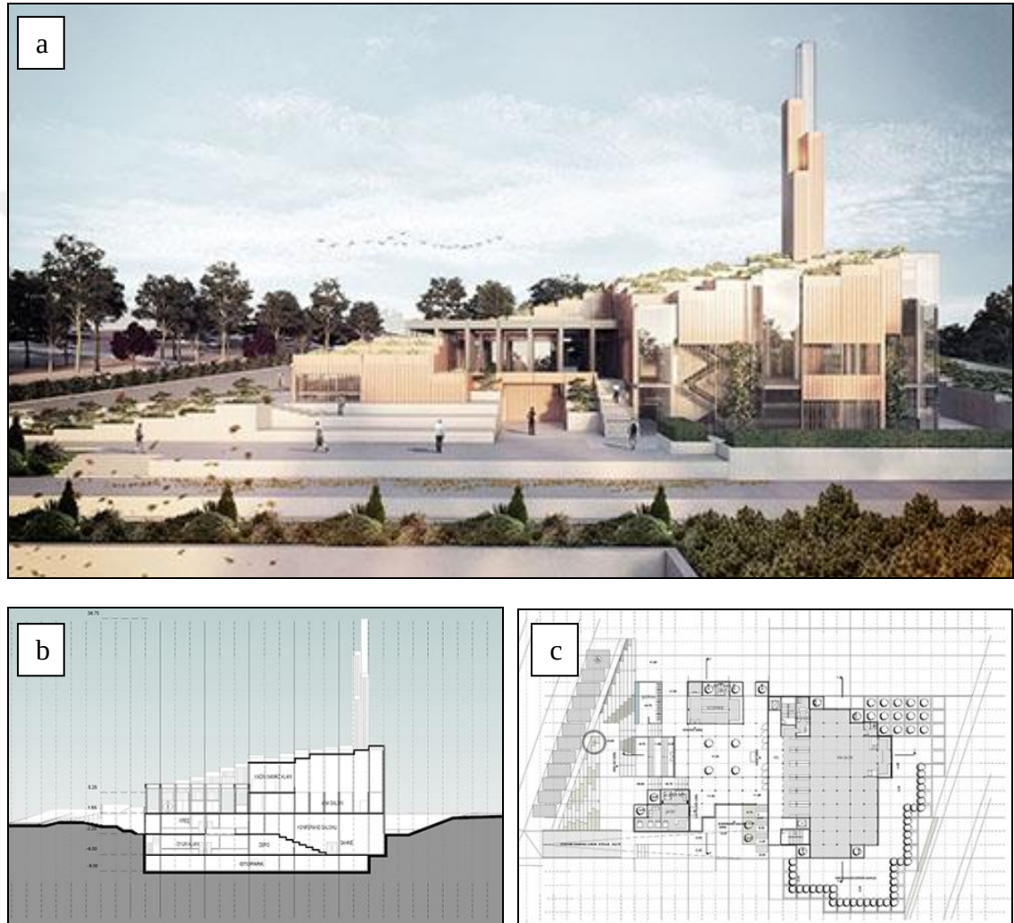
Şekil 2.13. a) İki Pınar cami modeli; b) A-A kesiti; c) Zemin kat planı (rggA 2019)
