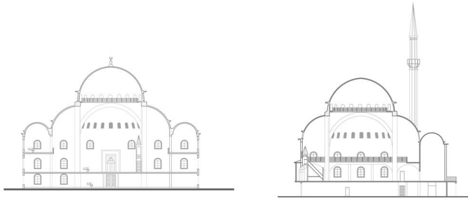
Şekil 3.53. Güzeloba Cami A-A kesiti, B-B kesiti
