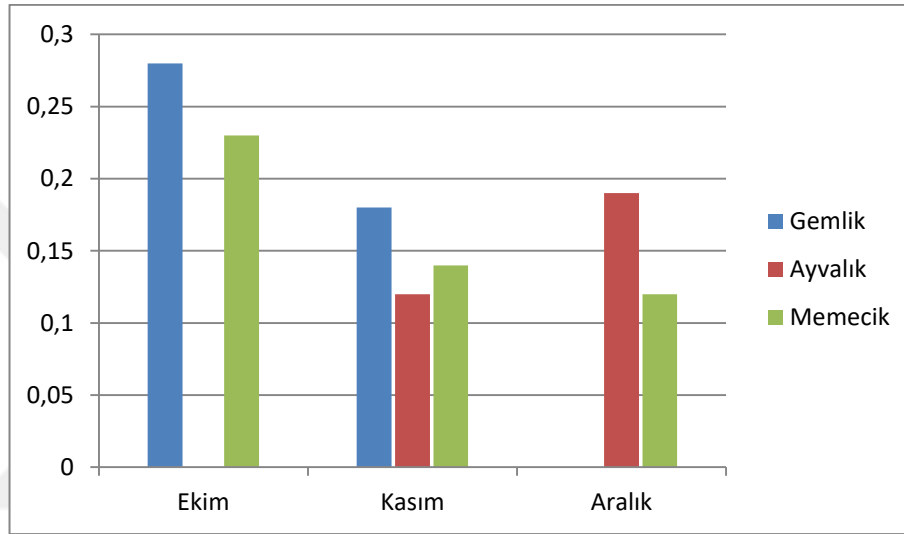
Şekil 4.13.8. Gemlik, Ayvalık ve Memecik zeytinyağlarının ferulik asit içeriklerinin olgunlaşma dönemiyle değişimi (mg/100g)
