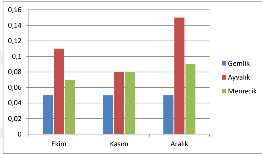
Şekil 4.10.1. Gemlik, Ayvalık ve Memecik zeytinyağlarının trilinolein içeriklerinin olgunlaşma dönemiyle değişimi (%)
