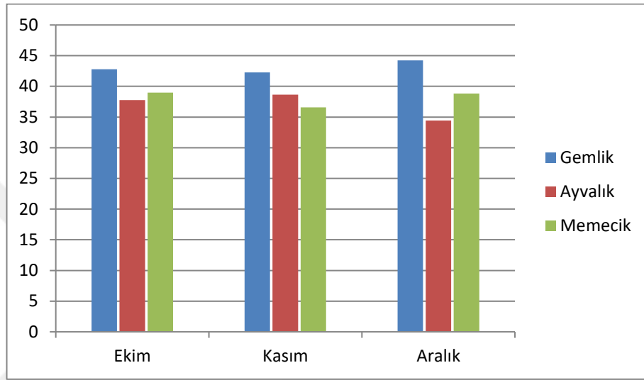
řekil 4.10.4. Gemlik, Ayvalık ve Memecik zeytinyađlarının triolein ieriklerinin olgunlařma dnemiyle deđiřimi (%)
