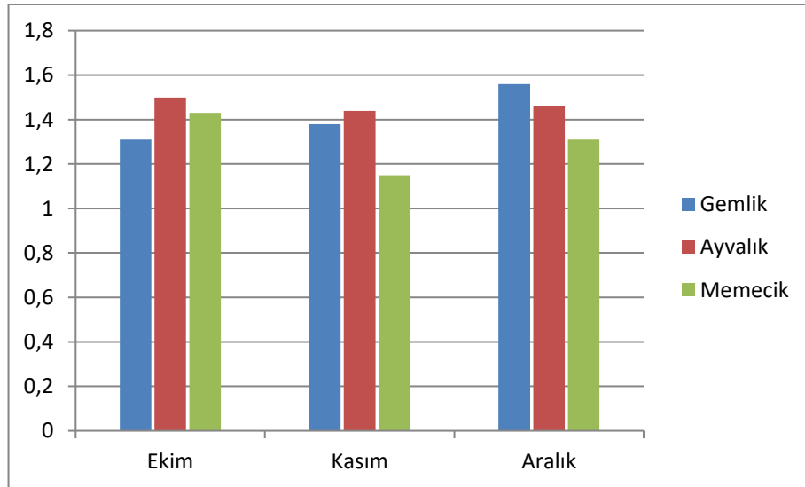
Şekil 4.6.1. Gemlik, Ayvalık ve Memecik zeytinyağlarının K_{232} içeliklerinin olgunlaşma dönemiyle değışimi
