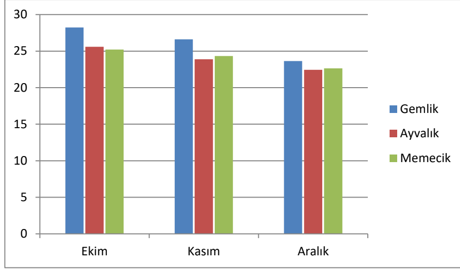
Şekil 4.10.5. Gemlik, Ayvalık ve Memecik zeytinyağlarının palmitodiolin içeriklerinin olgunlaşma dönemiyle değişimi (%)
