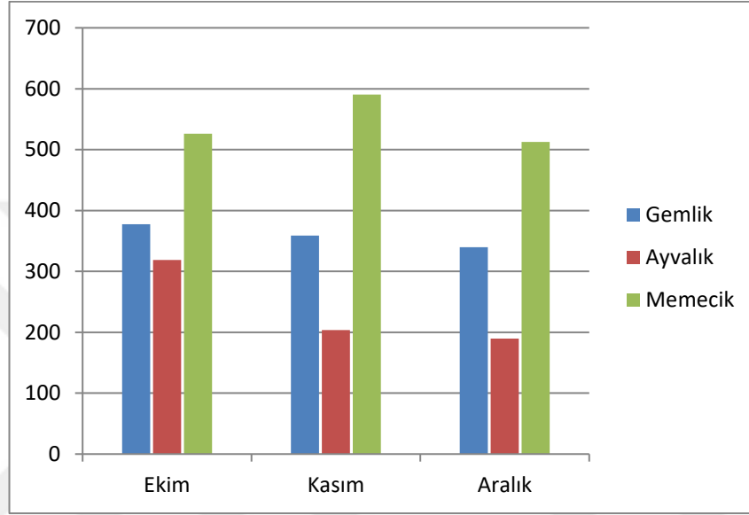
Şekil 4.11. Gemlik, Ayvalık ve Memecik zeytinyağlarının \alpha - tokoferol içeriklerinin olgunlaşma dönemiyle değişimi (mg/kg)
