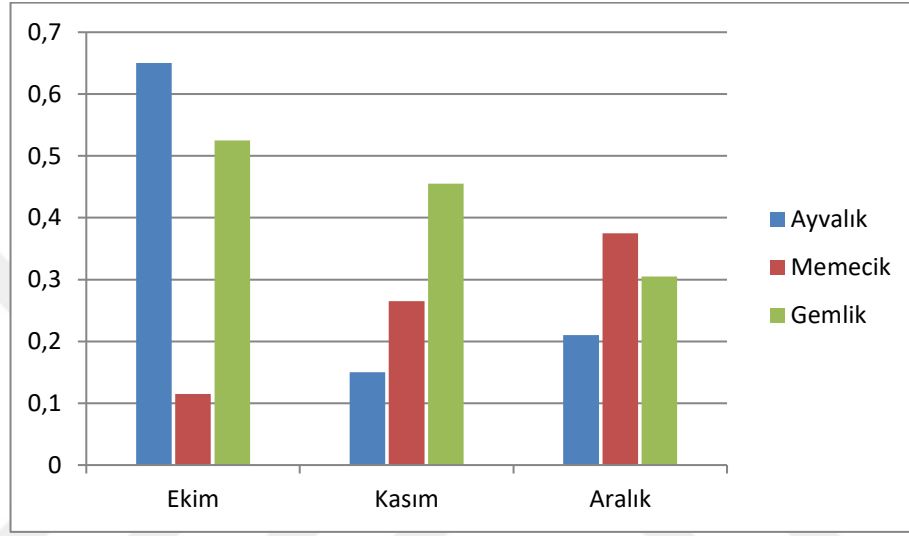
Şekil 4.12.7. Gemlik, Ayvalık ve Memecik zeytinyağlarının \Delta^7 -kampesterol içeriklerinin olgunlaşma dönemiyle değişimi (%)
