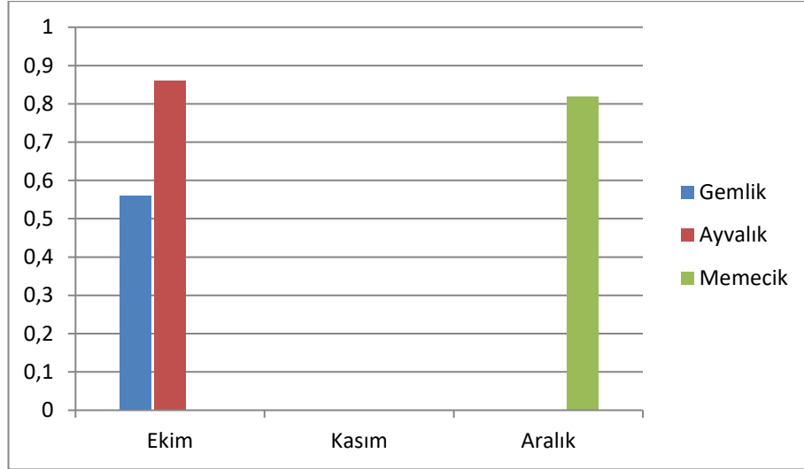
Şekil 4.13.12. Gemlik, Ayvalık ve Memecik zeytinyağlarının 3-hidroksitirozol içeriklerinin olgunlaşma dönemiyle değişimi (mg/100g)
