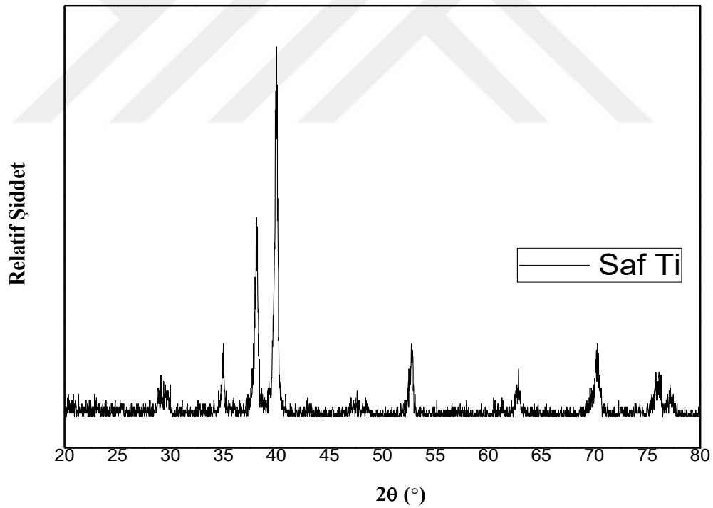
Şekil 5 1. Titanyum Tozun XRD Patterni
