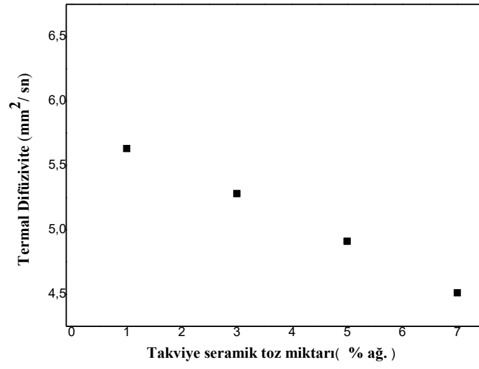
Şekil 5. 7. Kompozitlerin Termal Difüzyivite Değerlerinin Değişimi
