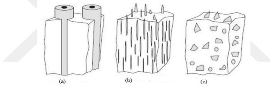
Şekil 2.1. Takviye Şekilleri (a) Monofilament, (b) Kesikli lifler, (c) Partiküller
