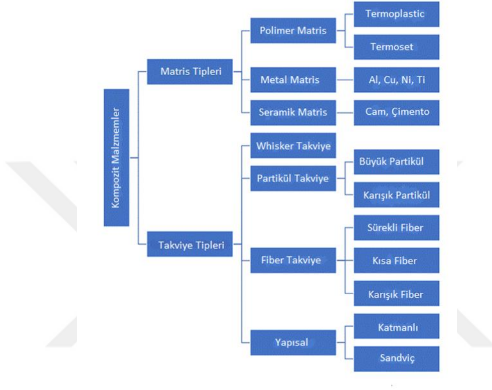
Şekil 2.3. Kompozit Malzemelerin Sınıflandırılması
