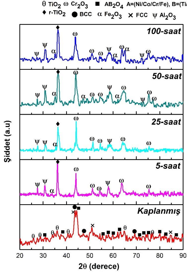
Şekil 4.30: MA + APS tekniğiyle üretilen AlCoCrFeNiTi YEA içerikli TBC numunelerine ait 1200°C'de sıcaklıkta farklı sürelerdeki oksidasyon testi sonrası XRD analizi
