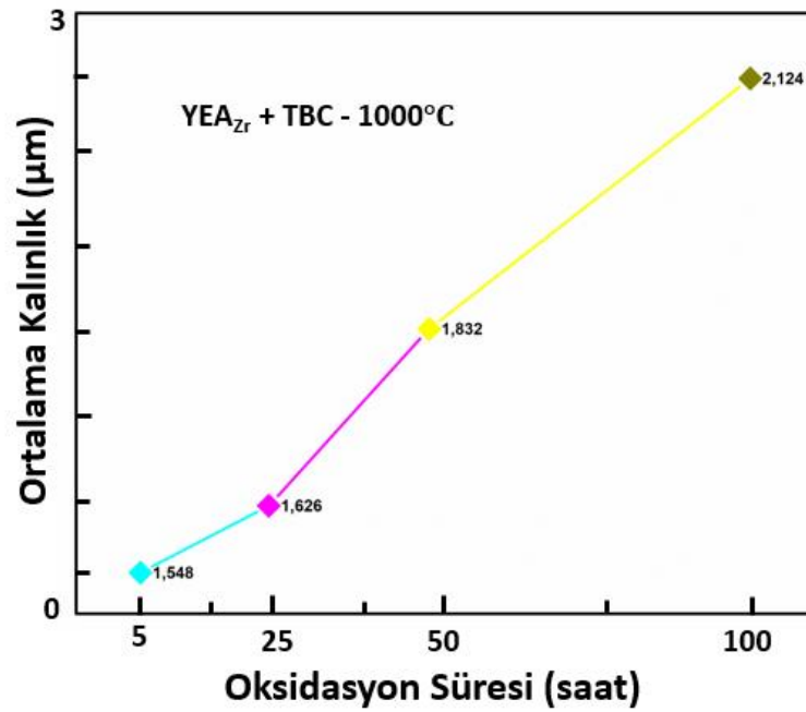
Şekil 4.16: Zr katkılı YEA TBC sisteminin 1000°C oksidasyon sonrası TGO tabakası kalınlık grafiği
