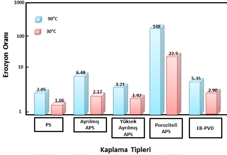
Şekil 2.46: APS ve EB-PVD TBC kaplamaların 700°C’de 30°- 90° açılarında erozif aşınmaya karşı dirençleri (Cernuschi, 2011).
