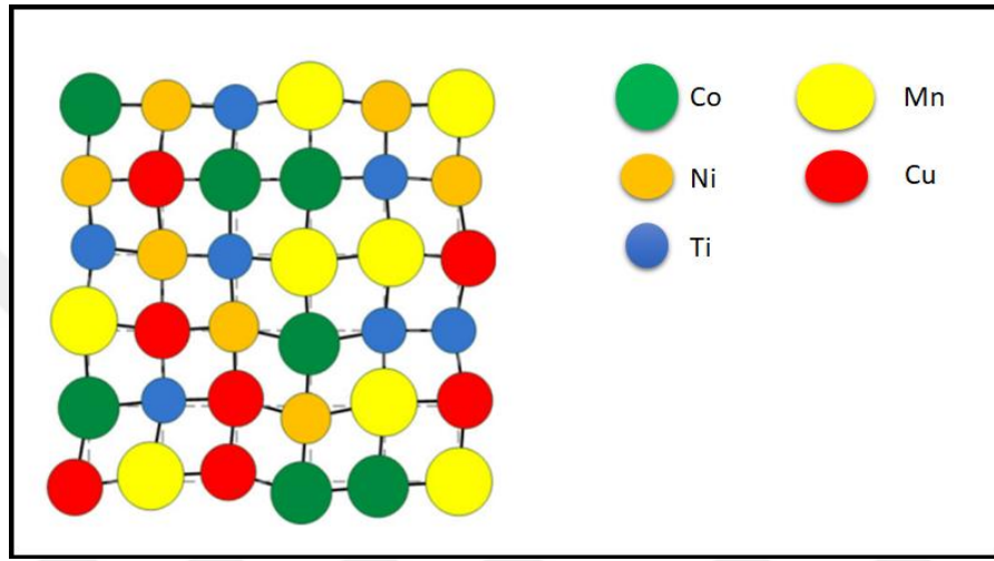
řekil 2.15: Kokteyl etkisi sonrası alařımın kafes örgü yapısının bozulması (Yeh, 2013).
