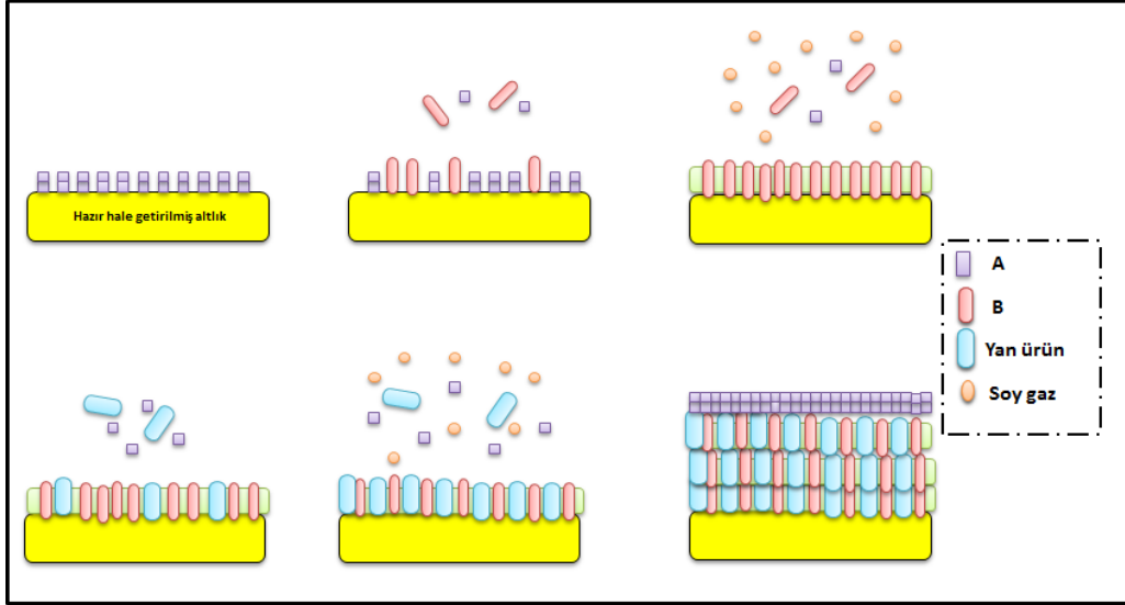
Şekil 2.34: ALD yönteminin şematik görünümü (Richard, 2014).
