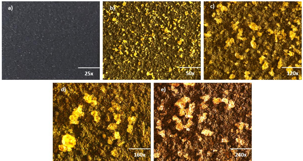
. Şekil 4.41:Ti katkılı YEA içerikli TBC sistemine ait 700^\circ\text{C} sıcak korozyon sonrası farklı büyütmelerdeki stereo mikroskop görüntüleri
