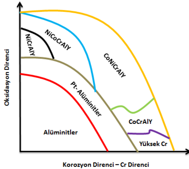
Şekil 2.4: Farklı bileşime sahip bağ kaplamaların oksidasyon ve korozyon hasarlarına karşı direnci (Özgürlük, 2020).
