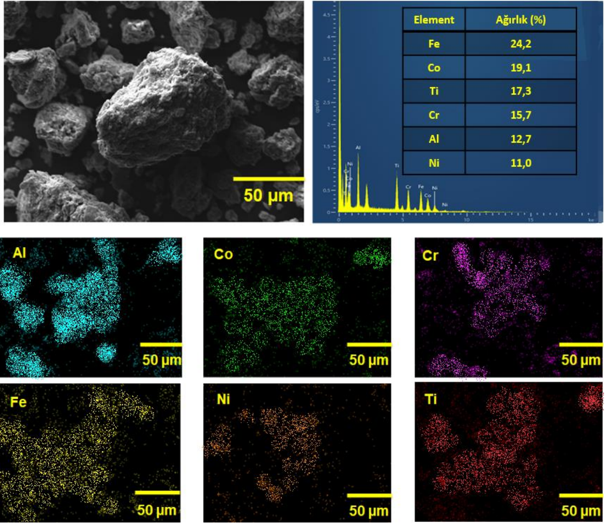
Şekil 3.10: 10 saatlik MA sonrası AlCoCrFeNiTi YEA tozunun SEM, EDS ve elementel haritalama analizi
