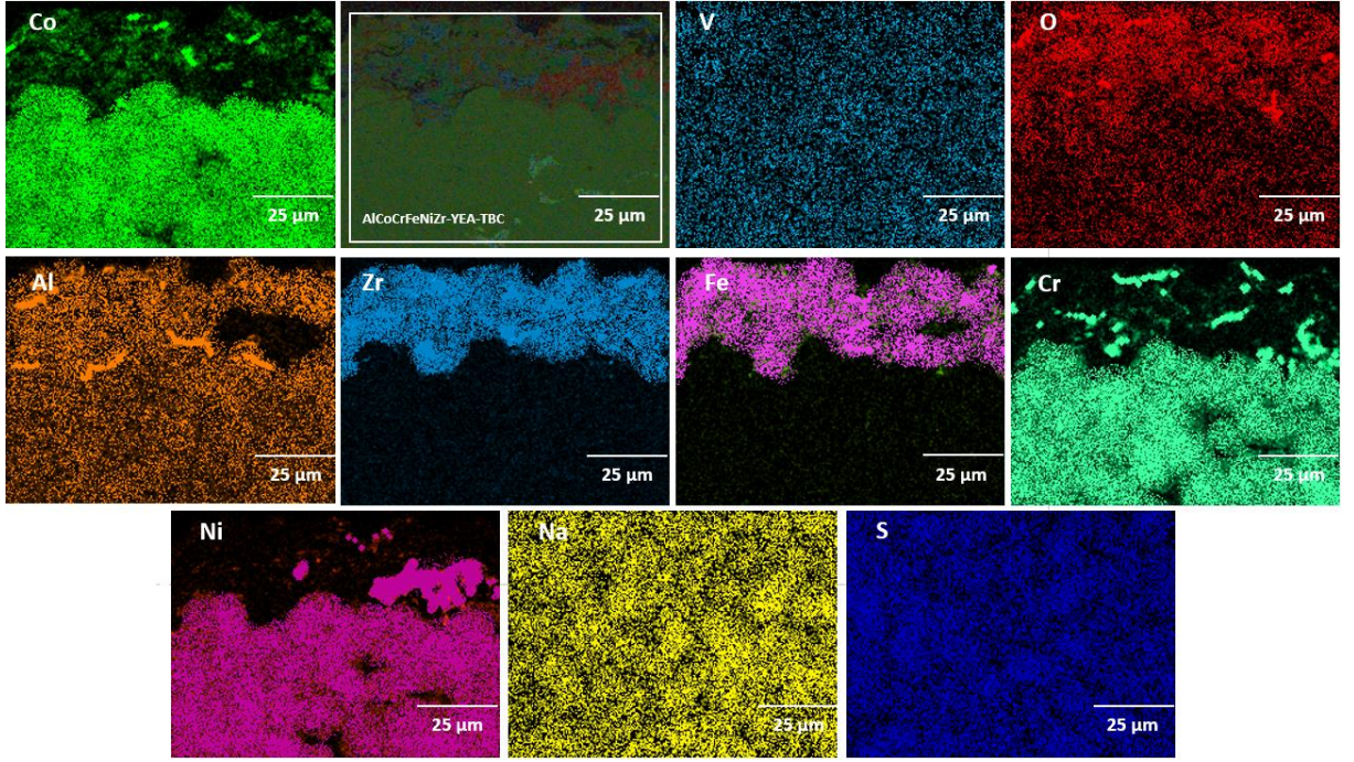
Şekil 4.50: Zr katkılı YEA içerikli TBC kaplamasına ait 700^\circ\text{C} ’de sıcak korozyon sonrası ara yüzey kesit alanından alınan elementel haritalama analizi
