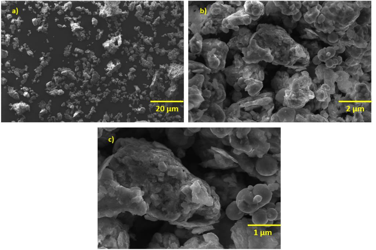
Şekil 3.12: 10 saatlik MA sonrası AlCoCrFeNiZr YEA tozunun; (a) 500X, (b) 5kX, (c) 10kx büyütmelelerdeki SEM üst yüzey görüntüleri
