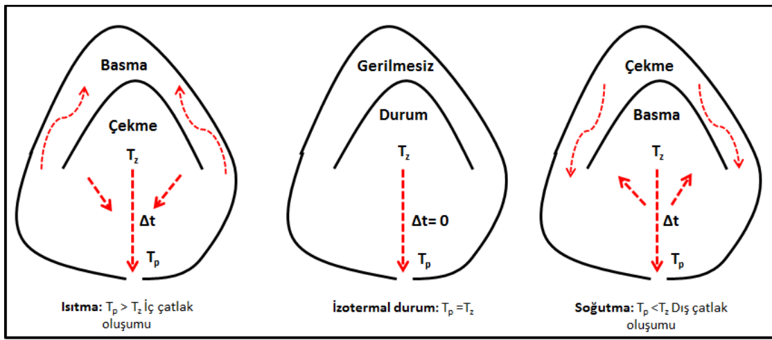
Şekil 2.49: Farklı termal şoklar altında gerilmelerin gösterimi (Karaoğlu, 2012).
