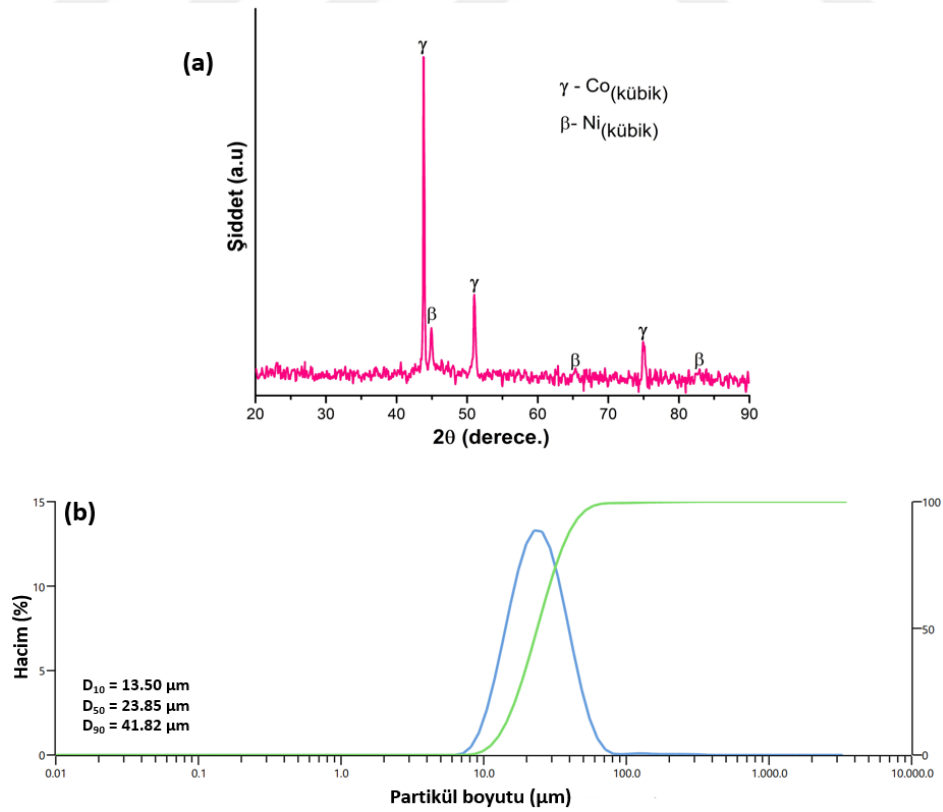
Şekil 3.3: CoNiCrAlY tozuna ait; (a) XRD grafięi, (b) partikül boyut daęılımı analizi
