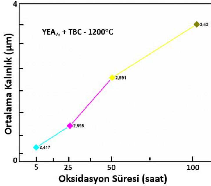
Şekil 4.37: Zr katkılı YEA TBC sisteminin 1200°C oksidasyon sonrası TGO tabakası kalınlık grafiği
