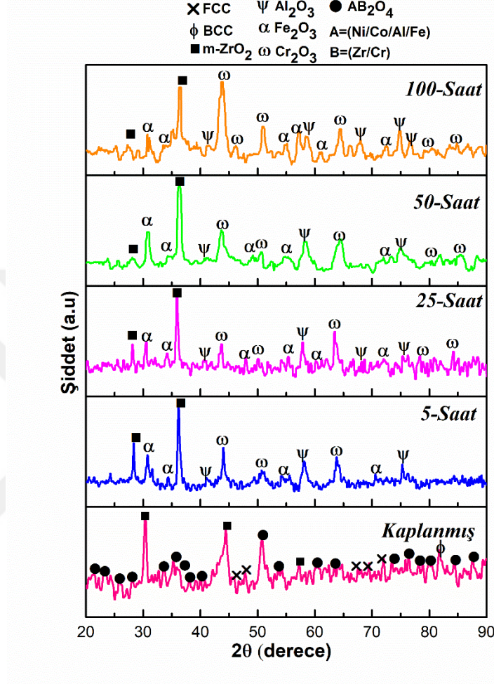
Şekil 4.34: MA + APS tekniğiyle üretilen AlCoCrFeNiZr YEA içerikli TBC numunelerine ait 1200°C’de sıcaklıkta farklı sürelerdeki oksidasyon testi sonrası XRD analizi
