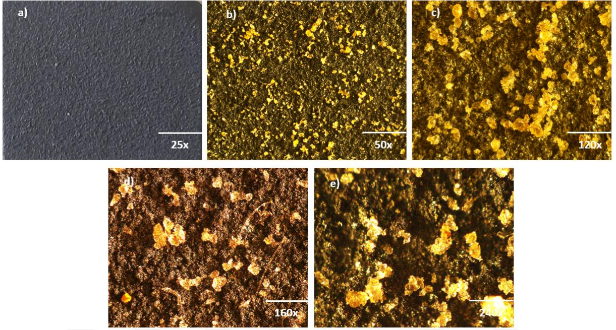
Şekil 4.47: Zr katkılı YEA içerikli TBC sistemine ait 700°C sıcak korozyon sonrası farklı büyütmelerdeki stereo mikroskop görüntüleri
