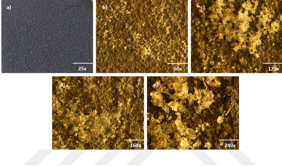
Şekil 4.59: Zr katkılı YEA içerikli TBC sistemine ait 800°C sıcak korozyon sonrası farklı büyütme ölçeklerindeki stereo mikroskop görüntüleri
