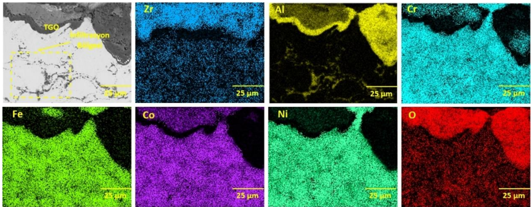
Şekil 4.36: MA + APS tekniğiyle üretilen AlCoCrFeNiZr YEA içerikli TBC sisteminde ait 1200°C sıcaklıkta 100 saat oksidasyon sonrasına ait elementel haritalama analizi
