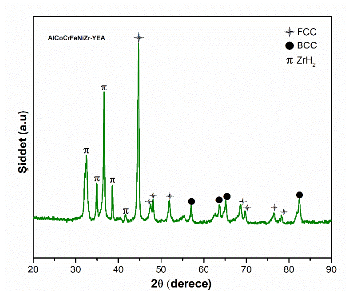
Şekil 3.13: 10 saatlik MA sonrası üretilen yeni nesil AlCoCrFeNiZr YEA tozunun XRD grafiği
