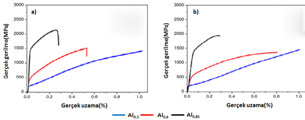
Şekil 2.17: Al içeriğine göre YEA'nın gerçek gerilme – birim uzama grafiğindeki değişim; (a) lazer ile sinterleme sonrası, (b) ark ergitme yöntemi sonrası (Alaneme, 2016).
