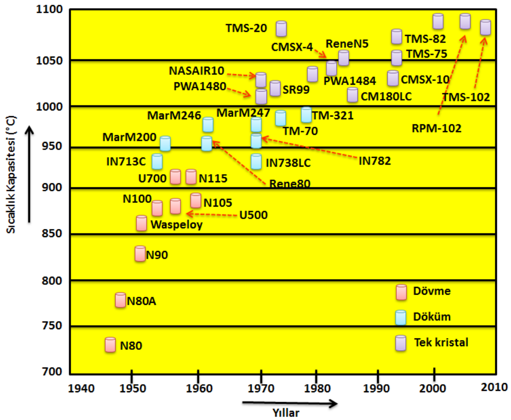
Şekil 2.3: Tarih boyunca farklı özellik sergileyen süper alaşımların sıcaklık dayanımını gösteren grafik (Aydınmakina, 2014).
