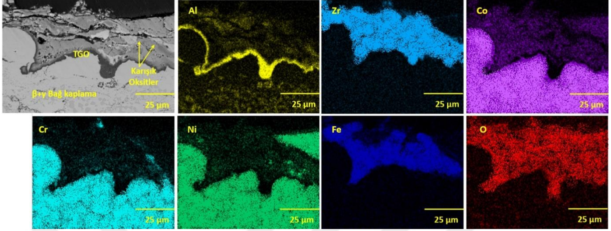
Şekil 4.26: MA + APS tekniğiyle üretilen AlCoCrFeNiZr YEA içerikli TBC sistemine ait 1100°C sıcaklıkta 100 saat oksidasyon sonrasında ait elementel haritalama analizi
