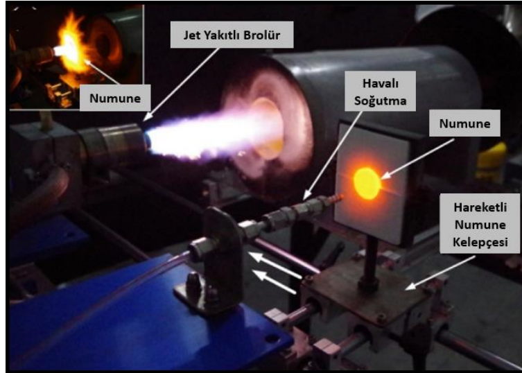
Şekil 2.50: Brolürlü Termal Şok/Çevrim Test Sisteminin görünümü (Zhoungliu, 2016).
