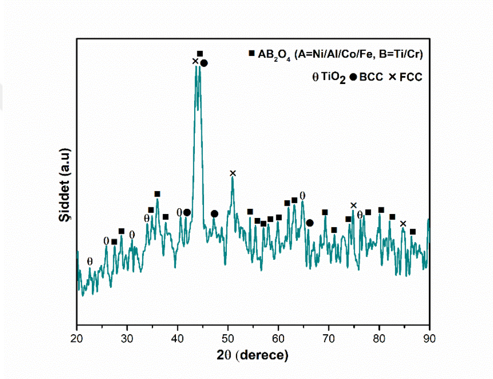
Şekil 4.3: MA + APS sonrası üretilen yeni nesil üst kaplama olarak AlCoCrFeNiTi YEA içerikli TBC sistemine ait kaplanmış XRD analizi
