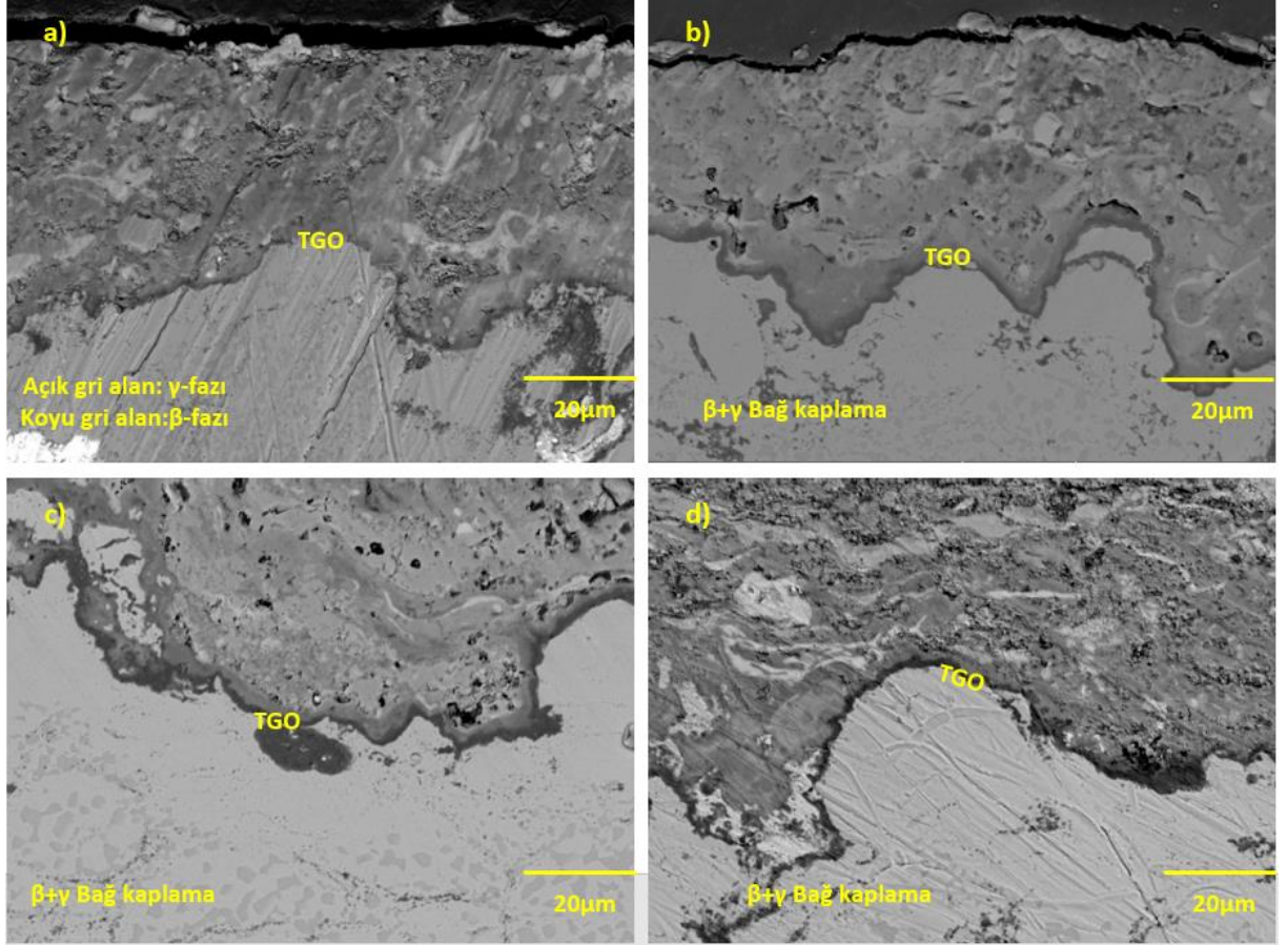
Őekil 4.13: MA + APS tekniđiyle retilen AlCoCrFeNiZr YEA ierikli TBC numunelerine ait 1000°C'de sıcaklıkta oksidasyon sonrası SEM grntleri; (a) 5 saat, (b) 25 saat, (c) 50 saat, (d) 100 saat
