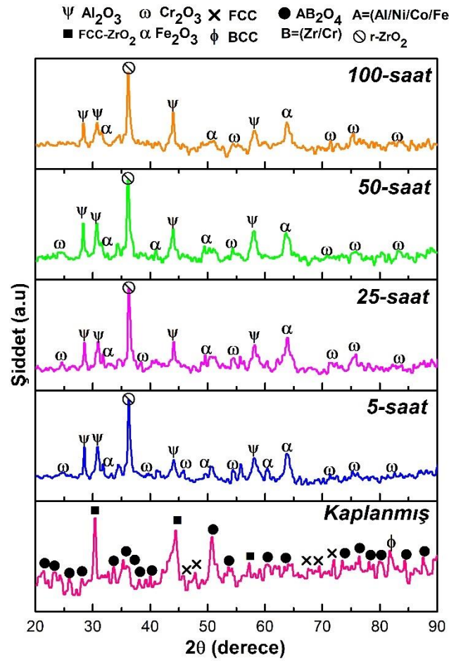
Şekil 4.24: MA + APS tekniğiyle üretilen AlCoCrFeNiZr YEA içerikli TBC numunelerine ait 1100^\circ\text{C} 'de sıcaklıkta farklı sürelerdeki oksidasyon testi sonrası XRD analizi
