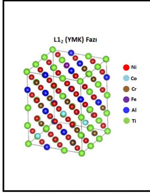
Şekil 2.19: L_{12} faz yapısına sahip bir alaşımanın şematik görünümü (Yang, 2018).
