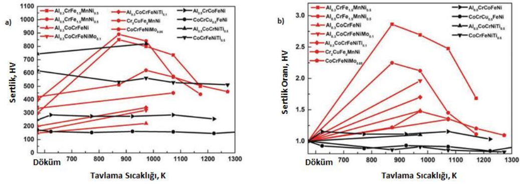
Şekil 2.38: YEA'ların sertliği üzerindeki tavlama ısı işlemi; (a) sertlik değerleri, (b) sertlik oranı (Michael, 2016).
