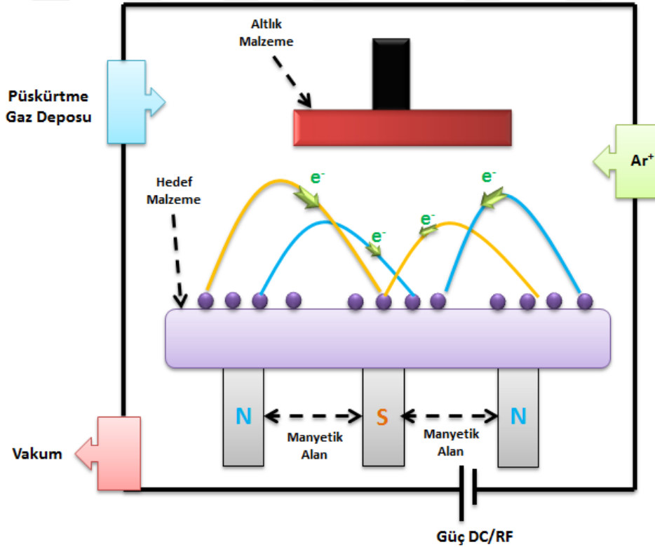
Şekil 2.32:Magnetron püskürtme yönteminin şematik görünümü (Jain, 2016).
