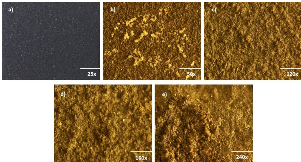
Şekil 4.65: Ti katkılı YEA içerikli TBC sistemine ait 900°C sıcak korozyon sonrası farklı büyütme ölçeklerindeki stereo mikroskop görüntüleri
