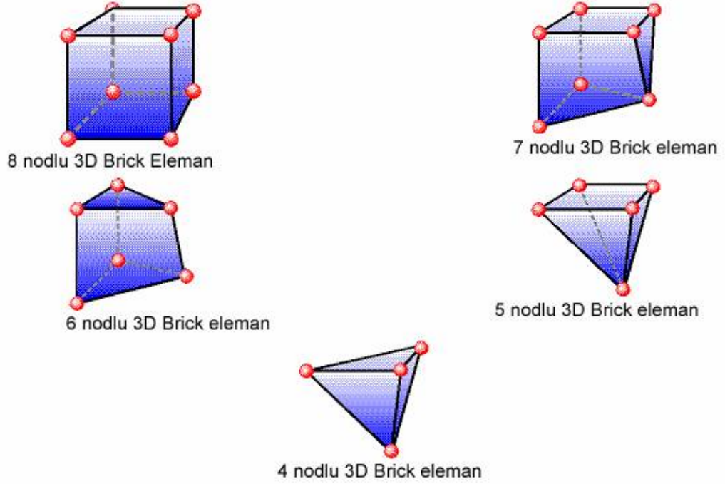
Şekil 3.58 : Bricks ve Tetrahedra katı modelleme sistemi.
