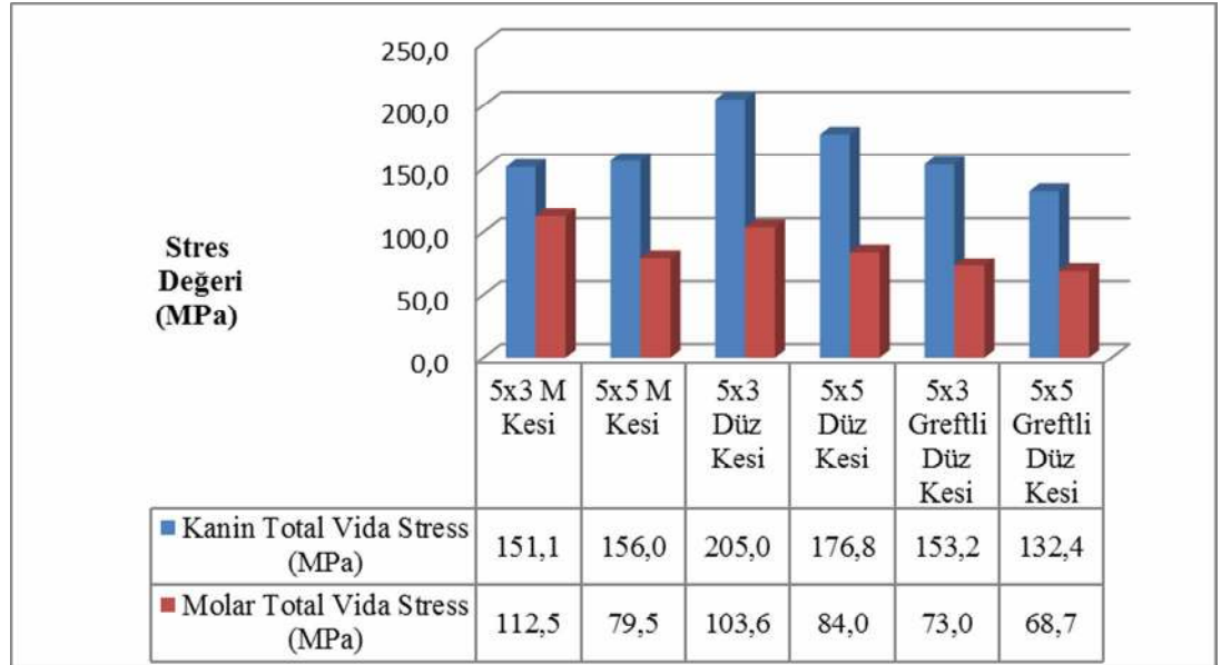
Şekil 4.1 : Vidalar üzerinde oluşan Von Misses stres değerleri.
