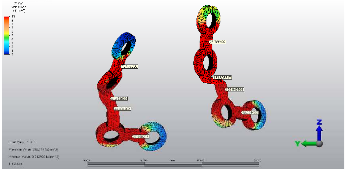
Şekil 4.26 : 5 mm maksiller ilerletme, 3 mm inferior hareket ile düz kesi uygulanan çalışma grubundan plaklarda oluşan Von Misses stres dağılımı.
