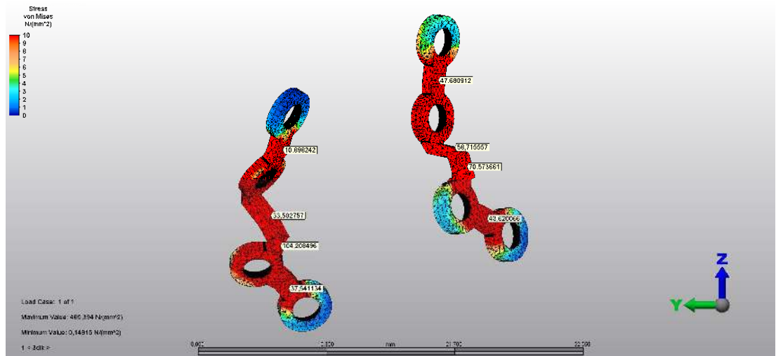
Şekil 4.25 : 5 mm maksiller ilerletme, 5 mm inferior hareket ile M-kesi uygulanan çalışma grubundan plaklarda oluşan Von Misses stres dağılımı.
