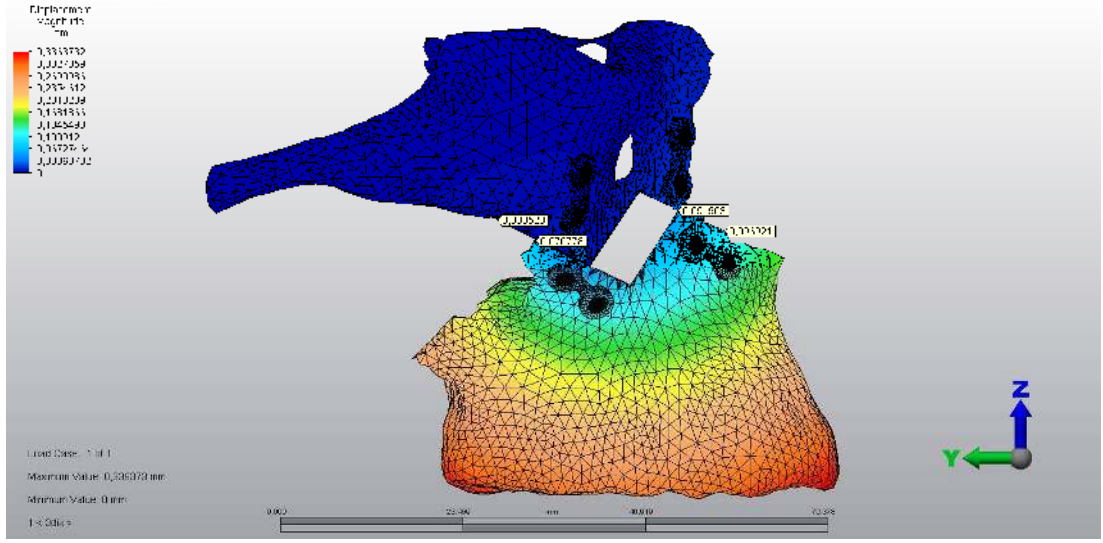
Şekil 4.38 : 5 mm maksiller ilerletme, 3 mm inferior hareket ile M-kesi uygulanan çalışma grubunda kanin yükleme sonucunda oluşan deplasman miktarı.
