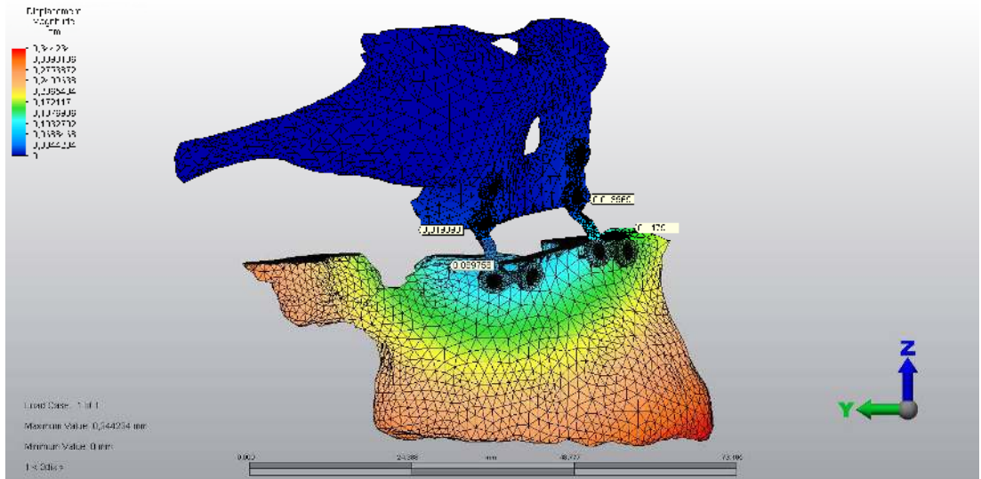
Şekil 4.41 : 5 mm maksiller ilerletme, 5 mm inferior hareket ile düz kesi uygulanan çalışmada kanin yükleme sonucunda oluşan deplasman miktarı.
