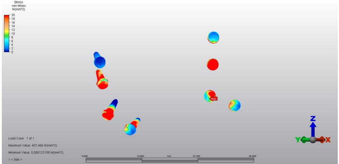
Şekil 4.3 : 5 mm maksiller ilerletme, 5 mm inferior hareket uygulanan M-kesi çalışma grubu vidalar üzerindeki Von Misses stres değerleri.
