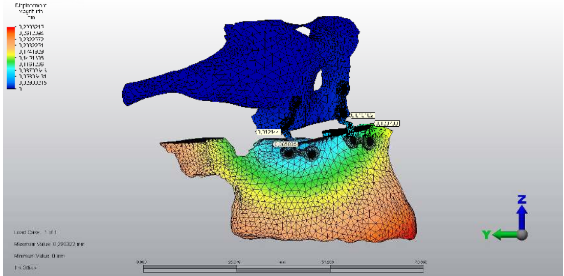
Şekil 4.40 : 5 mm maksiller ilerletme, 3 mm inferior hareket ile düz kesi uygulanan çalışmada kanin yükleme sonucunda oluşan deplasman miktarı.
