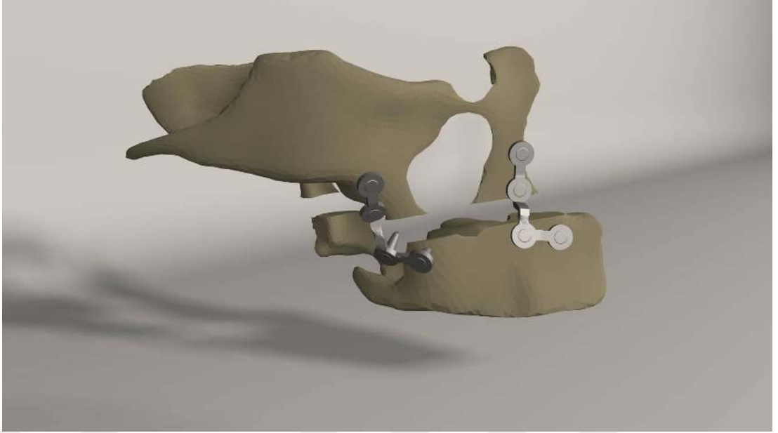
Şekil 3.52 : 5 mm maksiller ilerletme 3 mm inferior hareket uygulanan greftli düz kesi yapılmış çalışma grubuna uyumlandırılan vida ve plakların spongioz kemikteki görünümü.
