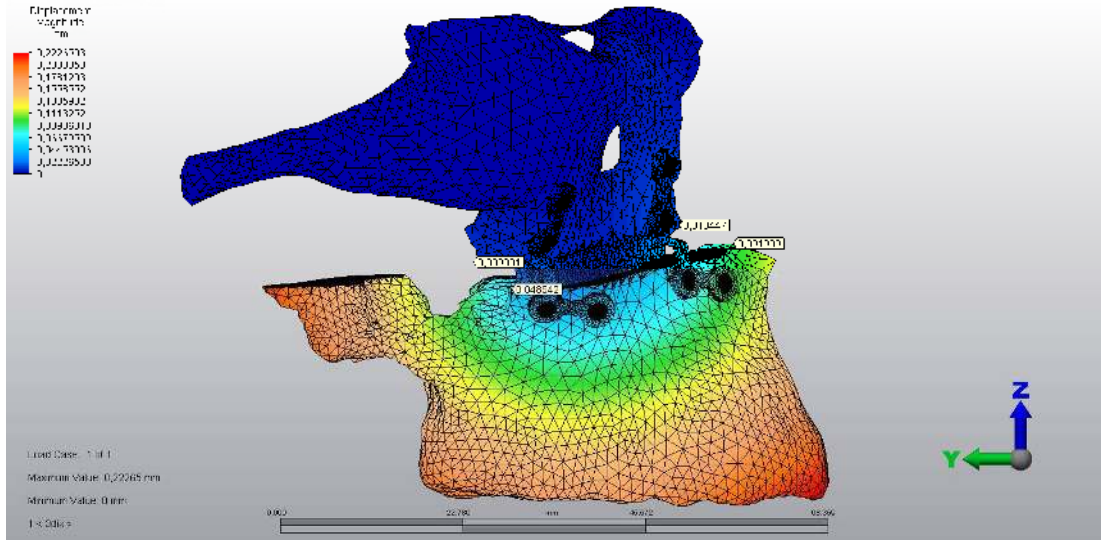
Şekil 4.42 : 5 mm maksiller ilerletme, 3 mm inferior hareket ile greftli düz kesi uygulanan çalışmada kanin yükleme sonucunda oluşan deplasman miktarı.
