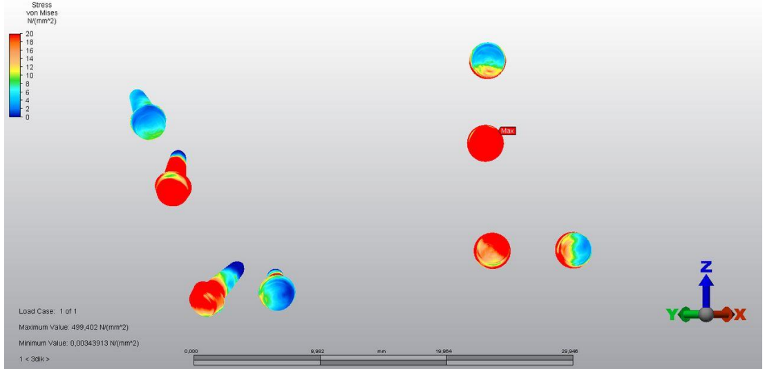
Şekil 4.5 : 5 mm maksiller ilerletme, 5 mm inferior hareket uygulanan greftsiz düz kesi çalışma grubu vidalar üzerindeki Von Misses stres değerleri.
