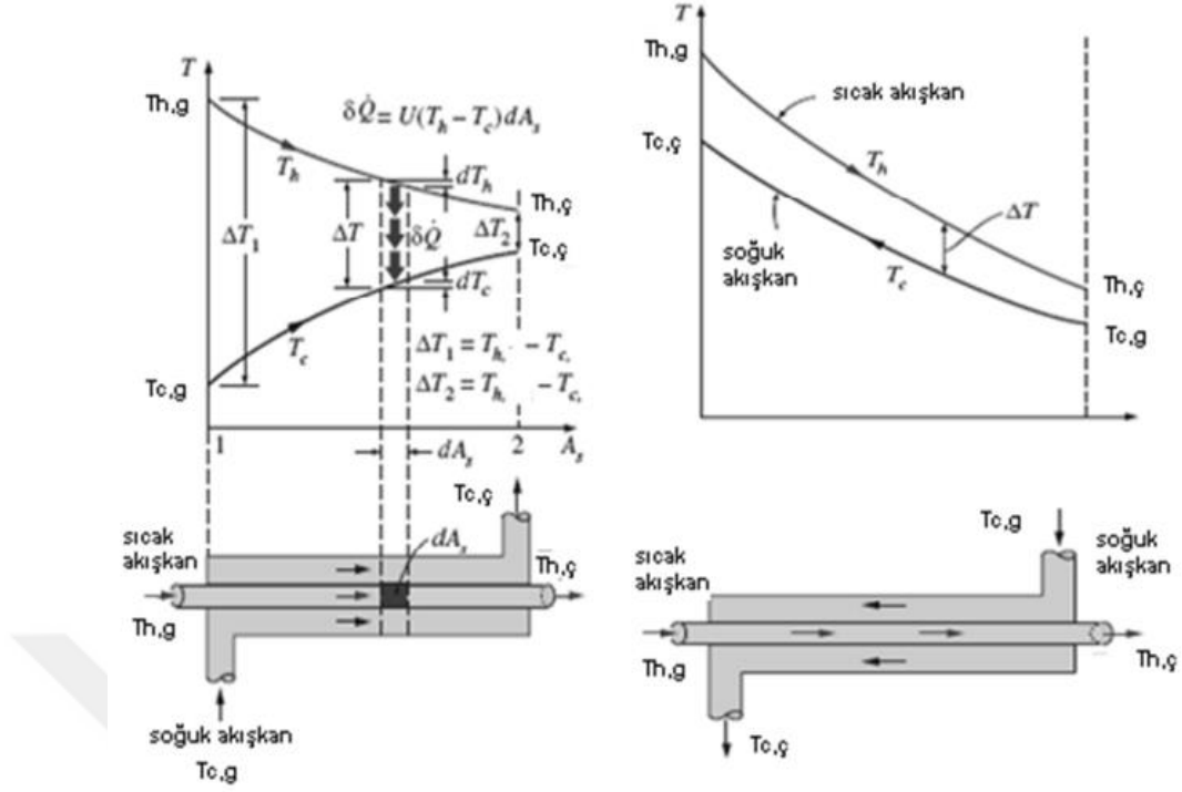
Şekil 4.15. Paralel ve çapraz akışlı eşanjörlerde sıcaklık fark grafiği (Çengel, 2002)
