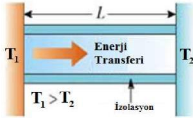
Şekil 3.2. Kondüksiyon yolu ile ısı transferi (MEB-I)
