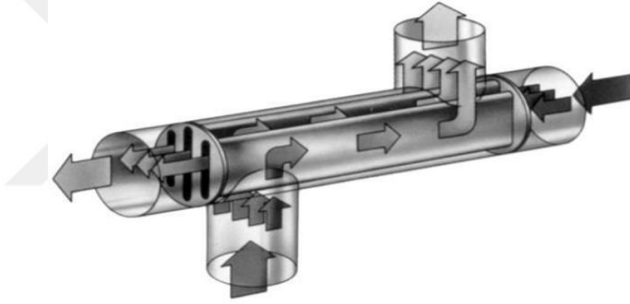
řekil 3.25. Lamelli ısı deęiřtiricisi (Kaya, 2013)
