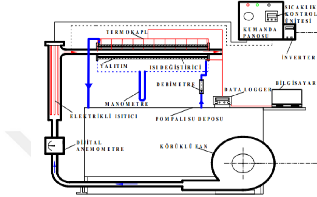
Şekil 2.4. Ölçüm cihazlarının şematik görünümü (Baysal, 2008)
