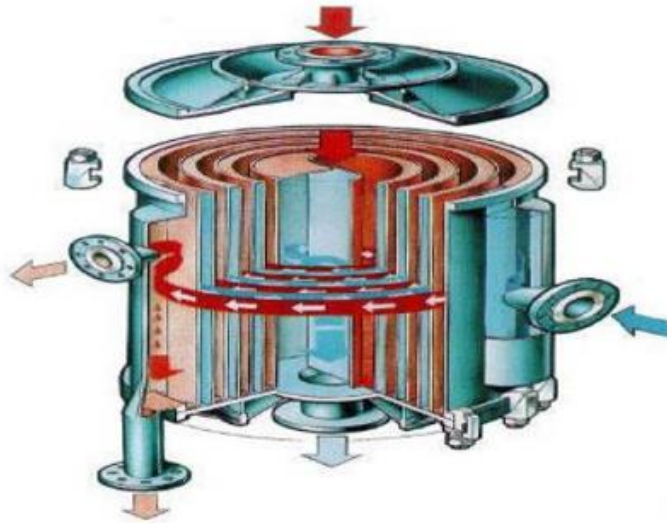
Şekil 3.24. Spiral borulu ısı değıştircileri (Ertaylan, 2012)
