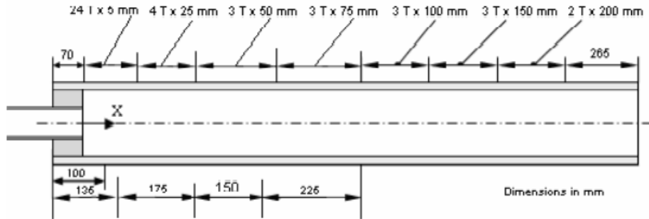
Şekil 2.1. Test çıkış borusundaki termokupl dağılımı (Migay ve Golubev, 1970)
