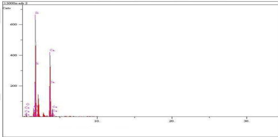
Şekil 4.34. %25 uçucu kül katkılı numuneye ait eds grafiği ve değerleri.
