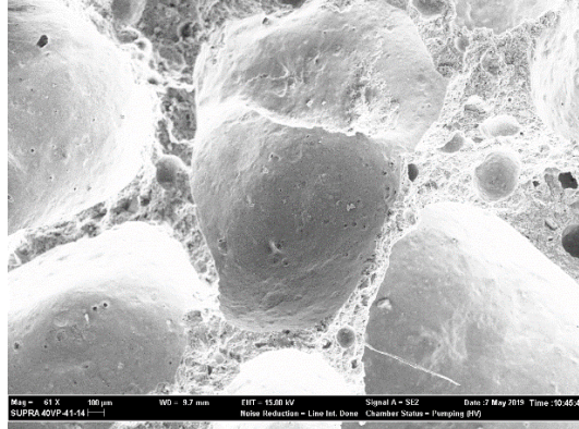
Şekil 4.31. %25 riylit katkılı numunenin sem görüntüsü (60 x).
