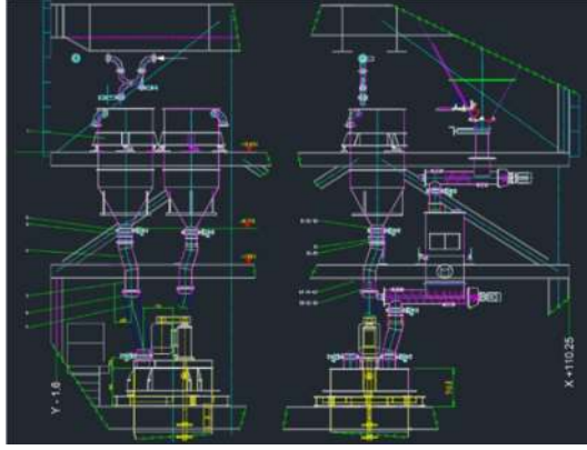
a) Döküm Ünitesi ve Sloların kesit görünüşü
