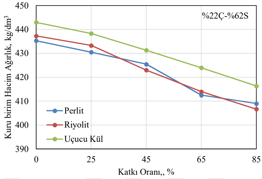
Şekil 4.16. Mineral katkı oranının kuru birim hacim ağırlığa etkisi (%22Ç-%62sk).
