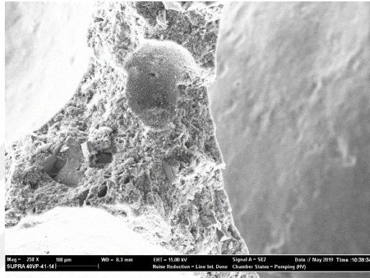
Şekil 4.29. %25 perlit katkılı numunenin sem görüntüsü (250 x).
