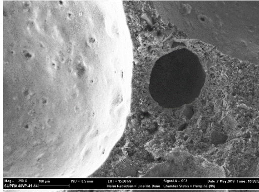
Şekil 4.27. %25 uçucu kül katkılı numunenin sem görüntüsü (250 x).
