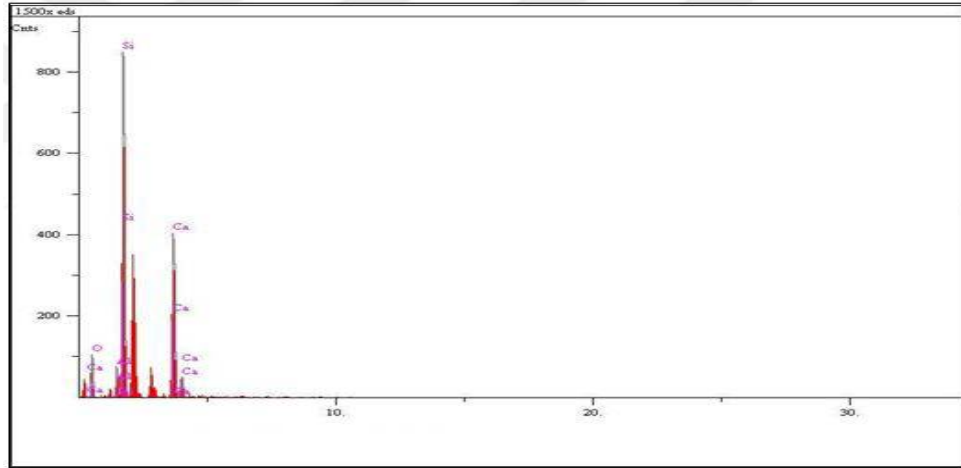
Şekil 4.33. %25 riylit katkılı içeren numuneye ait eds grafiği ve değerleri.
