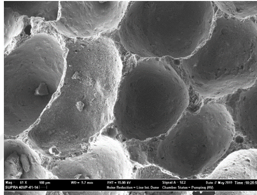
Şekil 4.26. %25 uçucu kül katkılı numunenin sem görüntüsü (60x).
