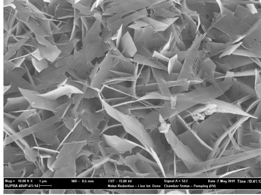
Şekil 4.28. %25 perlit katkılı numunenin sem görüntüsü (10k x).
