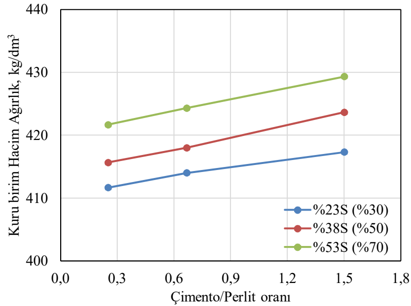
Şekil 4.19. Farklı silis kumu içeren karışımlarda çimento/perlit oranının kuru birim hacim ağırlığına etkisi.
