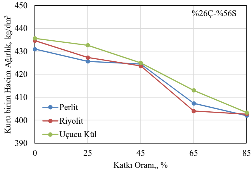
Şekil 4.17. Mineral katkı oranının kuru birim hacim ağırlığa etkisi (%26Ç-%56sk).
