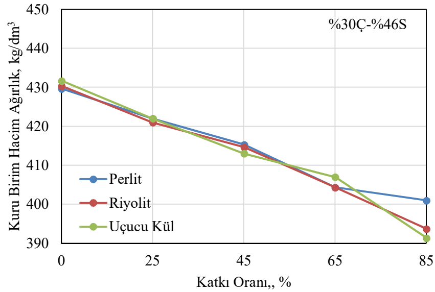
Şekil 4.18. Mineral katkı oranının kuru birim hacim ağırlığına etkisi (%30Ç-%46sk).
