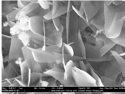
Şekil 4.30. %25 riyolit katkılı numunenin sem görüntüsü (10k x).
