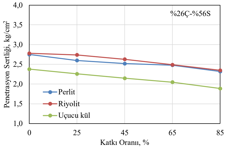
Şekil 4.7. Mineral katkı oranının penetrasyon sertliğine etkisi (%26Ç-%56sk).
