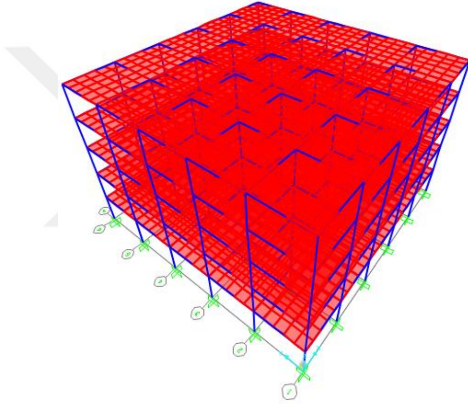
Şekil 2.6. İncelenen binanın sonlu eleman modeli
