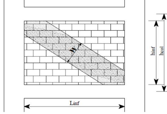
Şekil 1.2. Eşdeğer diyagonal basınç çubuğu
