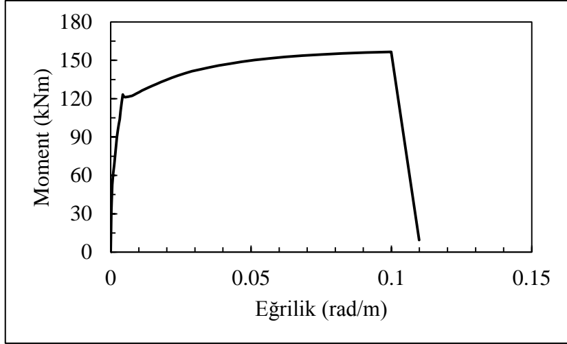
Şekil 3.21. Kirişler için elde edilen moment-eğrilik ilişkisi
