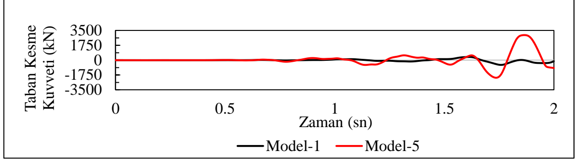
Şekil 3.8. Dolgu duvarların kapasitesine erişinceye kadar taban kesme kuvveti deęişimi
