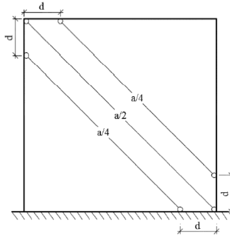
Şekil 1.4. Çoklu diyagonal basınç çubuğu modeli
