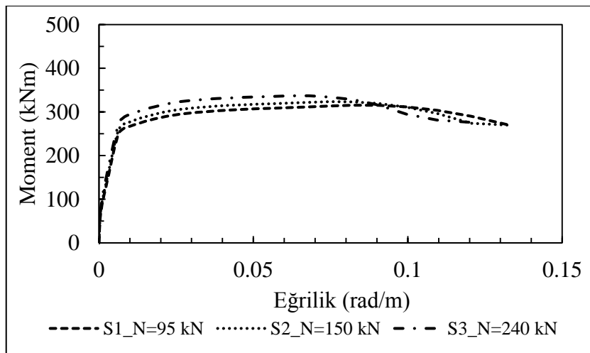
Şekil 3.22 (devamı). Kolonlar için elde edilen moment-eğrilik ilişkileri
