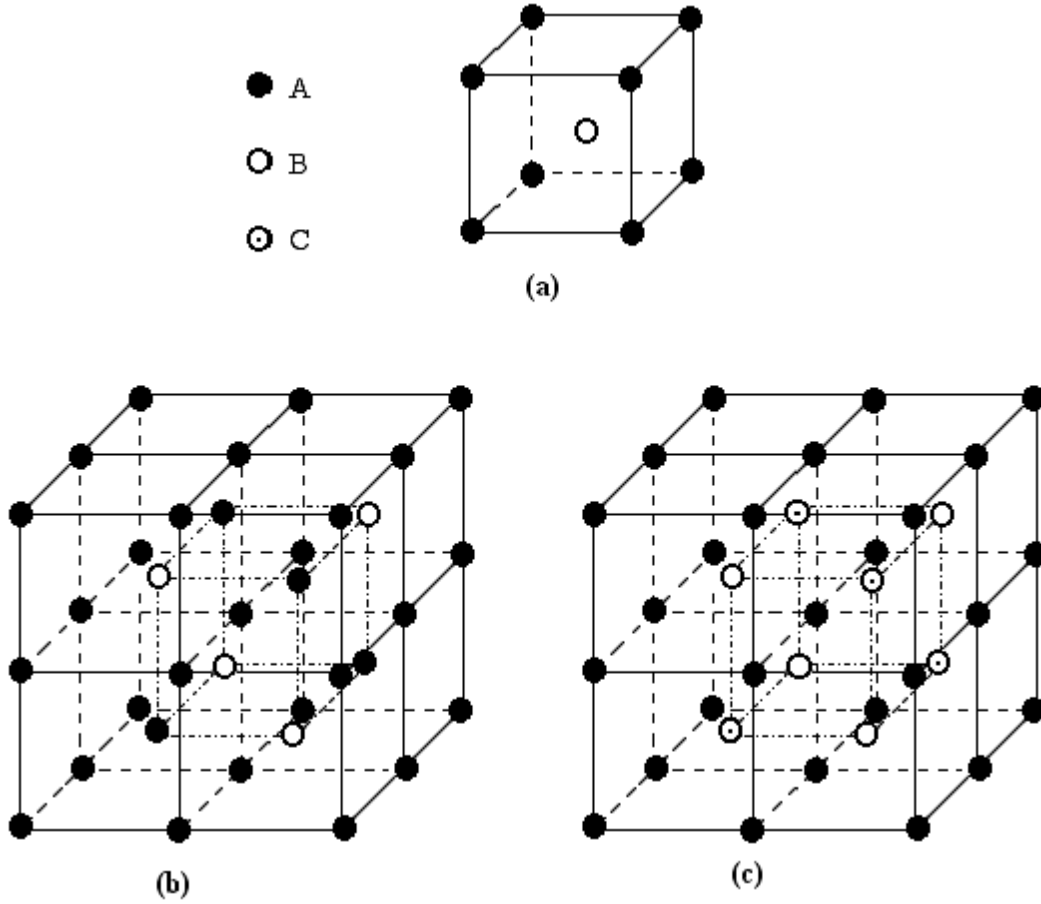
Şekil 3.1. Şekil hatırlama özelliğine sahip düzenli kristal yapı birim hücreleri a) CsCl yapı, b) \text{Fe}_3\text{Al} yapı, c) \text{Cu}_2\text{MnAl} tipi yapı [10].
