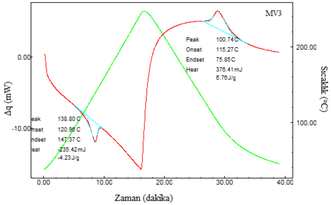
Şekil 6.27. MV3 alaşımı için 15 °C/dk. ısıtma ve soğutma hızı için elde edilen DSC eğrisi.
