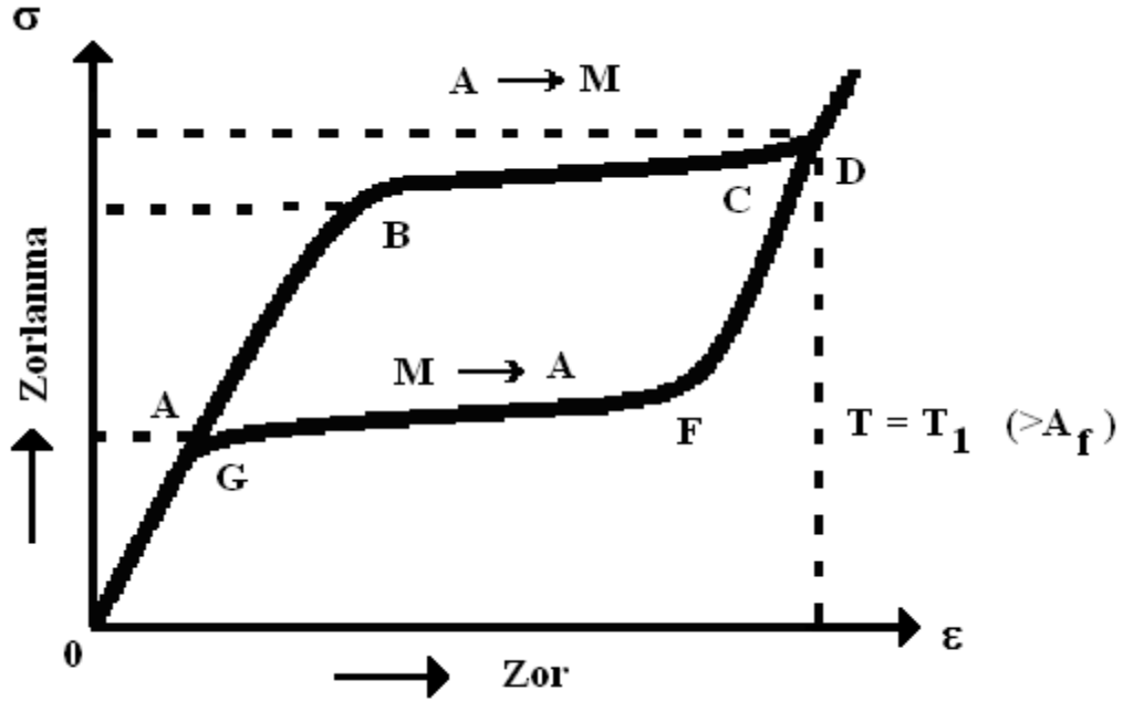
Şekil 3.8. Süperelastiklik histerisisinin şematik gösterimi [1].
