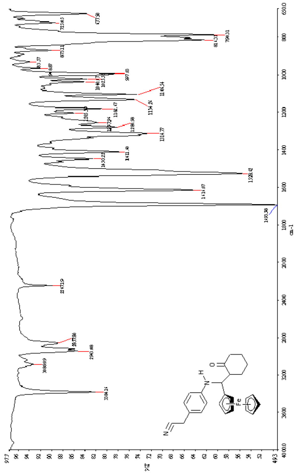
Şekil 5. 87 Bileşik 14' ün FTIR NMR spektrumu
