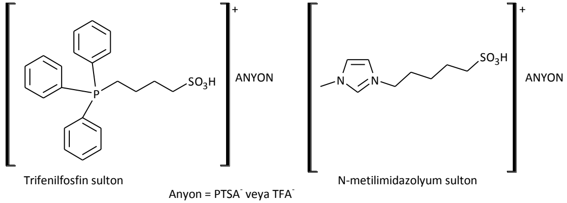
Şekil 3. 14 N-metil imidazol, trifenilfosfinin, PTSA ve TFA ile oluşturulan iyonik sıvı
