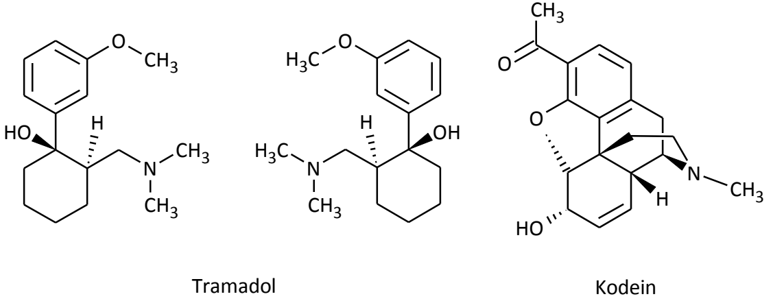
Şekil 6. 3 Tramadol ve Kodein bileşiklerinin molekül yapıları
