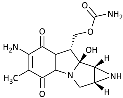
Şekil 4. 10 Mitomicinin molekül yapısı
