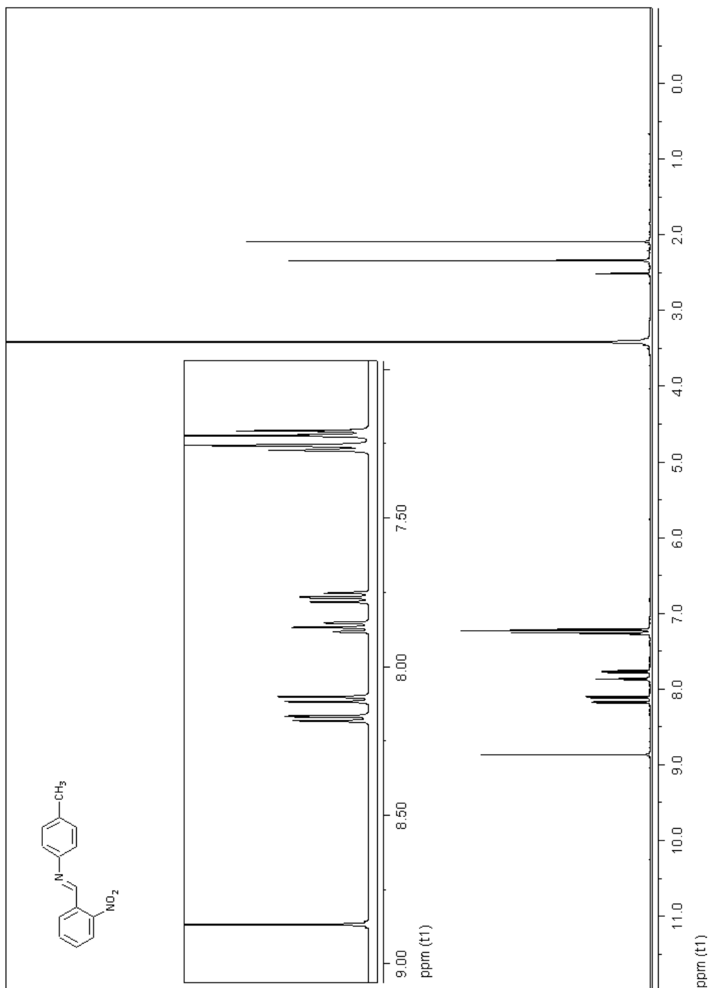
Şekil 5. 94 Bileşik 15' in 1 H NMR spektrumu
