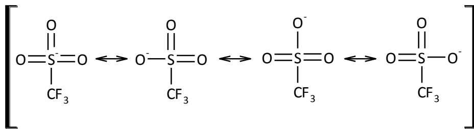
Şekil 3. 2 Triflatın rezonans yapısı
