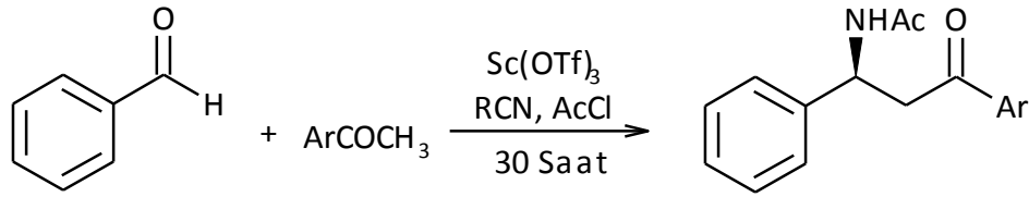
Şekil 3. 4 \text{Sc(OTf)}_3 varlığında tek-kaplı üç bileşenli \beta -asetamido ketonların sentezi
