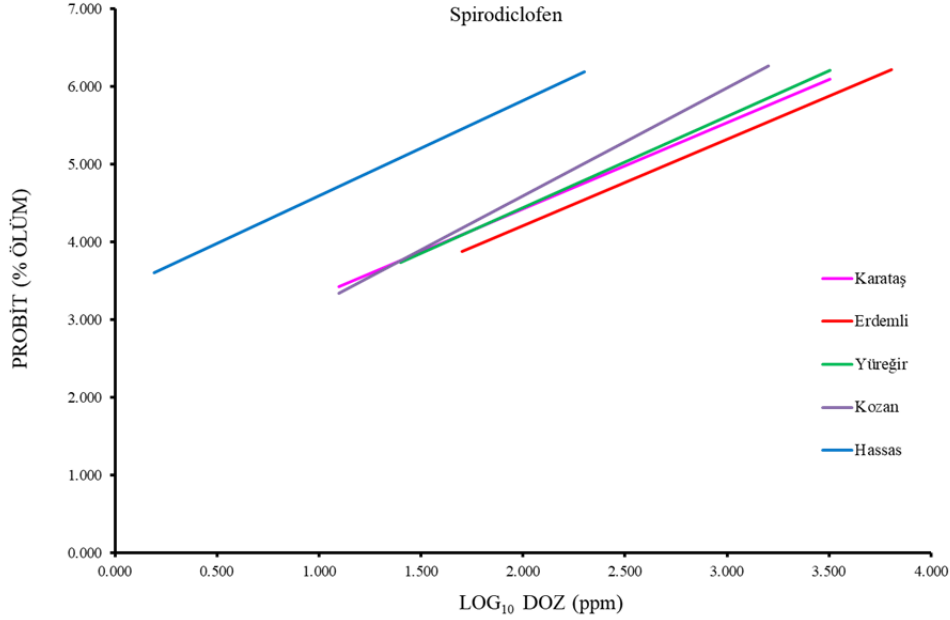
Şekil 4.4. Farklı Phyllocoptruta oleivora popülasyonlarının spirodiclofen etkili maddeli akarısitelerle karşı göstermiş oldukları logaritmik doz-probit (% ölüm) eğrileri.
