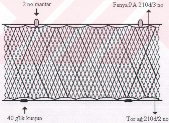
Şekil 3.2. Çalışmada kullanılan multifilament fanyalı uzatma ağların yapısı
