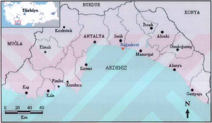
Şekil 3.1. Çalışmanın gerçekleştirildiği araştırma bölgesi
