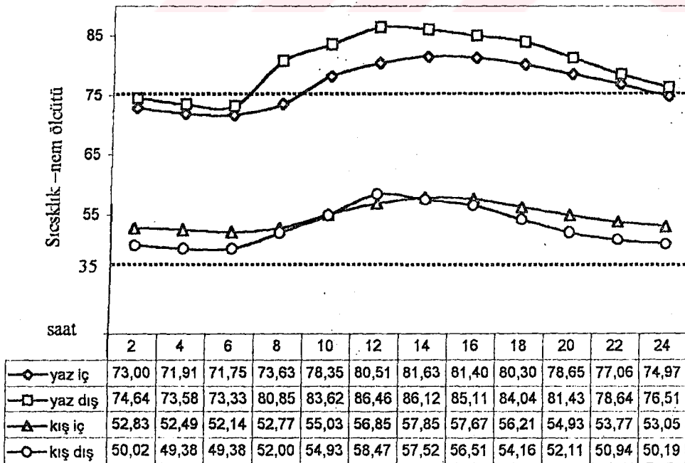
Şekil 5.5. Yaz ve kış mevsimlerindeki sıcaklık-nem ölçütü değerlerinin değişimi
