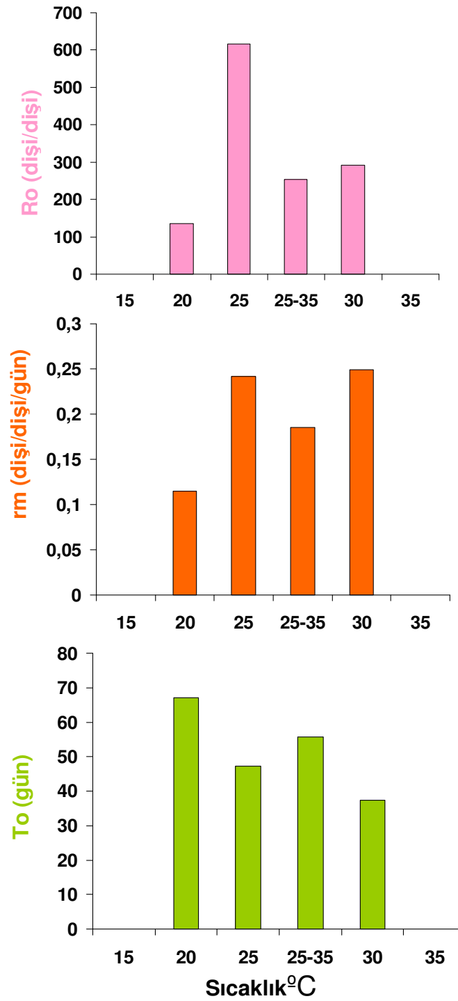
Şekil 4.4. Cheilomenes propinqua 'nın net üreme gücü ( R_o ), kalıtsal üreme kapasitesi ( r_m ) ve ortalama döl süresi ( T_o ) değerlerinin sıcaklıklara göre değişimi
