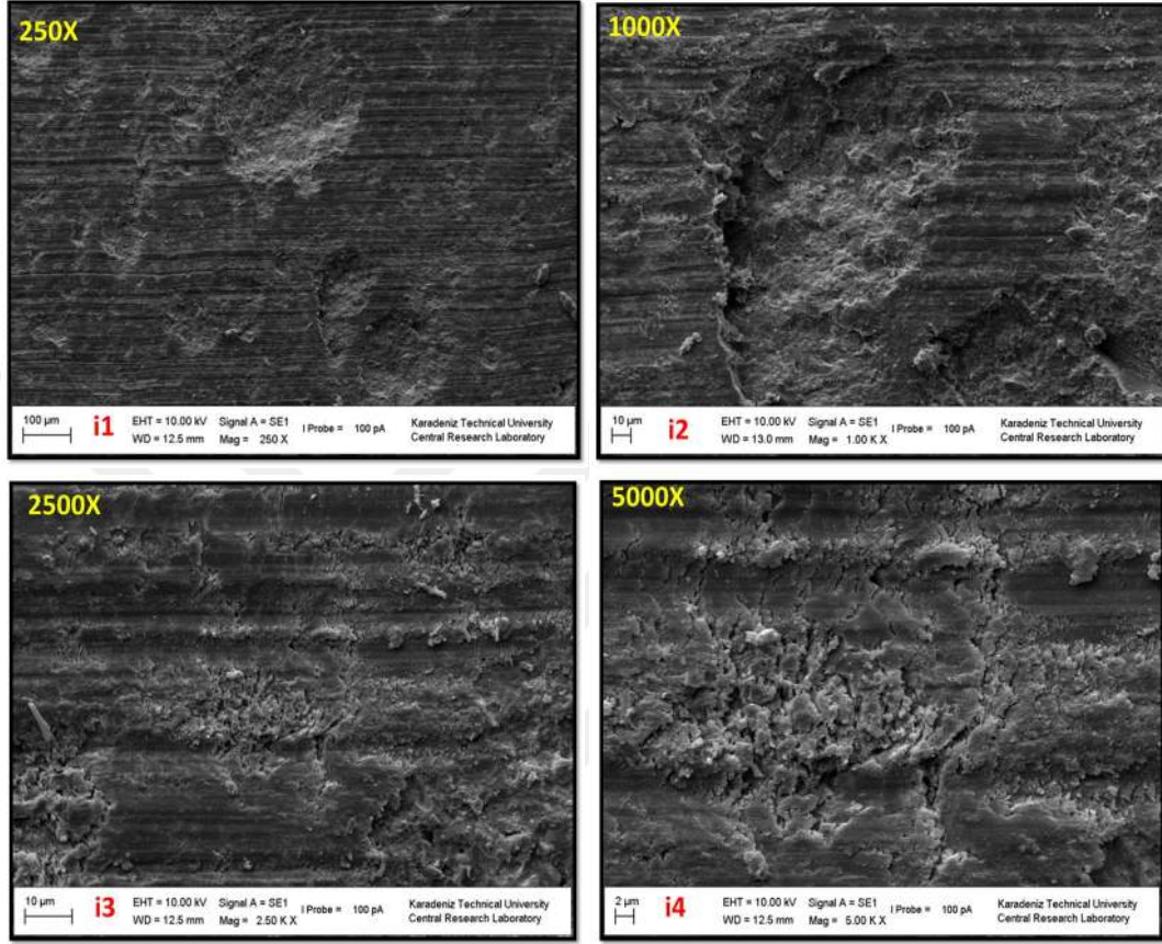
Resim 26. 72 Saat Sertleştirilen MTA'nın SEM Görüntüsü
