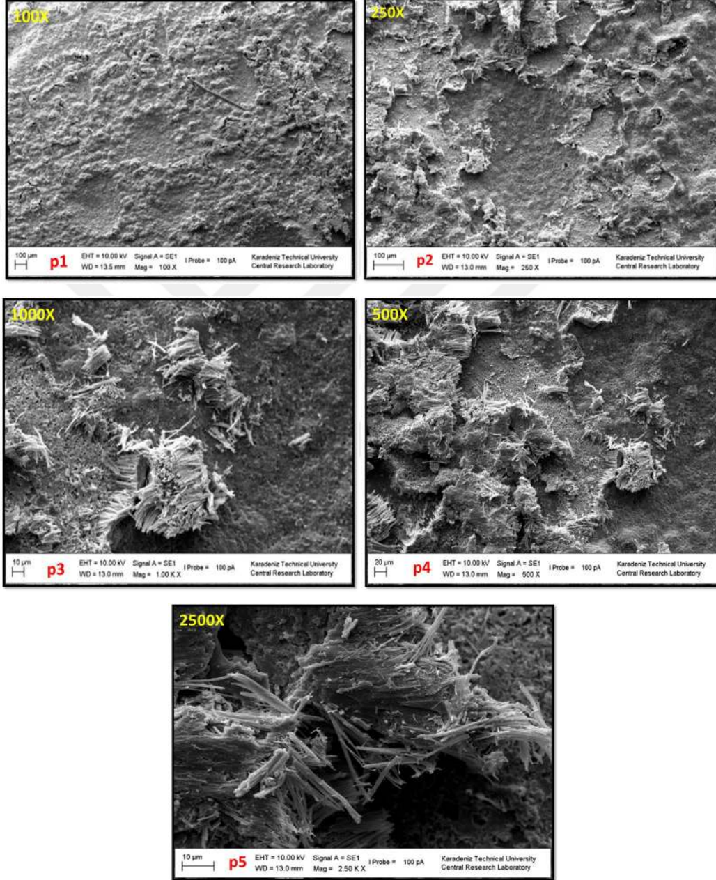
Resim 33. 96 Saat Sertleştirilen MTA'nın Kanla Kontamine Edilmiş Yüzeyine Primer Uygulanmış SEM Görüntüsü
