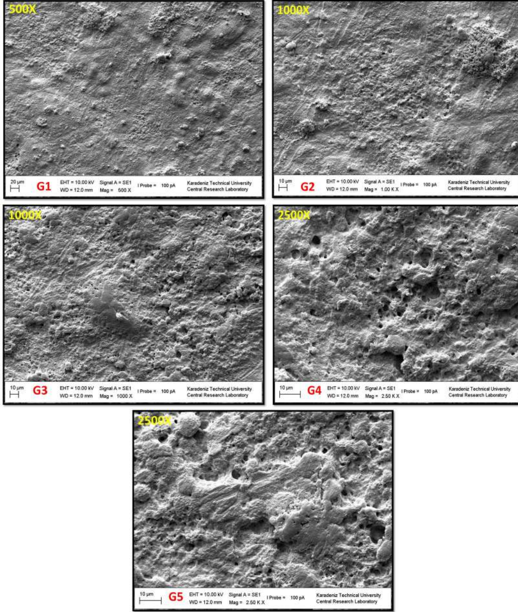
Resim 48. 96 Saat Sertleştirilen Biodentin Yüzeyinin Kanla Kontamine Edilmiş SEM Görüntüsü
