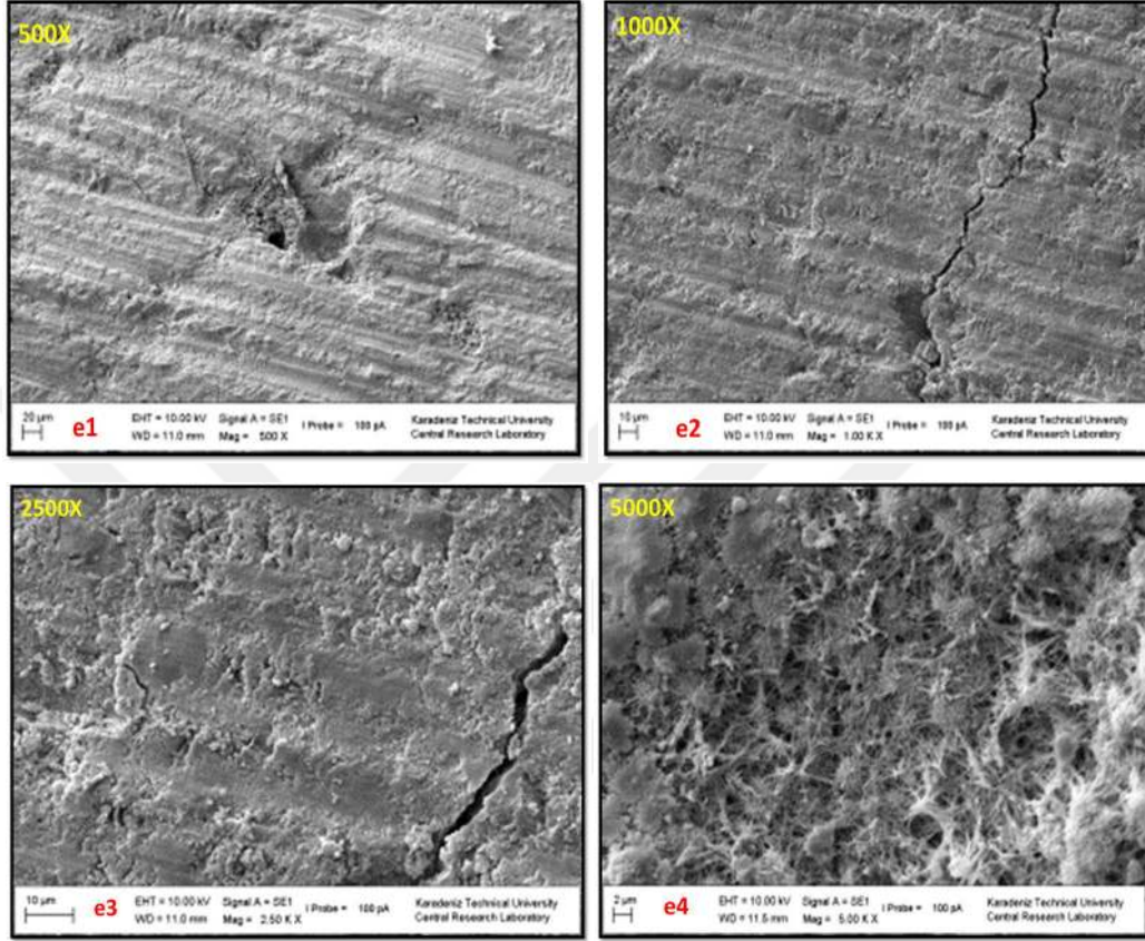
Resim 22. 48 Saat Sertleştirilen MTA Yüzeyinin SEM Görüntüsü
