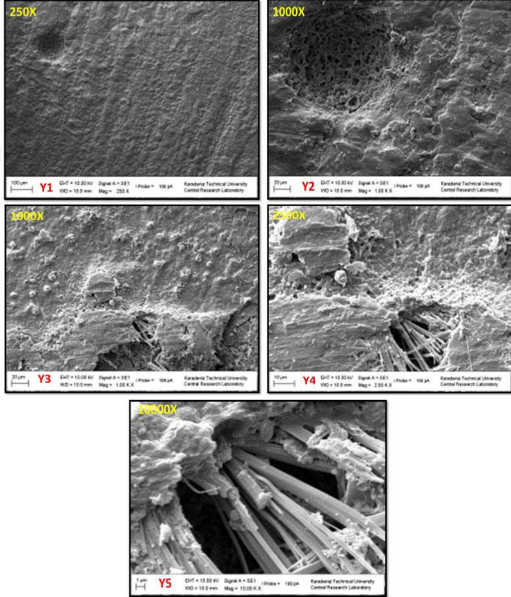
Resim 39. 48 Saat Sertleştirilen Biodentin Yüzeyinin Primer Uygulanmış SEM Görüntüsü
