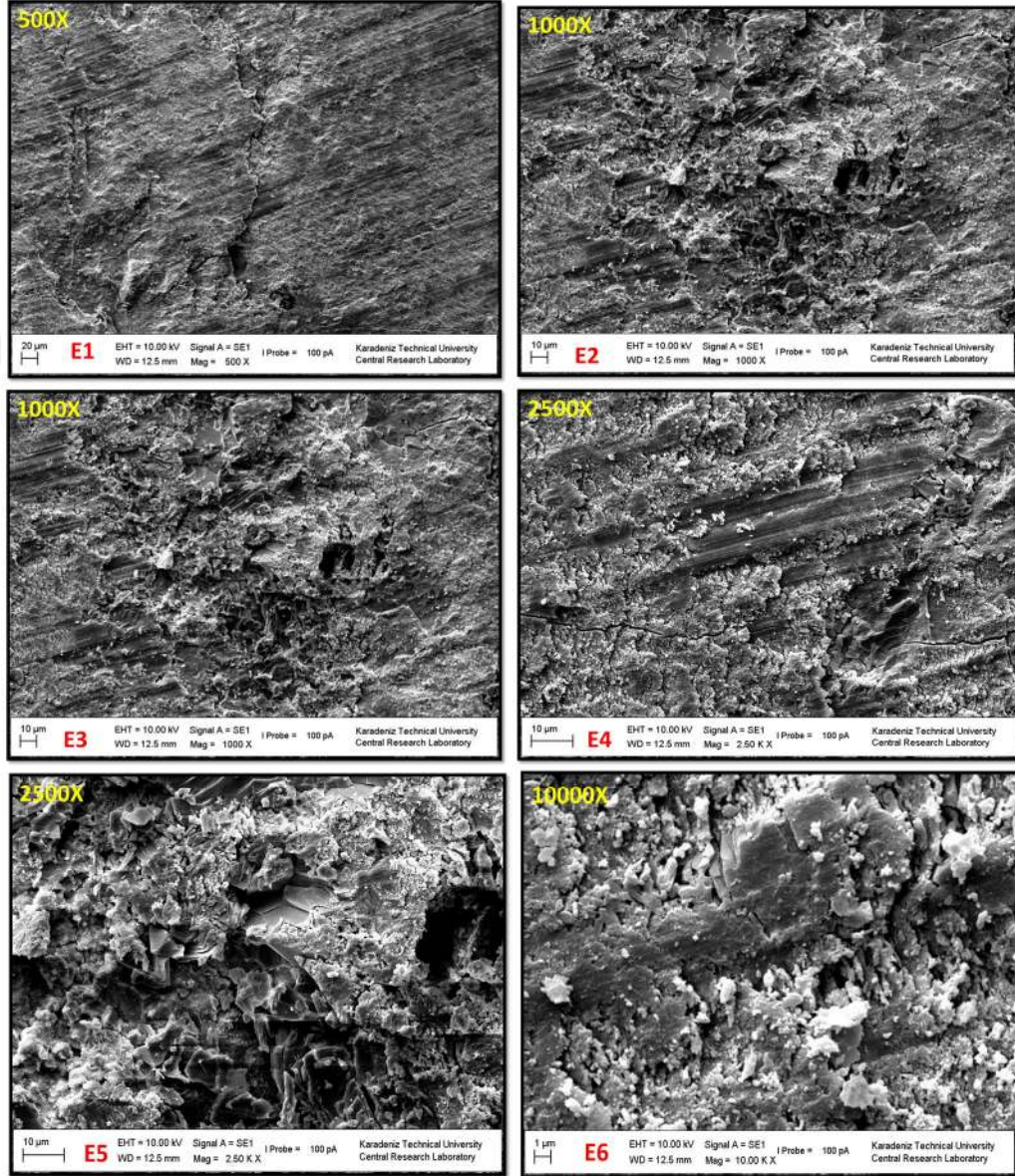
Resim 46. 96 Saat Sertleştirilen Biodentin Yüzeyinin SEM Görüntüsü
