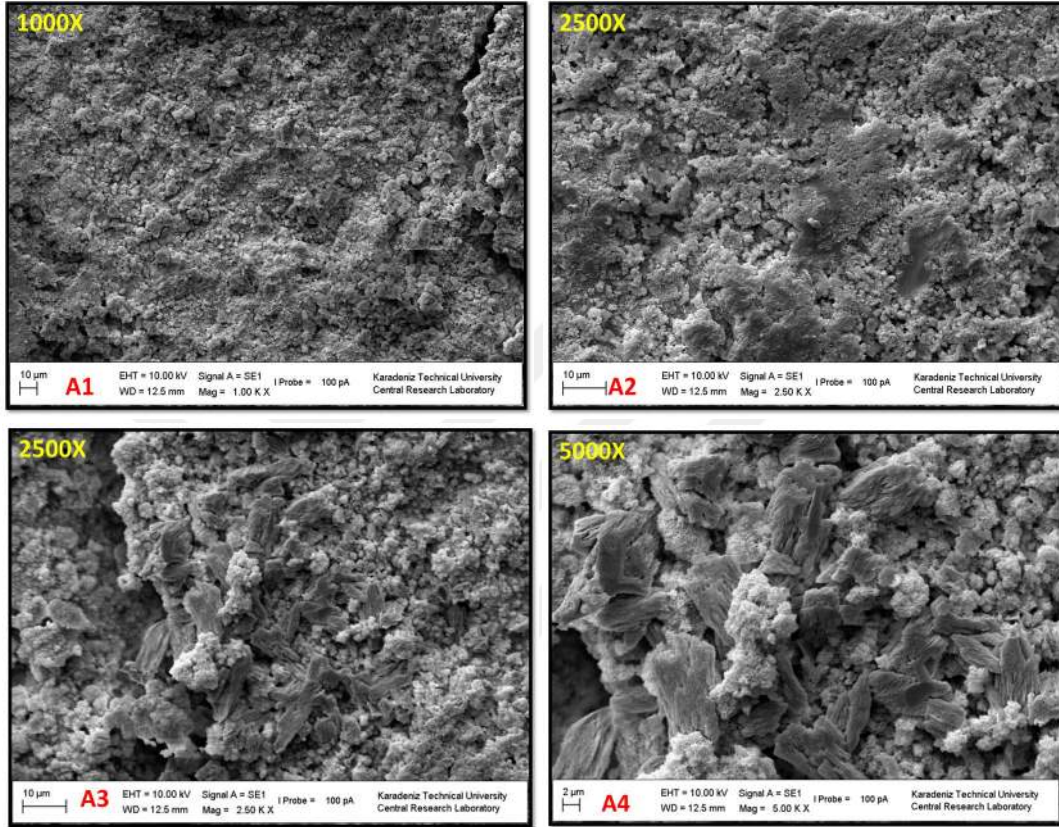
Resim 42. 72 Saat Sertleştirilen Biodentin Yüzeyinin SEM Görüntüsü
