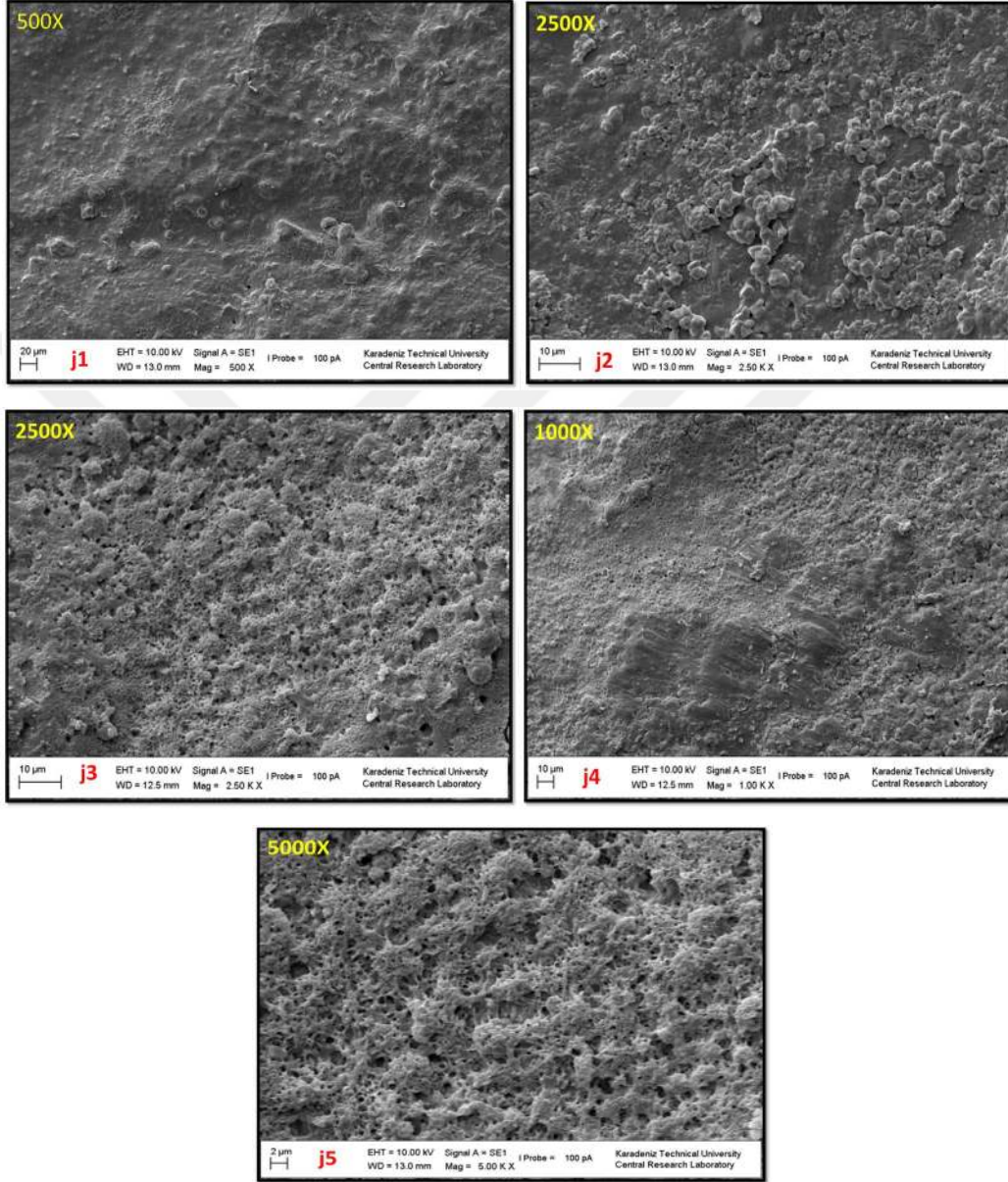
Resim 27. 72 Saat Sertleştirilen MTA Yüzeyinin Primer Uygulanmış SEM Görüntüsü Görüntüsü
