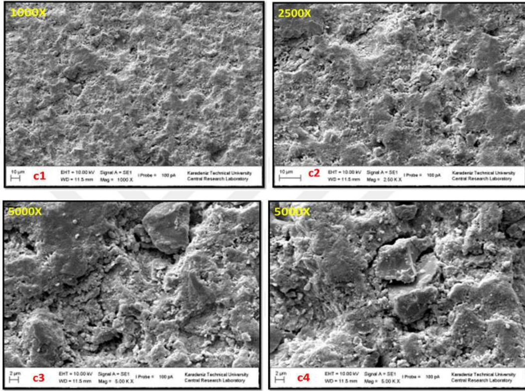
Resim 20. 24 saat sertleştirilen MTA'nın Kanla Kontamine Edilmiş Yüzeyinin SEM Görüntüsü
