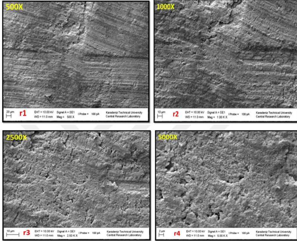
Resim 34. 24 Saat Sertleştirilen Biodentin Yüzeyinin SEM Görüntüsü
