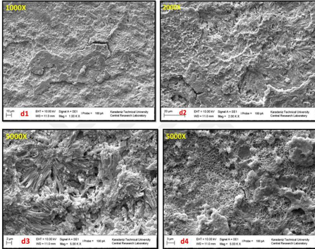
Resim 21. 24 saat sertleştirilen MTA ‘nın Kanla Kontamine Edilip Primer Uygulanmış Yüzeyinin SEM Görüntüsü
