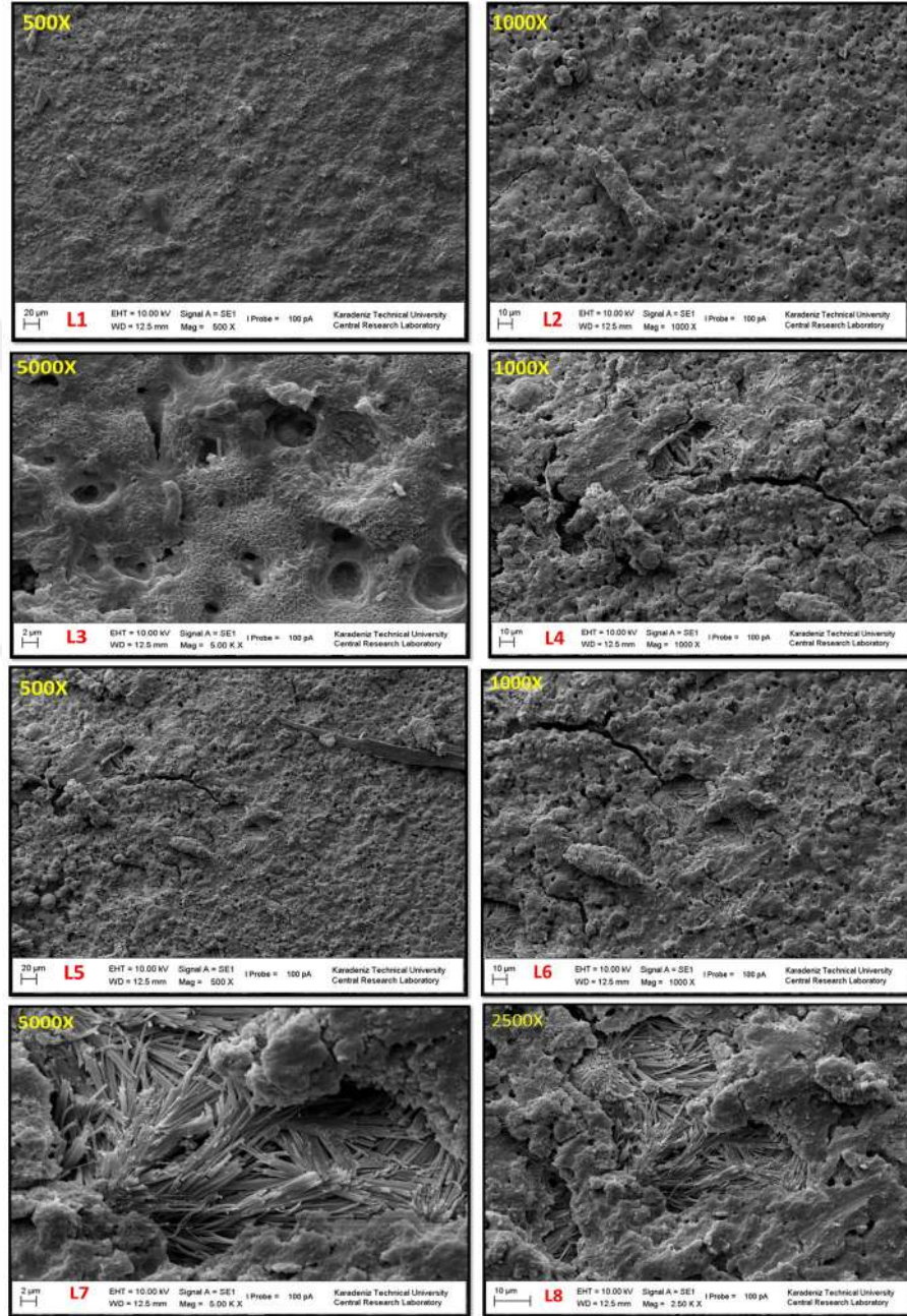
Resim 29. 72 Saat Sertleştirilen MTA Yüzeyinin Kanla Kontamine Edilip Primer Uygulanmış SEM Görüntüsü
