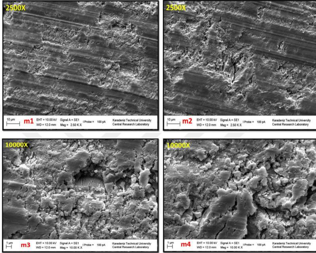
Resim 30. 96 Saat Sertleştirilmiş MTA'nın yüzey SEM görüntüsü
