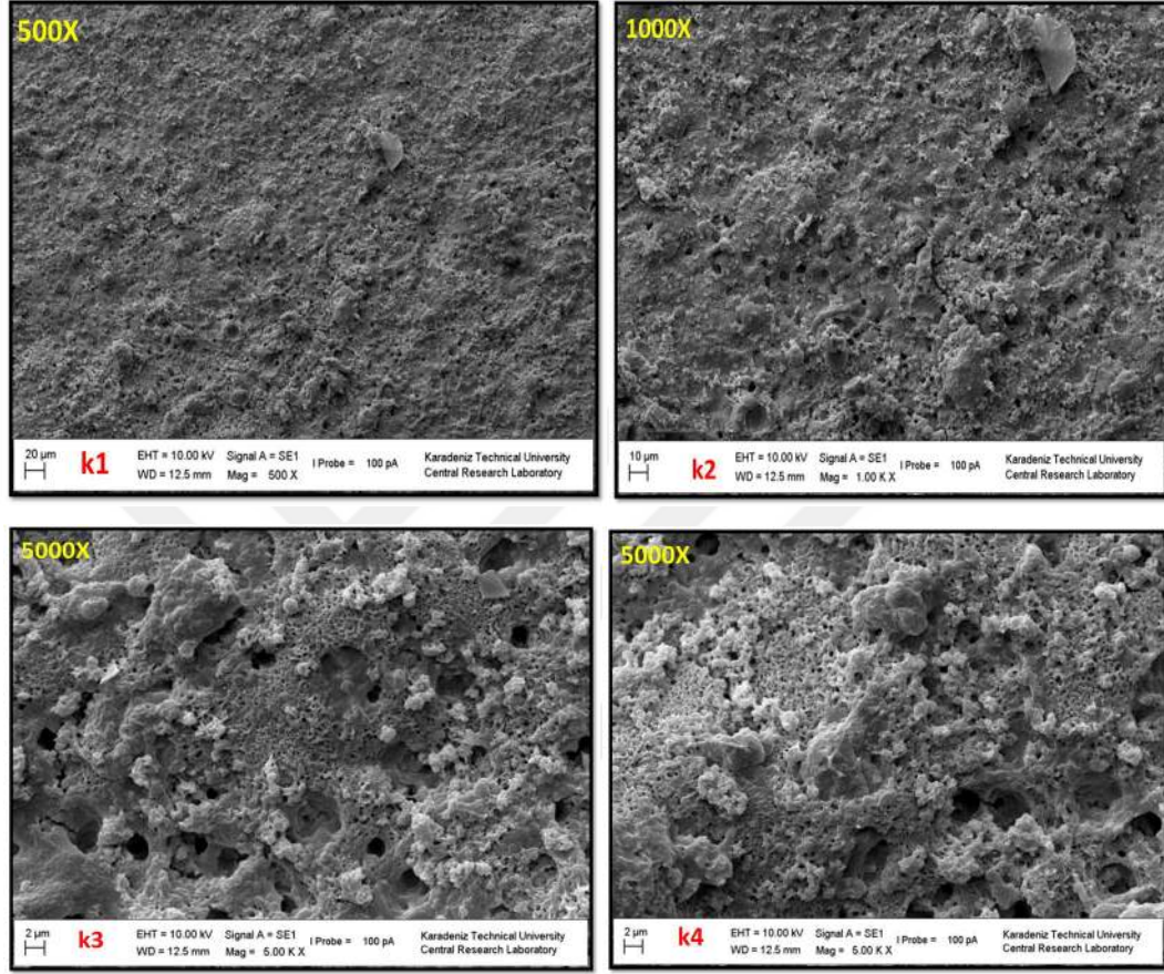
Resim 28. 72 Saat Sertleştirilen MTA Yüzeyinin Kan Uygulanmış SEM Görüntüsü
