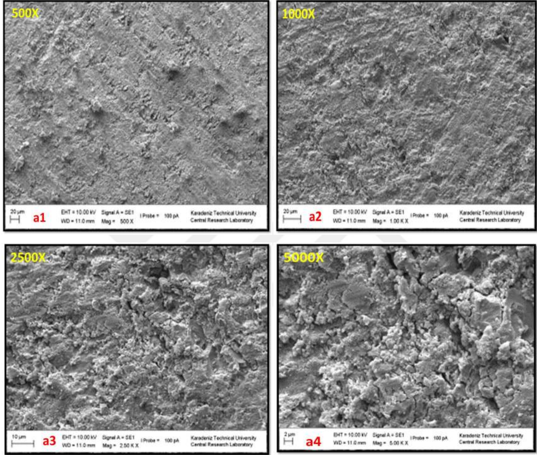
Resim 18. 24 Saat Sertleştirilen MTA yüzeyinin SEM Görüntüsü
