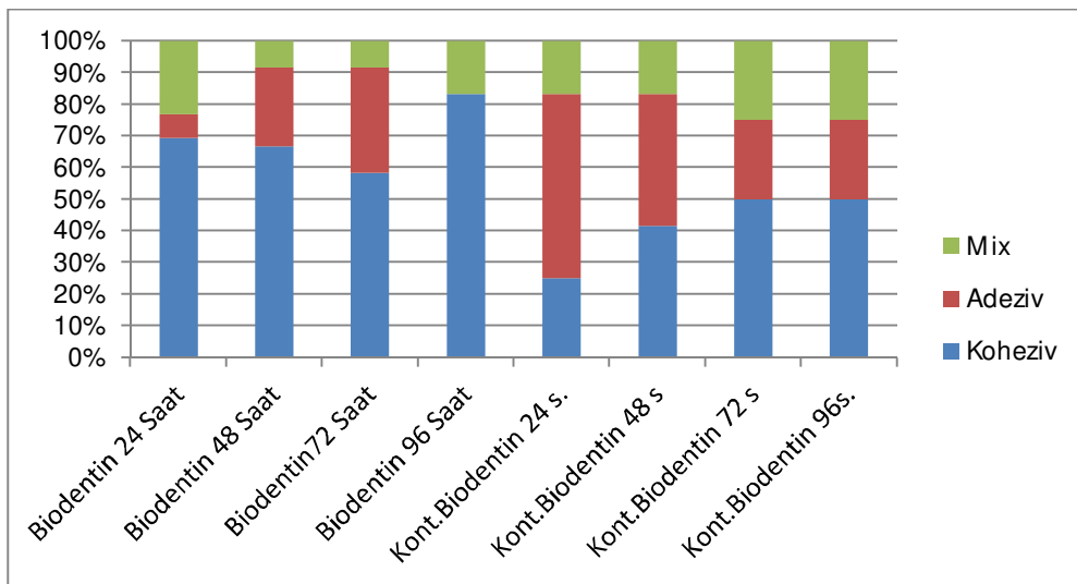
Şekil 3. Biodentin'in farklı sertleşme sürelerinde gözlenen kırılma tiplerinin dağılımı
