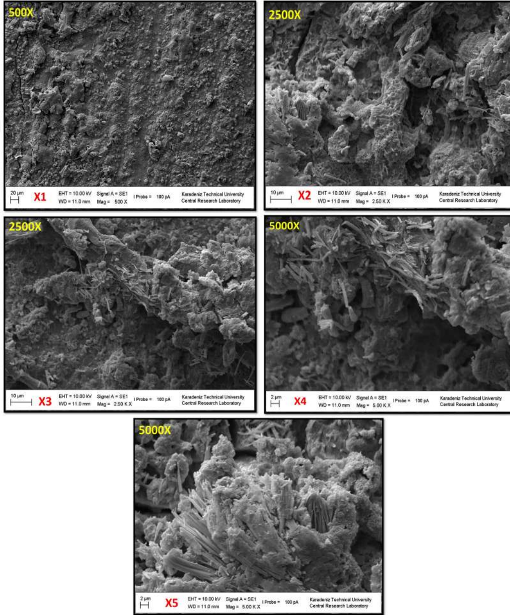
Resim 41. 48 Saat Sertleştirilen Biodentin Yüzeyinin Kanla Kontamine Edilip Primer Uygulanmış SEM Görüntüsü
