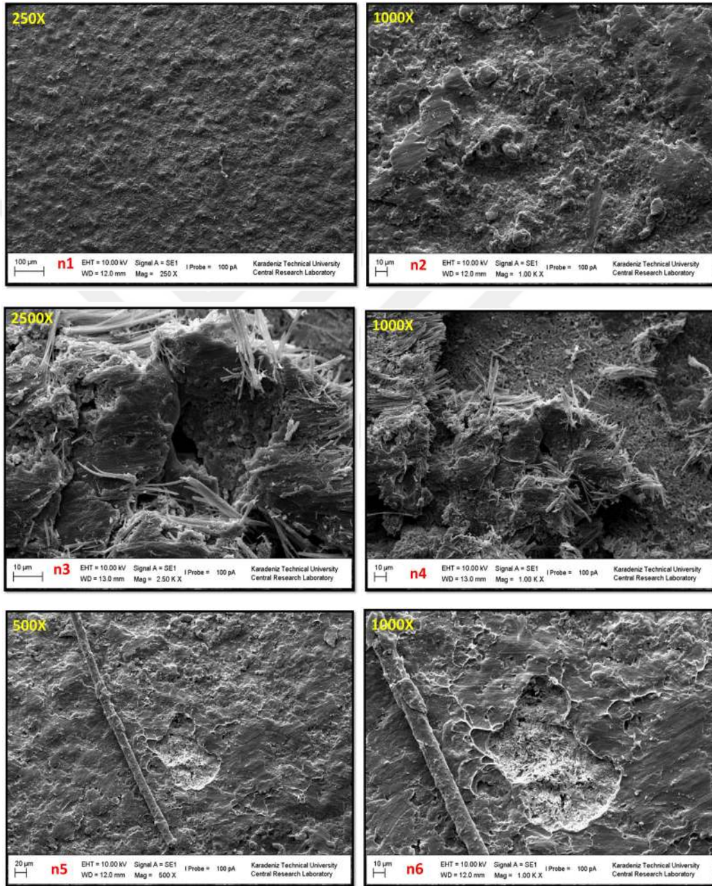
Resim 31. 96 Saat Sertleştirilen MTA'nın Primer Uygulanmış Yüzey Sem Görüntüsü
