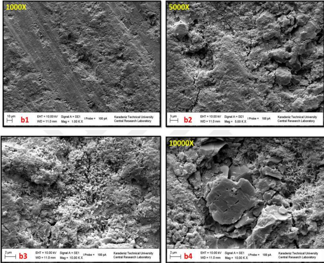
Resim 19. 24 Saat Sertleştirilen MTA'nın Primer uygulanmış yüzeyinin SEM Görüntüsü
