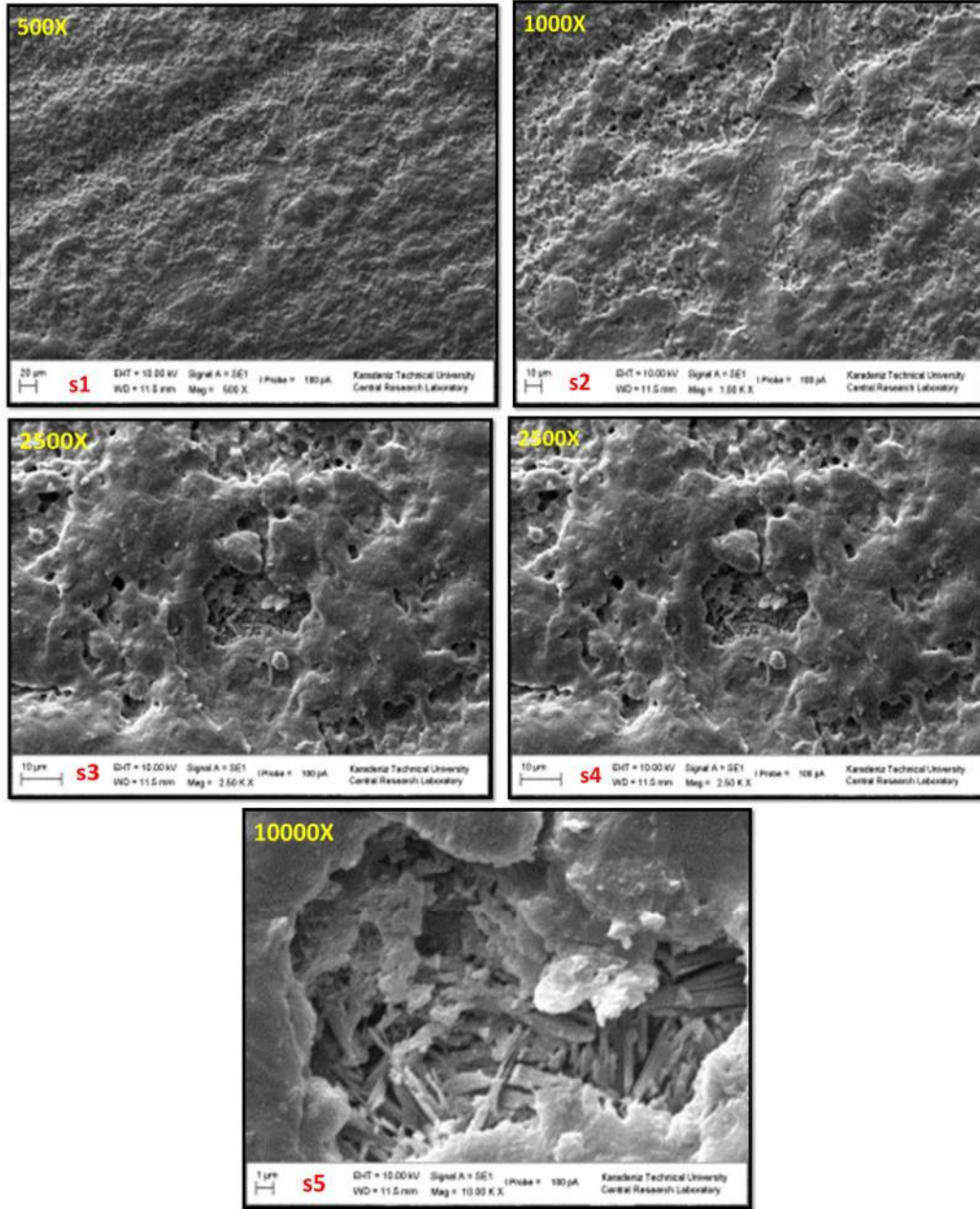
Resim 35. 24 Saat Sertleştirilen Biodentin Yüzeyinin Primer Uygulanmış SEM Görüntüsü
