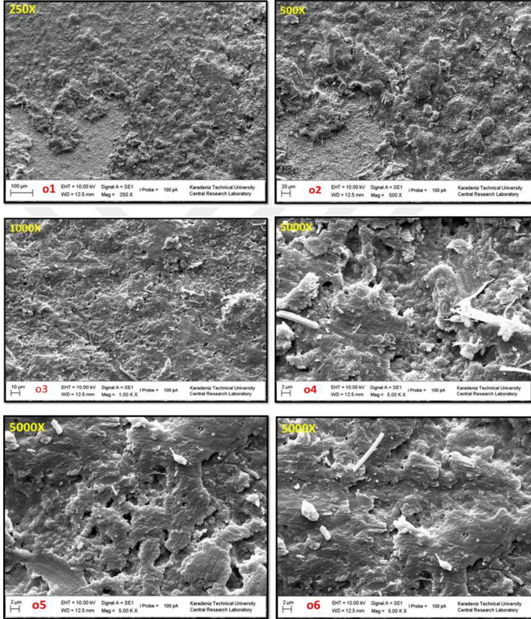
Resim 32. 96 Saat Sertleştirilen MTA'nın Kanla Kontamine Edilmiş Yüzey SEM Görüntüsü
