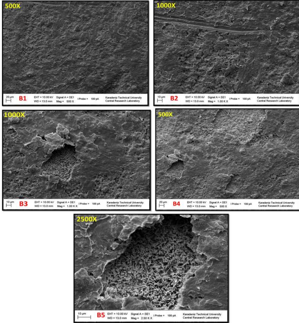
Resim 43. 72 Saat Sertleştirilen Biodentin Yüzeyinin Primer Uygulanmış SEM Görüntüsü
