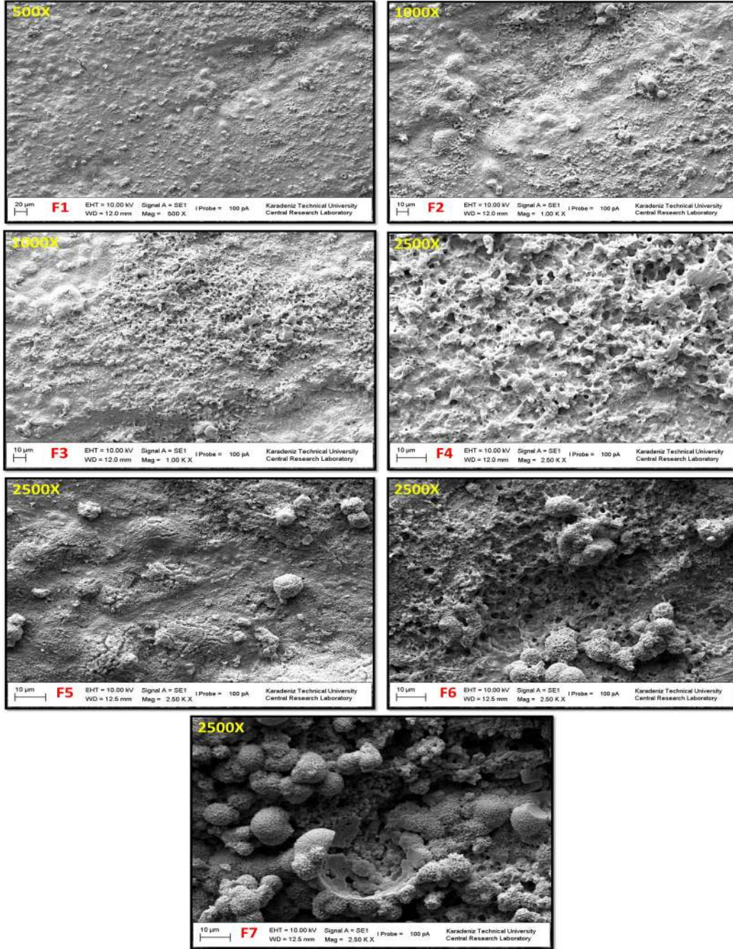
Resim 47. 96 Saat Sertleştirilen Biodentin Yüzeyinin Primer Uygulanmış SEM Görüntüsü
