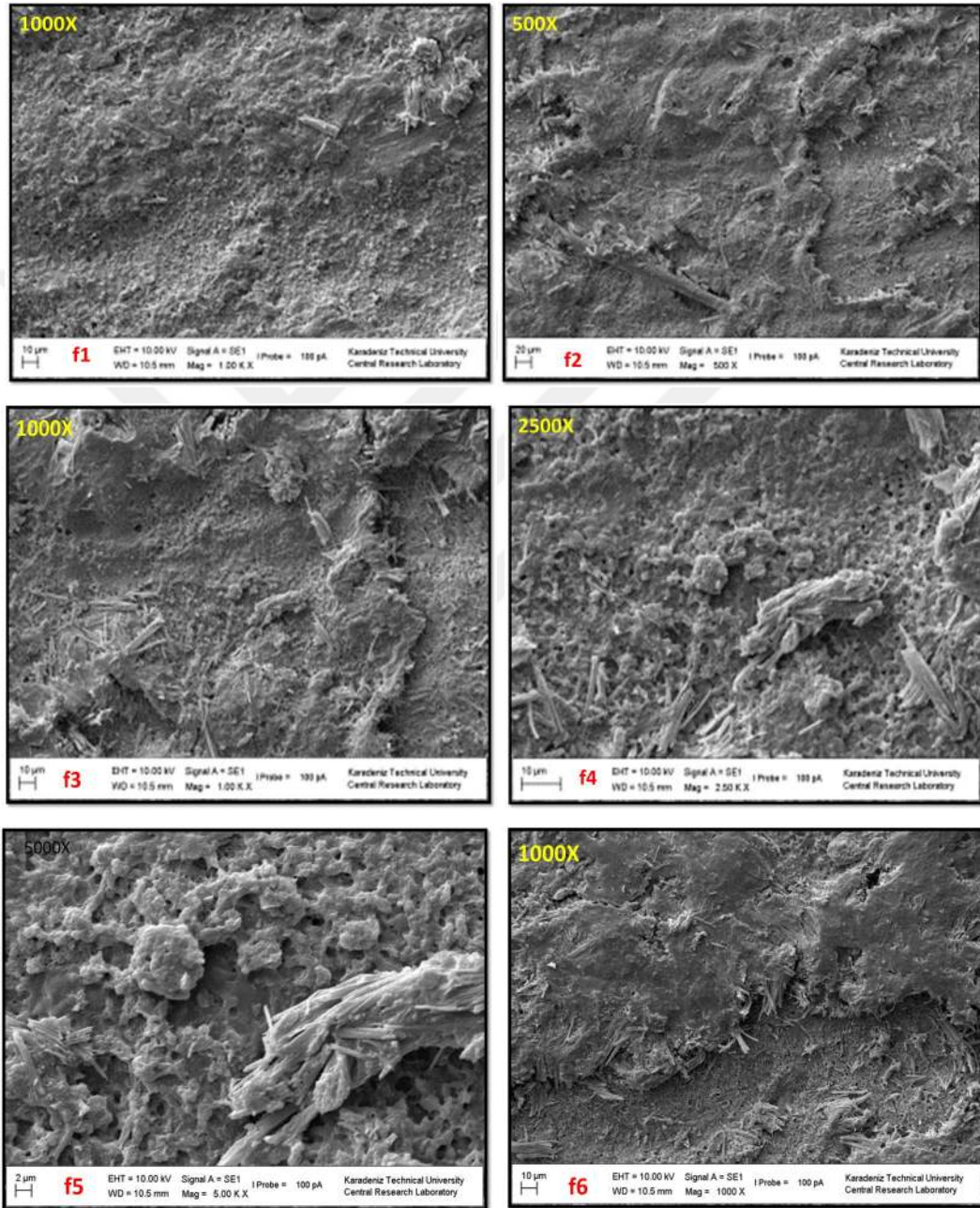
Resim 23. 48 Saat Sertleştirilen MTA Yüzeyinin Primer Uygulanmış Sem Görüntüsü
