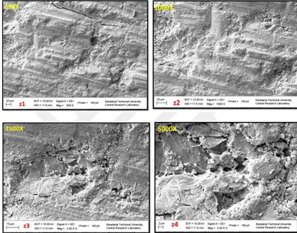
Resim 40. 48 Saat Serleştirilen Biodentin Yüzeyinin Kanla kontamine Edilmiş SEM Görüntüsü
