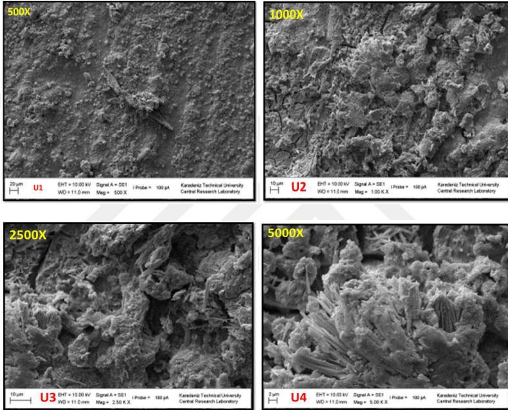
Resim 37. 24 Saat Sertleştirilen Biodentin Yüzeyinin Kanla Kontamine Edilip Primer Uygulanmış SEM görüntüsü
