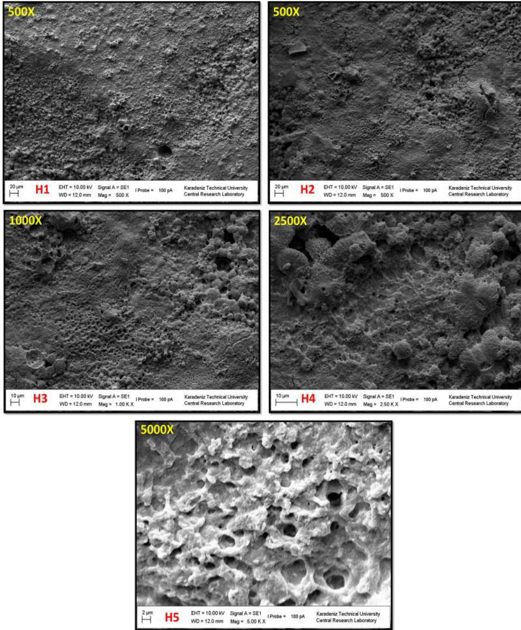
Resim 49. 96 Saat Sertleştirilen Biodentin Yüzeyinin Kanla Kontamine Edilip Primer Uygulanmış SEM Görüntüsü
