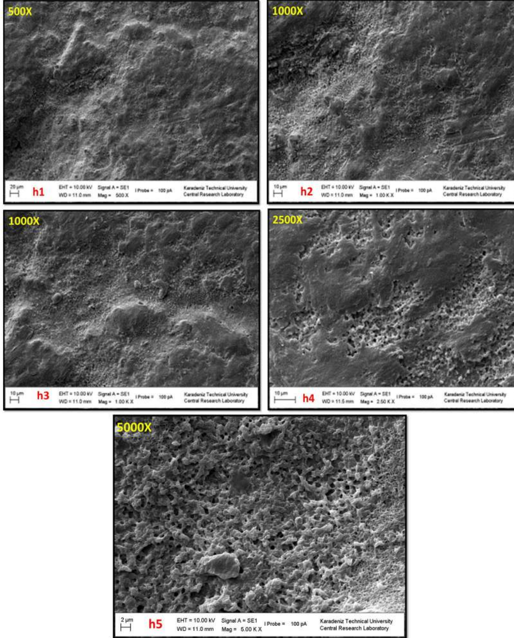
Resim 25. 48 Saat Sertleştirilen MTA Yüzeyinin Kanla Kontamine Edilip Primer Uygulanmış Sem Görüntüsü
