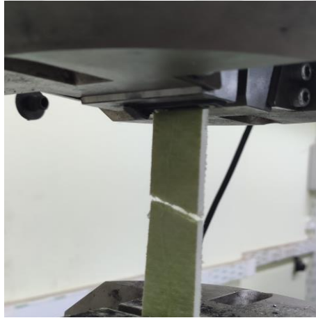
Şekil 4.8 \pm 45^\circ KETP kompozitin çekme deneyi
