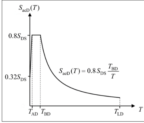
Şekil 4.4. TB DY-2018'e göre düşey elastik tasarım spektrumu grafiği
