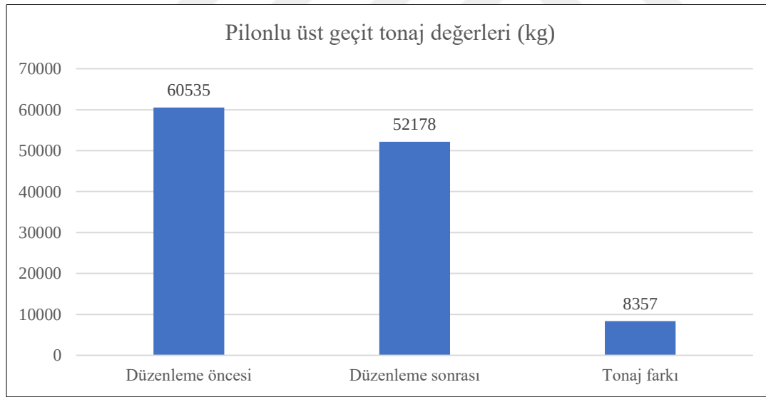
Şekil 5.79. Pilonlu üst geçit için tonaj değerleri
