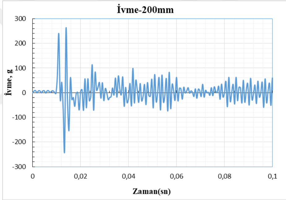
Şekil 4.3. 200 mm yüksekliğinden çekicin numunede oluşturduğu ait ivme-zaman grafiği
