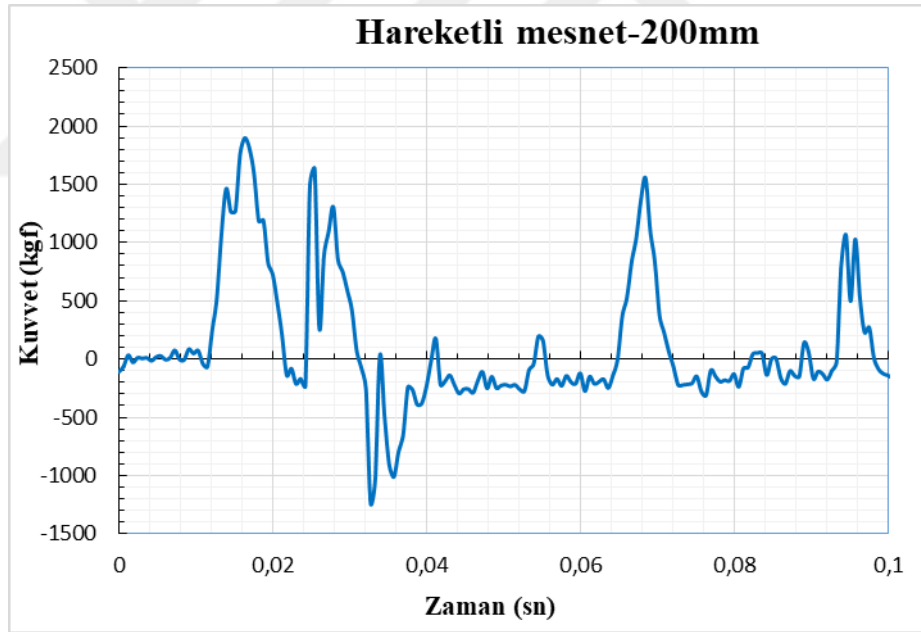
Şekil 4.7. 200 mm yüksekliğinden atılan çekicinin hareketli mesnette oluşturduğu kuvvet-zaman grafiği
