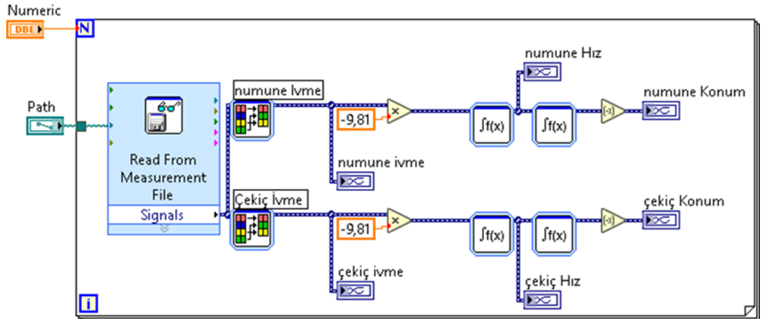
Şekil 3.22. LabVIEW Yazılımı Veri İşleme Algoritması
