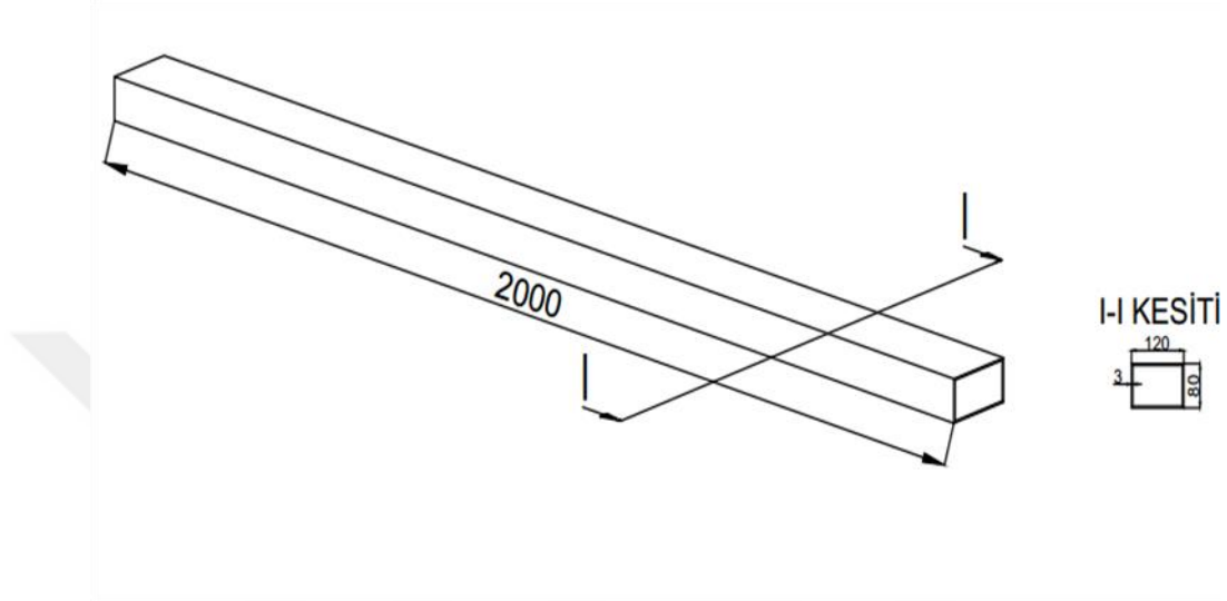
Şekil 3.5. Deneysel çalışmada kullanılan kutu profil tasarımı
