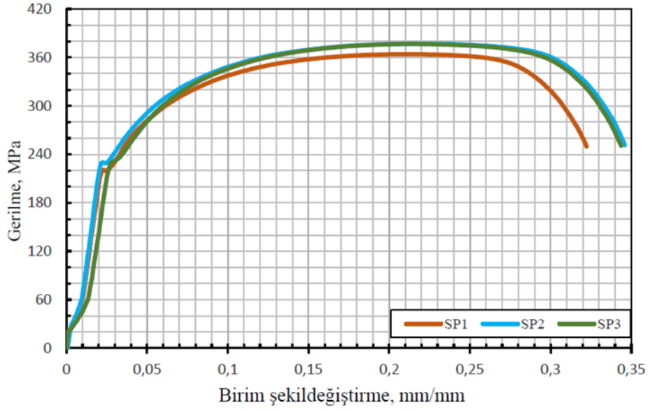
Şekil 3.3. Kupon numunelerine ait gerilme–birim şekil değiştirme grafiği
