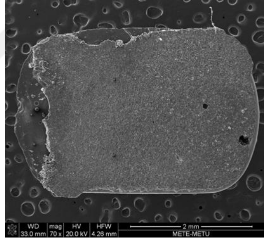
Şekil 4.6. Feldspatık porselen Al 2 O 3 grubu buton vkaidesi SEM görüntüsü
