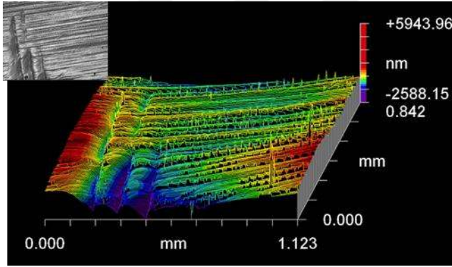
P: Monolitik zirkon elmas frez grubuna ait 3 boyutlu interferogram ve SEM görüntüsü
