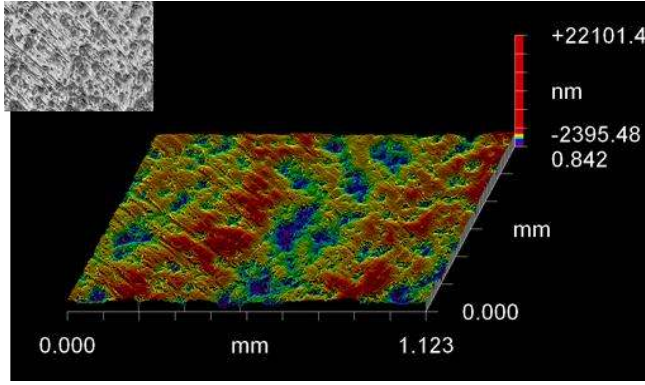
N: Monolitik zirkon \text{Al}_2\text{O}_3 grubuna ait 3 boyutlu interferogram ve SEM görüntüsü
