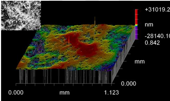
I: Feldpatik porselen \text{Al}_2\text{O}_3 grubuna ait 3 boyutlu interferogram ve SEM görüntüsü
