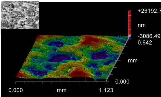
K: Feldspatik porselen elmas frez grubuna ait 3 boyutlu interferogram ve SEM görüntüsü
