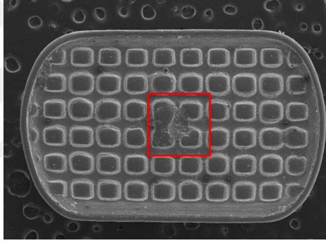
Şekil 3.14. Hesaplamalarda kullanılacak buton kaidesinin SEM görüntüsü
