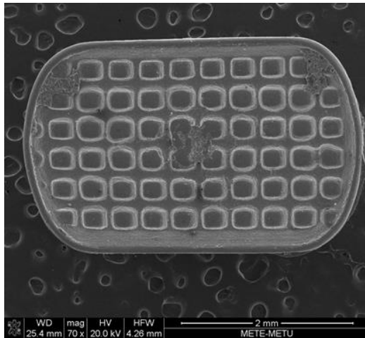
Şekil 4.1. Enamic elmas frez grubu buton kaidesi SEM görüntüsü
