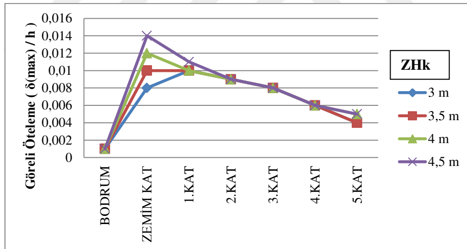
Şekil 3.12. 5 katlı referans sistemde görelî ötelemelerin katlara göre değişimi
