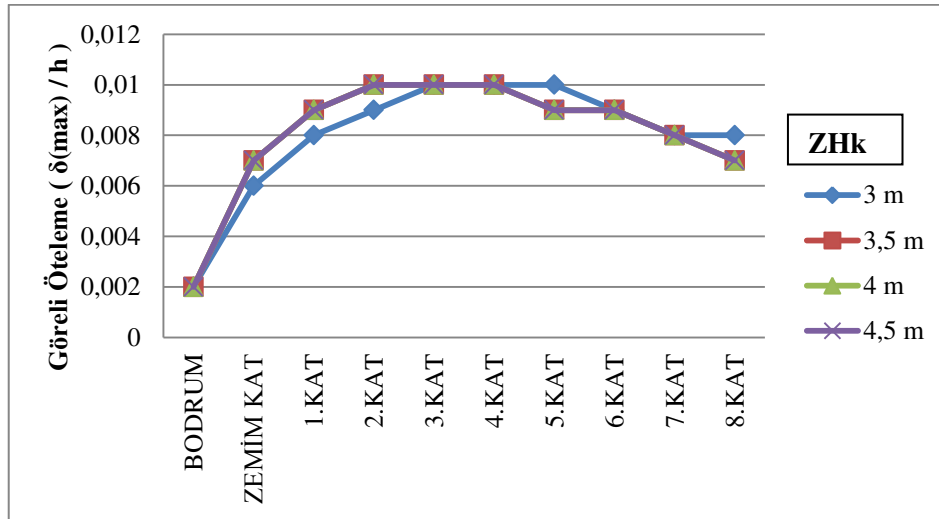
Şekil 3.14. 8 katlı referans sistemde görelî ötelemelerin katlara göre değışimi
