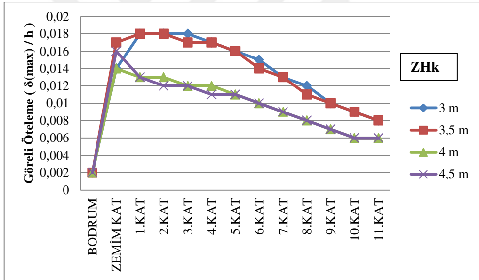
Şekil 3.17. 11 katlı numune sistemde görelî ötelemelerin katlara göre değişimi
