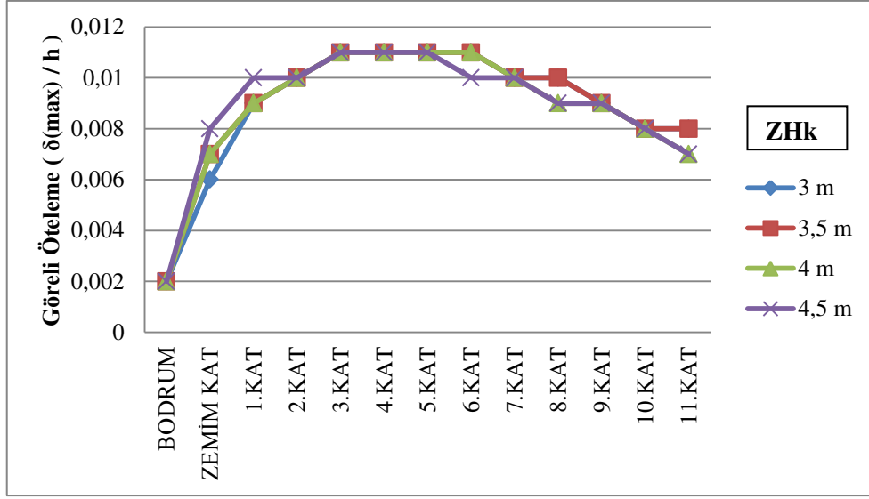
Şekil 3.16. 11 katlı referans sistemde görelî ötelemelerin katlara göre değişimi
