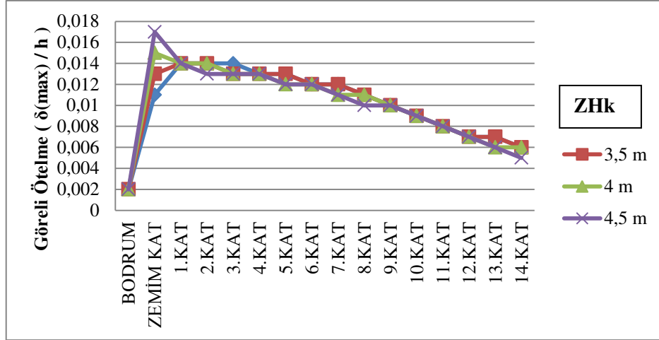
Şekil 3.19. 14 katlı numune sistemde görelî ötelemelerin katlara göre değişimi
