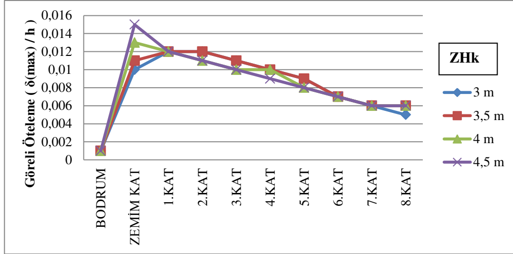
Şekil 3.15. 8 katlı numune sistemde görelî ötelemelerin katlara göre değişimi
