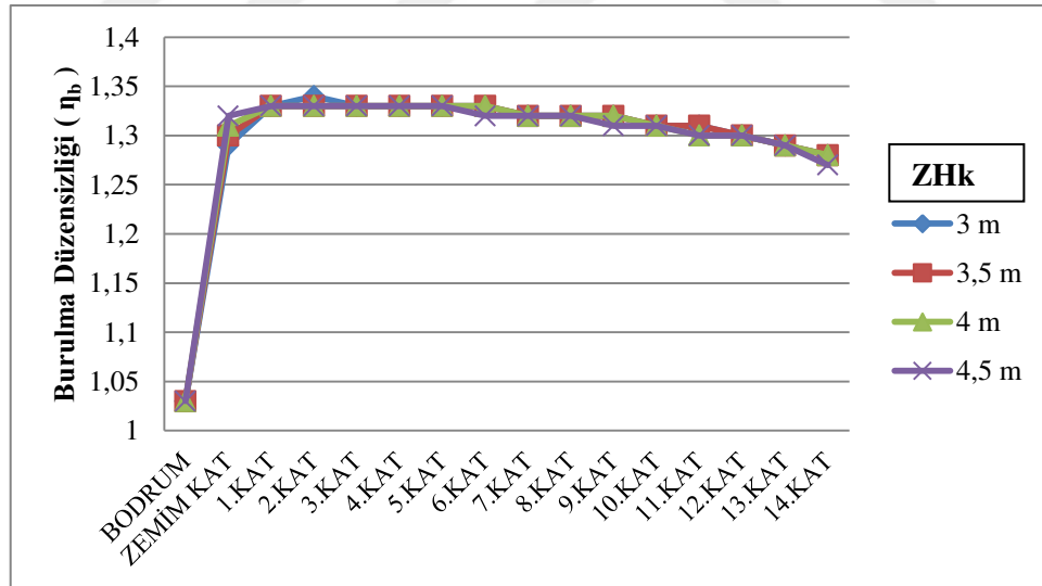
Şekil 3.9. 14 katlı referans sistemde burulma düzensizliğinin zemin kat yüksekliğine göre değişimi
