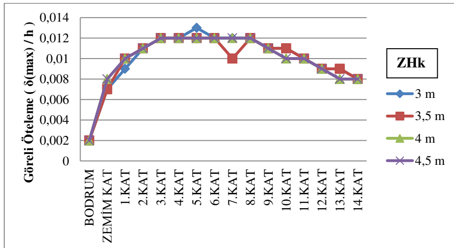
Şekil 3.18. 14 katlı referans sistemde görelî ötelemelerin katlara göre değışimi
