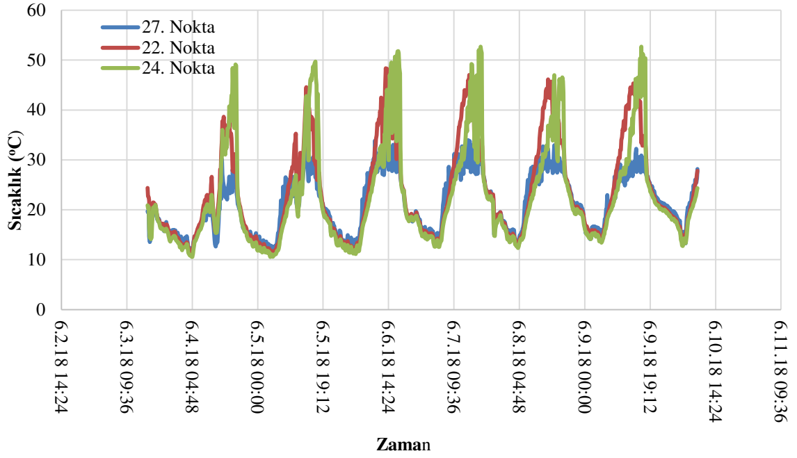
Şekil 3.3. Dış ortamda konumlandırılmış ısı çiftleri değerlendirilmesi
