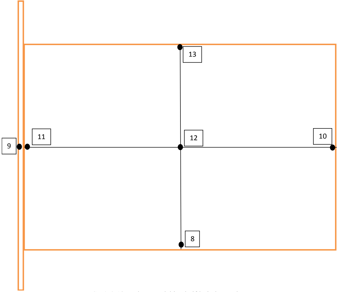
Şekil 2.18. Isı borusundaki ısı çiftlerinin konumları
