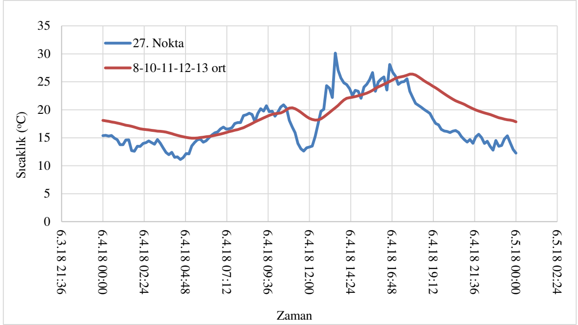
Şekil 3.6. Çevre sıcaklığının ısı borusun daki ısı çiftlerle iki günlük karşılaştırılması
