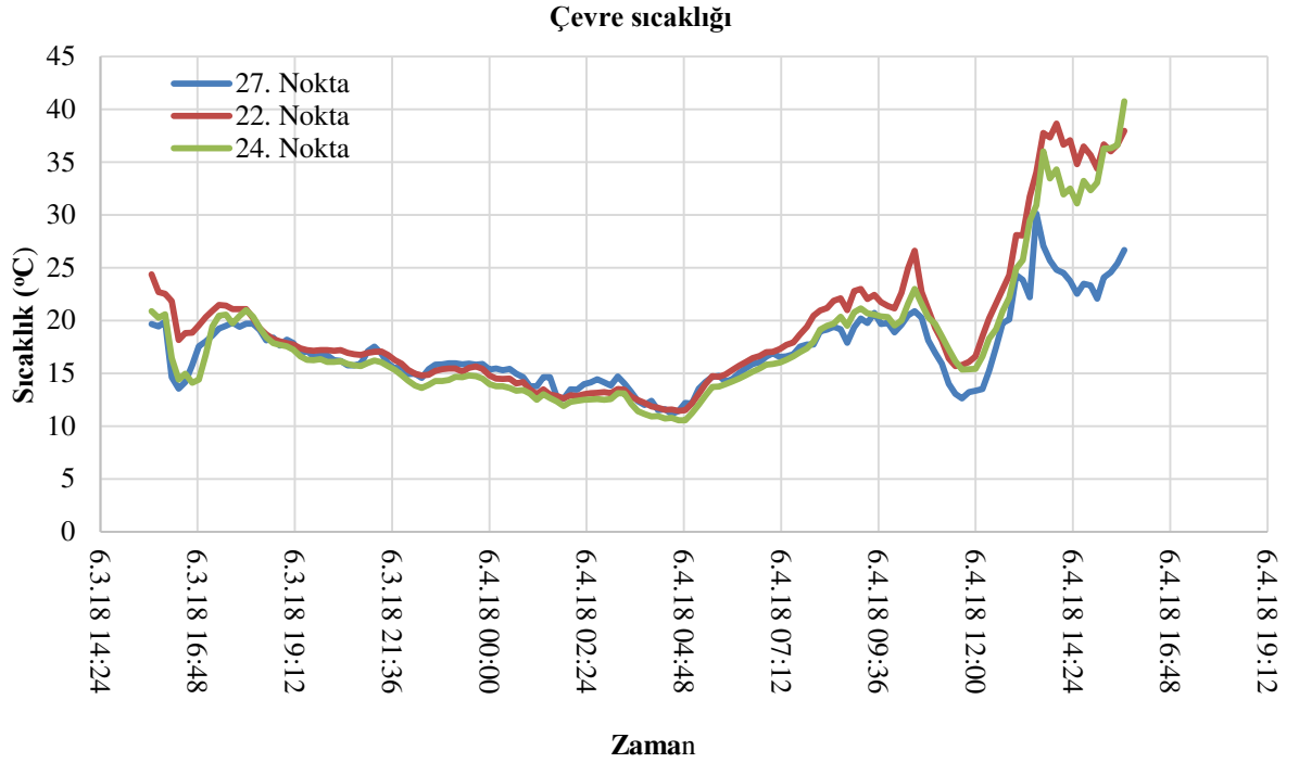
Şekil 3.4. Konteynerin ön, yan ve çevre sıcaklığının bir günlük karşılaştırılması
