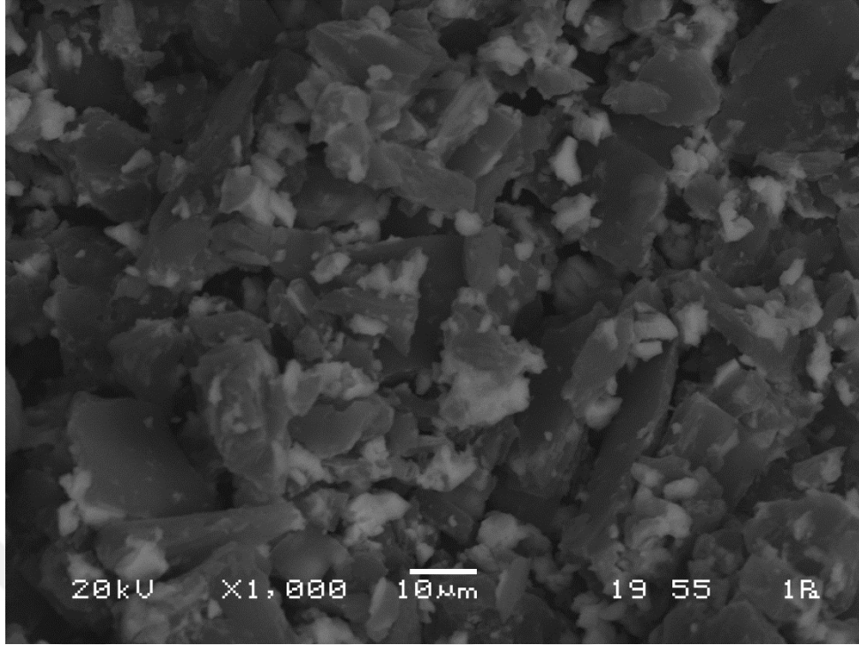
Şekil 6.6. Arsenik adsorpsiyonu sonrası \text{Fe}_3\text{O}_4\text{-TAK-As} ait SEM görüntüleri (10 \mu\text{m} ).
