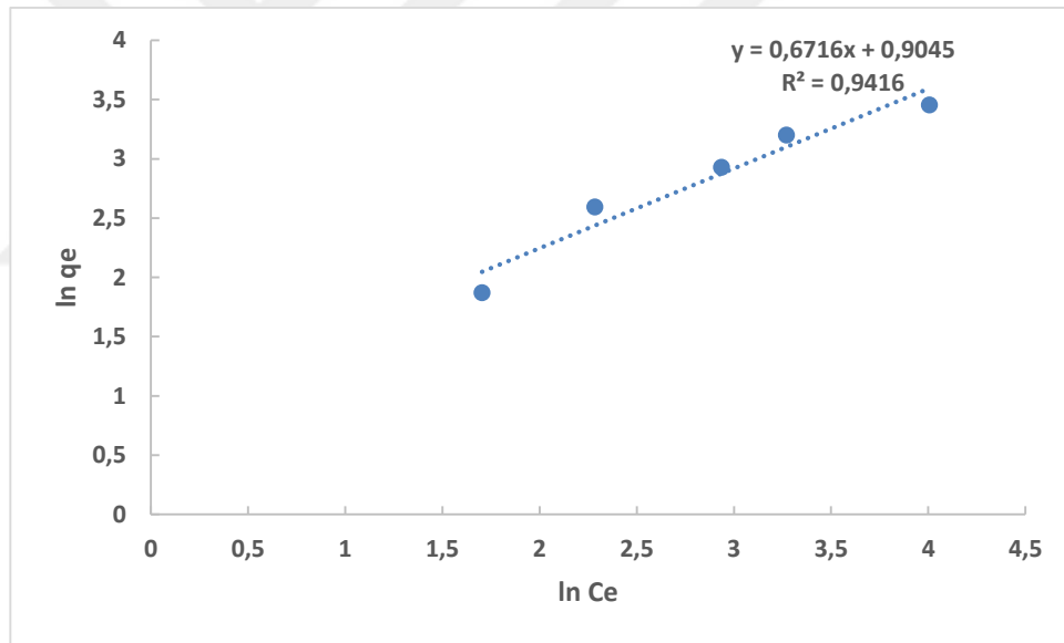
Şekil 6.20. Fe 3 O 4 -TAK sorbenti üzerine Arsenik adsorpsiyonu için 293K’de elde edilen Freundlich izotermeleri grafiği.
