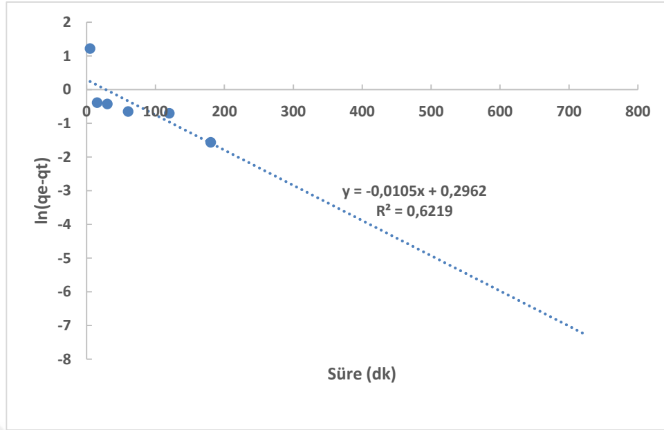
Şekil 6.24. Arseniğin \text{Fe}_3\text{O}_4 -TAK ile adsorpsiyonunun psödo 1. Derece denklem grafiği
