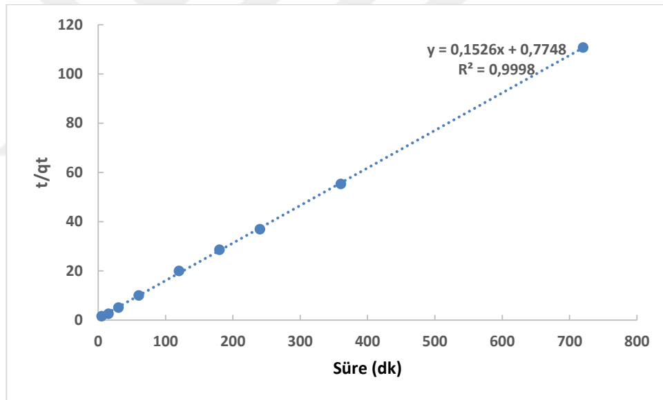
Şekil 6.25. Arseniğin \text{Fe}_3\text{O}_4 -TAK ile adsorpsiyonunun psödo 2. Derece denklem grafiği
