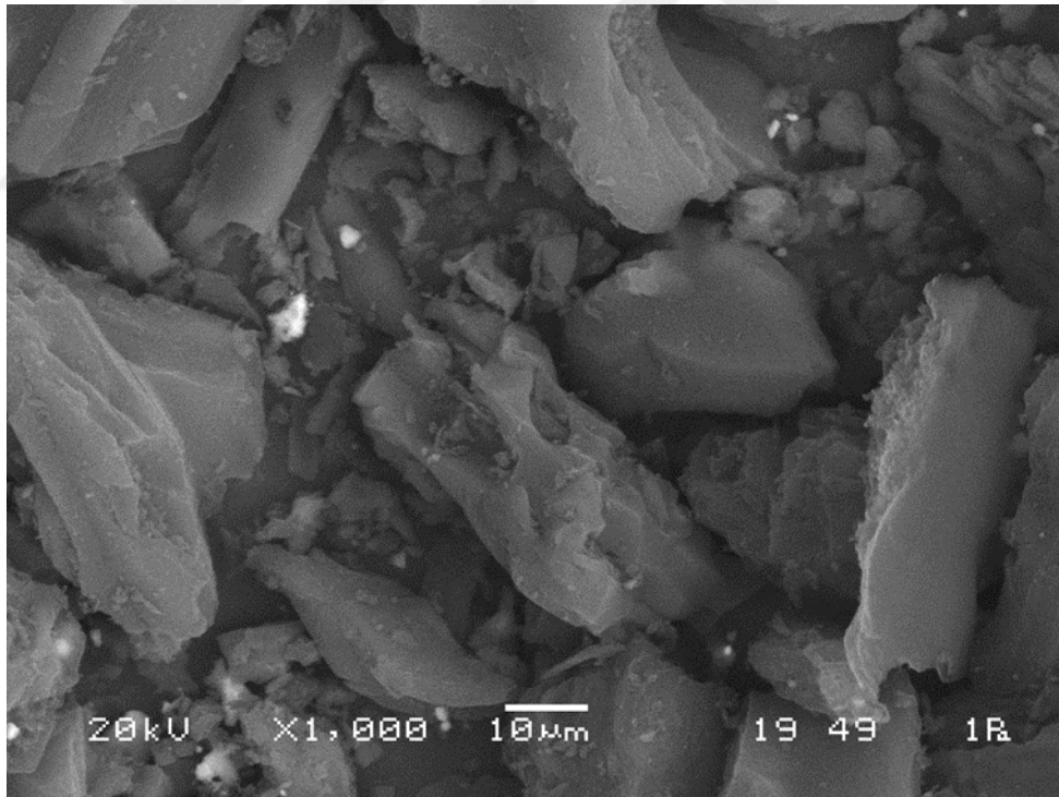
Şekil 6.4. Ticari Aktif karbon (TAK)'na ait SEM görüntüleri (10 \mu\text{m} ).
