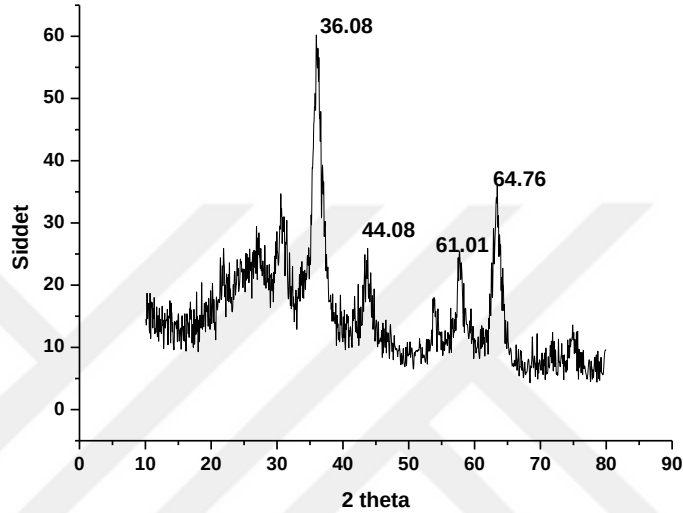
Şekil 6.9. Arsenik Adsorpsiyonu sonrası \text{Fe}_3\text{O}_4 -TAK'nun toz XRD spektrumu
