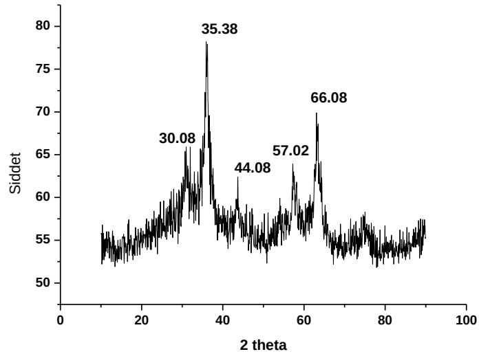
Şekil 6.8. \text{Fe}_3\text{O}_4 -TAK'nin toz XRD spektrumu
