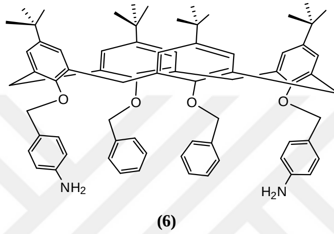
Şekil 3.6 5,11,17,23-ter-bütil-25,27-bis-(4-aminobenziloksi)-26,28-dibenziloksikaliks[4] aren (6)
