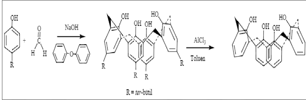
Şekil 2.6 p-ter -bütilkaliks[4]aren ve kaliks[4]aren eldesi
