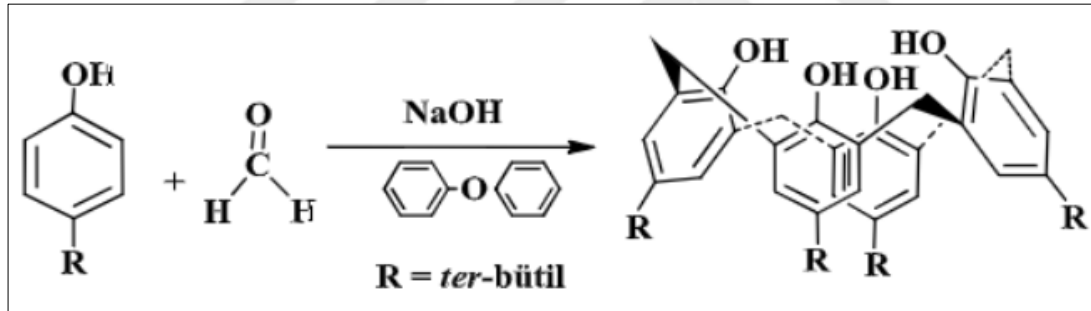
Şekil 2.7 p-ter-bütöl kaliks[4]aren sentezi
