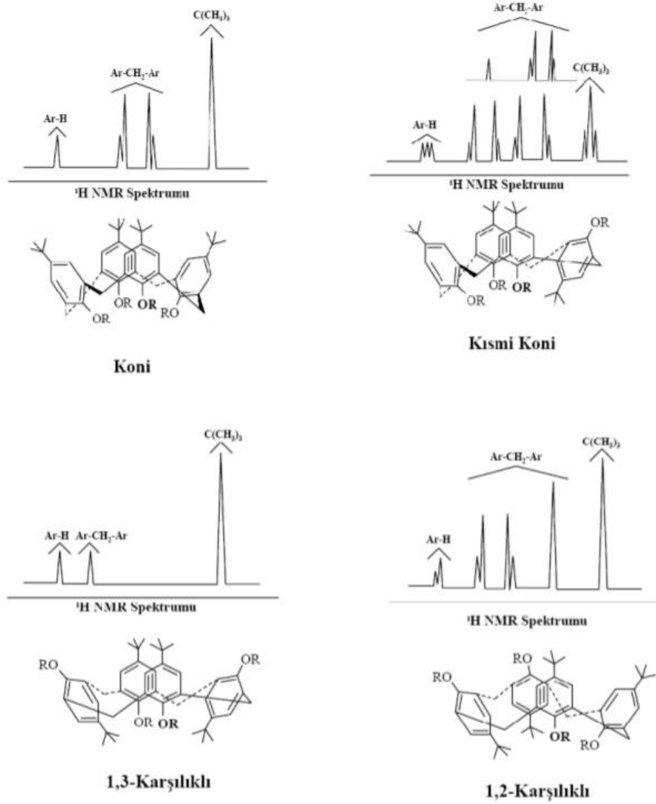
Şekil 2.18 p -ter-bütilkaliks[4]arenin konformasyonları ve 1 H-NMR spektrumları
