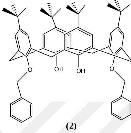
Şekil 3.2 5,11,17,23-tetra-tert-bütil-25,27-bisbenziloksi-26,28-dihidroksikaliks[4]aren (2)
