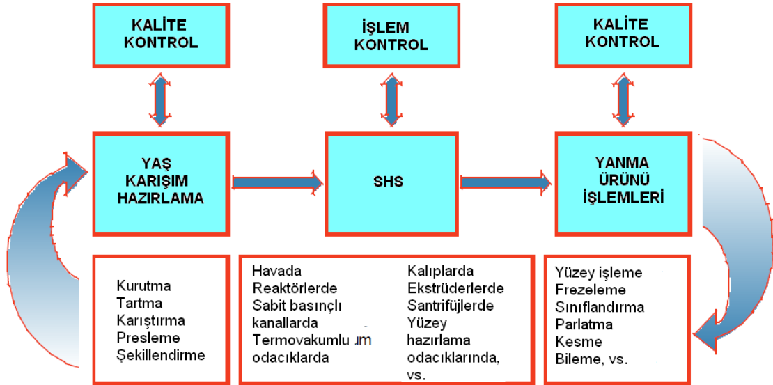
Çizelge 2. 7 SHS işlem şeması [15].
