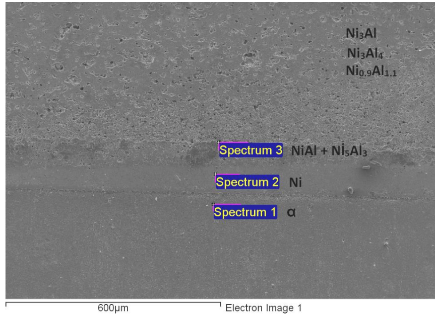
Şekil 4. 10 N3 nolu numunenin SEM ve XRD sonuçları.
