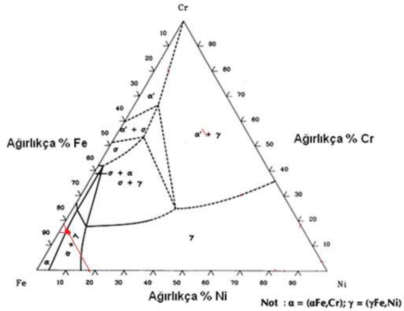
Şekil 4. 13 Fe-Ni-Cr üçlü denge diyagramı (400 °C).
