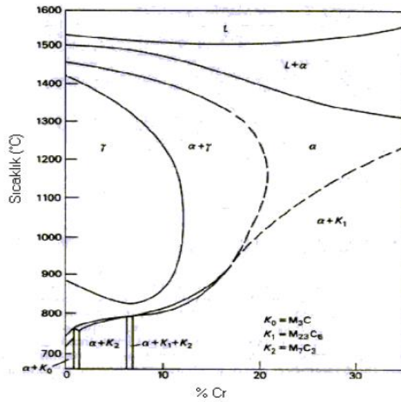
Şekil 2. 11a Fe-Cr diyagramı üzerinde C'un etkisi (% 0,05C) [4].
