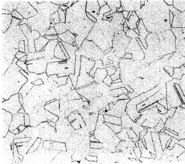
Şekil 2. 12 304 tipi östenitik paslanmaz elik şerit 1060 °C' de 5 dakika tavlandıktan sonra havada soęutulmuş. Yapı eşeksenel östenit tanelerinden oluşmaktadır ve yapıda tavlama ikizleri görölmekte (250X) [4].
