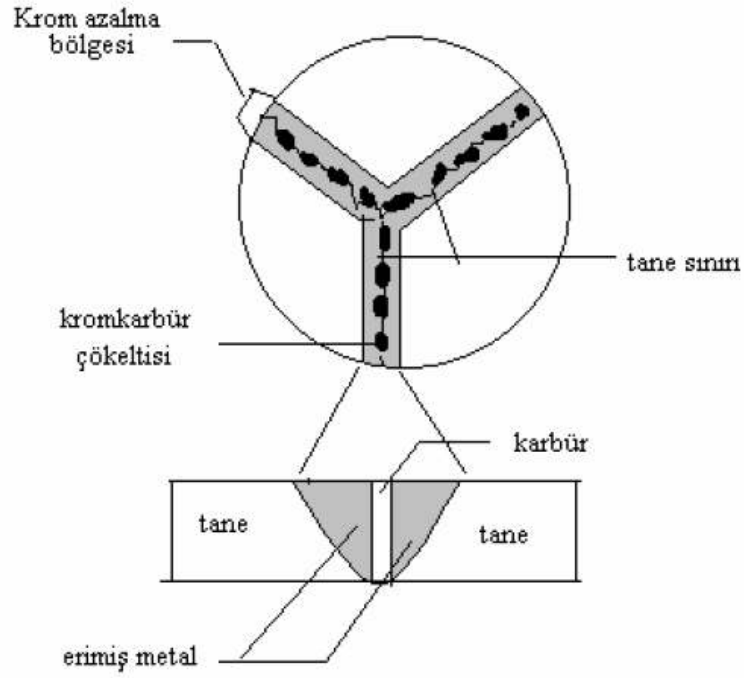
Şekil 2. 16 Paslanmaz çelikte tanelerarası korozyona duyarlaşma sırasında tane sınırındakarbür çökelmesinin şematik olarak görünümü [13].
