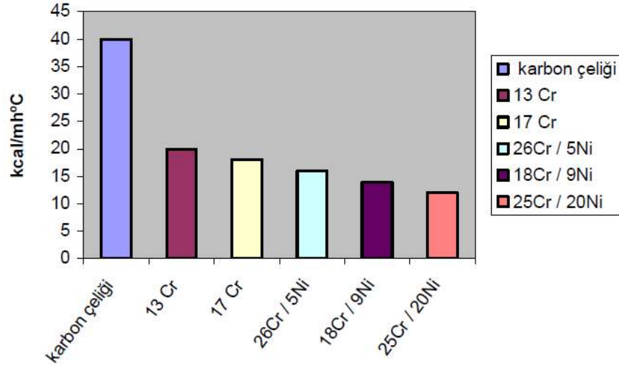
Şekil 2. 1 20-100 °C’de Çeşitli paslanmaz çelikler ile karbonlu çeliğin ısı iletim kabiliyetleri [2,3].
