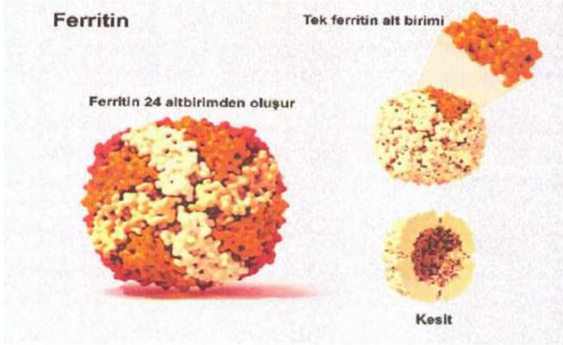
Şekil 2.4. Ferritinin yapısı
