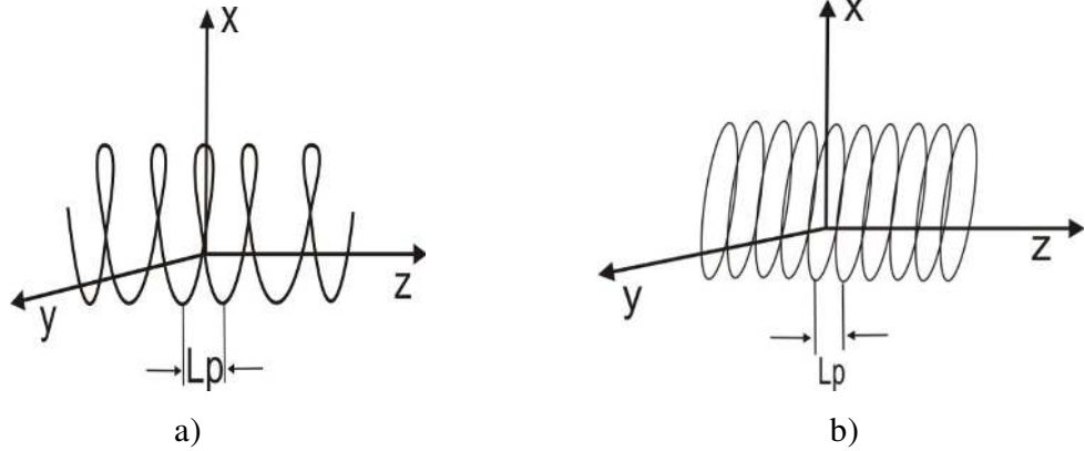
Şekil 2.7 Spiral (sarmal) şekilli (a) ve çevresel periyodik sarımlı (b) solenoidin prensip şeması.
