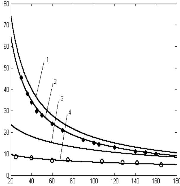
Şekil 3.4. Topların(1,2) manyetik geçirgenliği ve polyball yataklarının(3,4) ortalama manyetik geçirgenliği arasındaki ilişkinin tahmini yüzeyel manyetik alan yoğunluğuna karşı:1,3-[4,17],2,4, eq.(19) dan hesaplanan ● ve ○ - deneysel tarihler[17]
