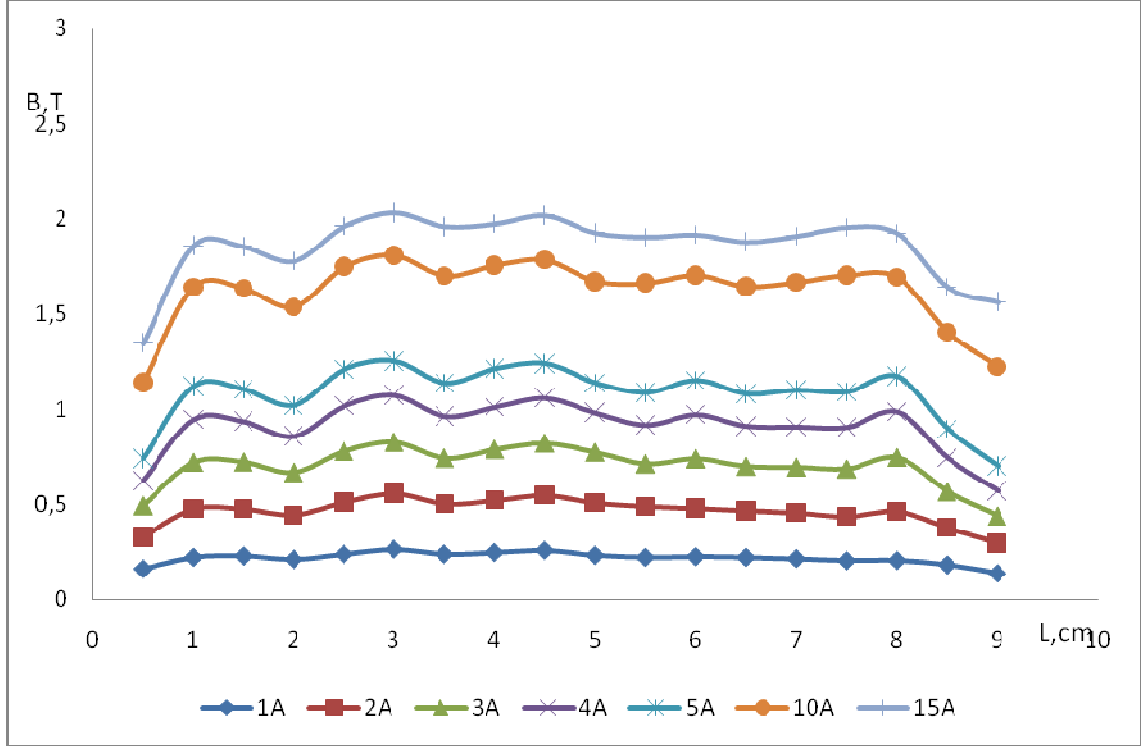
Şekil 4.3. Çapı d=6,28\text{mm} olan ferromanyetik bilyelerden oluşturulmuş dolgulu yatakların mıknatıslanma özelliklerinin deneysel incelemelerinin sonuçlarına göre 17 farklı noktada ölçülen B manyetik alan yoğunluğunun filtre boyunca uzunluğa bağlı değişim değerleri.
