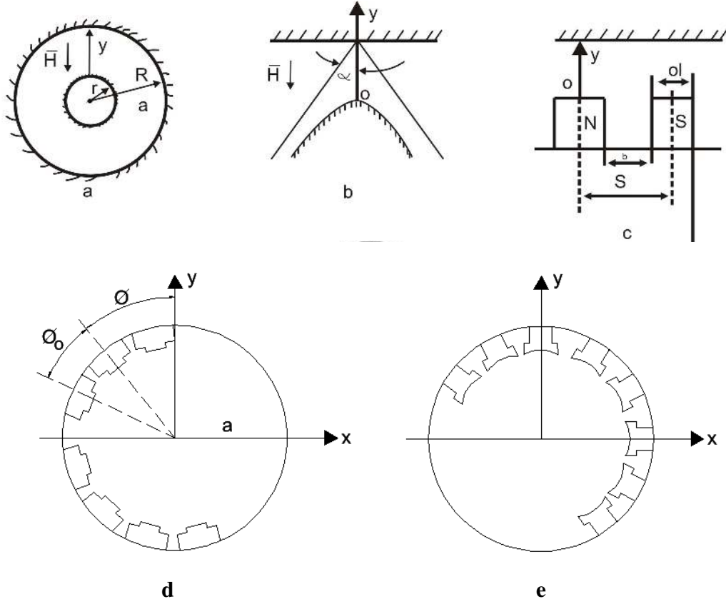
Şekil 2.9 Kutup şekillendirilmeleriyle oluşturulmuş gradyanlı manyetik alanlar a) halka şekilli boşluk b) Hiperbolik kutup-düzlem ikilisi; c) Birbirini seri izleyen açık kutuplu sistem; d) Tambur tipi açık manyetik sistem; e) Çok kutuplu kapalı manyetik sistem.
