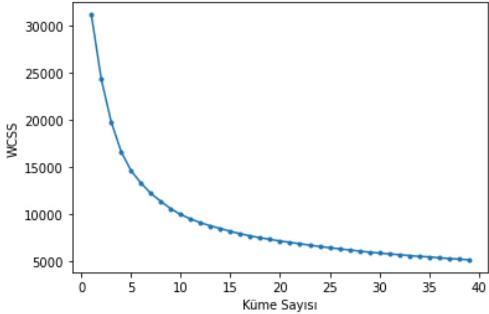
Şekil 5.13. Doc2vec Dirsek Grafiği
