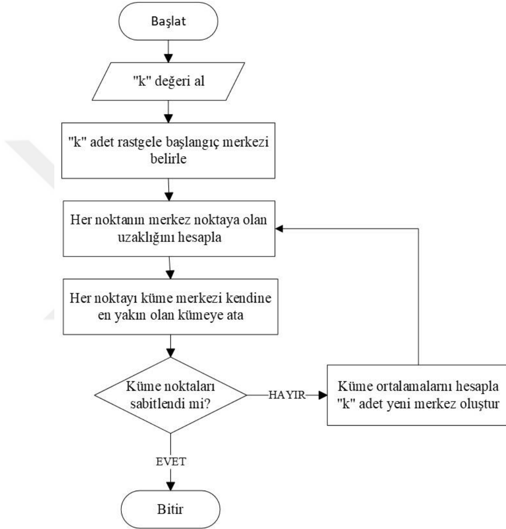
Şekil 2.5. K-Ortalamlar (K-Means) algoritması
