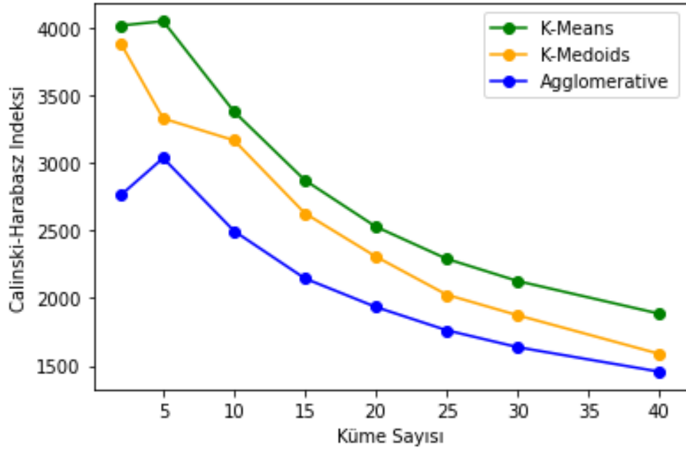
Şekil 5.16. Doc2vec CH İndeks
