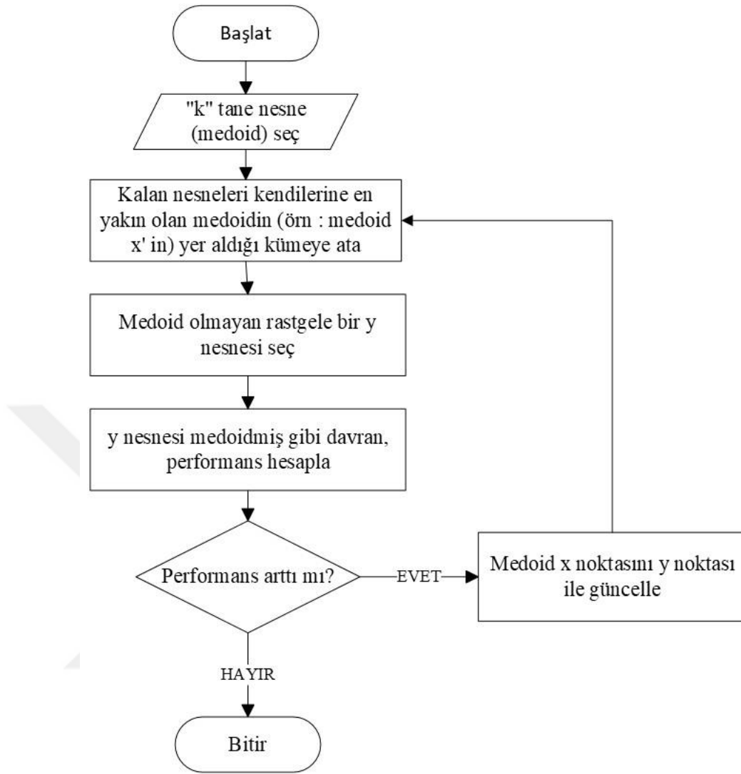
Şekil 2.6. K-Temsilci (K-Medoids) algoritması (Altıntaş, 2006)
