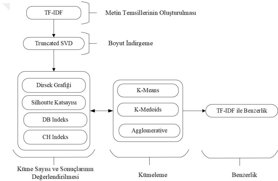
Şekil 5.2. TF-IDF senaryo akışı
