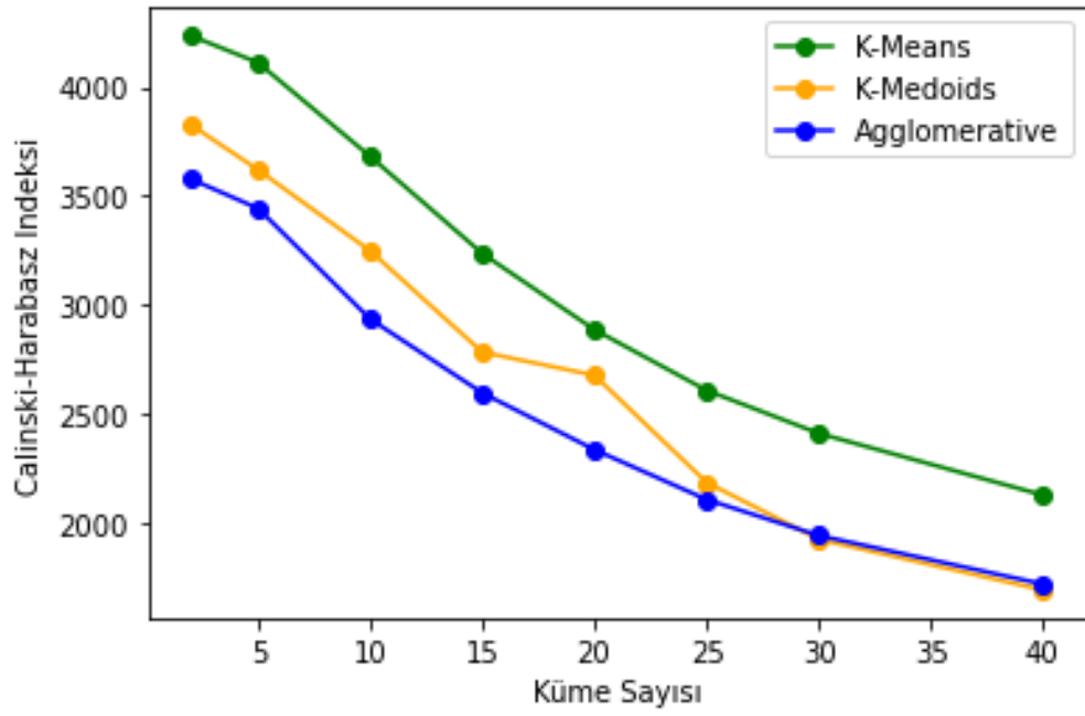
Şekil 5.12. Word2vec CH Index
