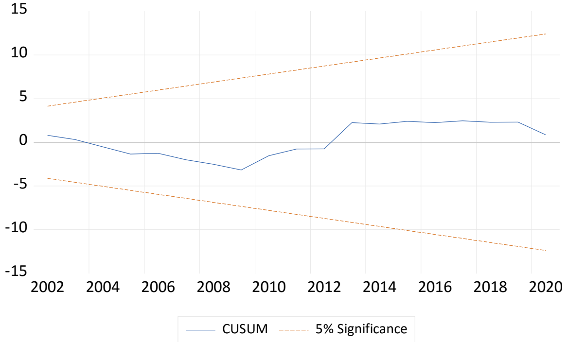
Şekil 8.1. Cusum Testi
