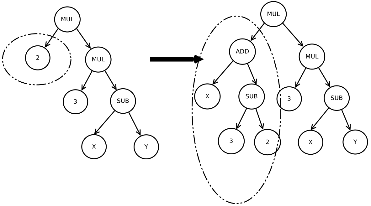
Şekil 2.13: Altağaç Mutasyonu
