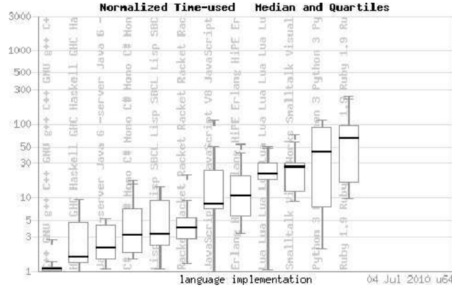
Şekil 2.15: x64 Mimarlı Intel® Q6600® İşlemciye Sahip GNU/Linux PC Üzerinde (Tek Çekirdekli) Bazı Gerçekleştirmelerin Çalışma Zamanı Kıyaslamaları
