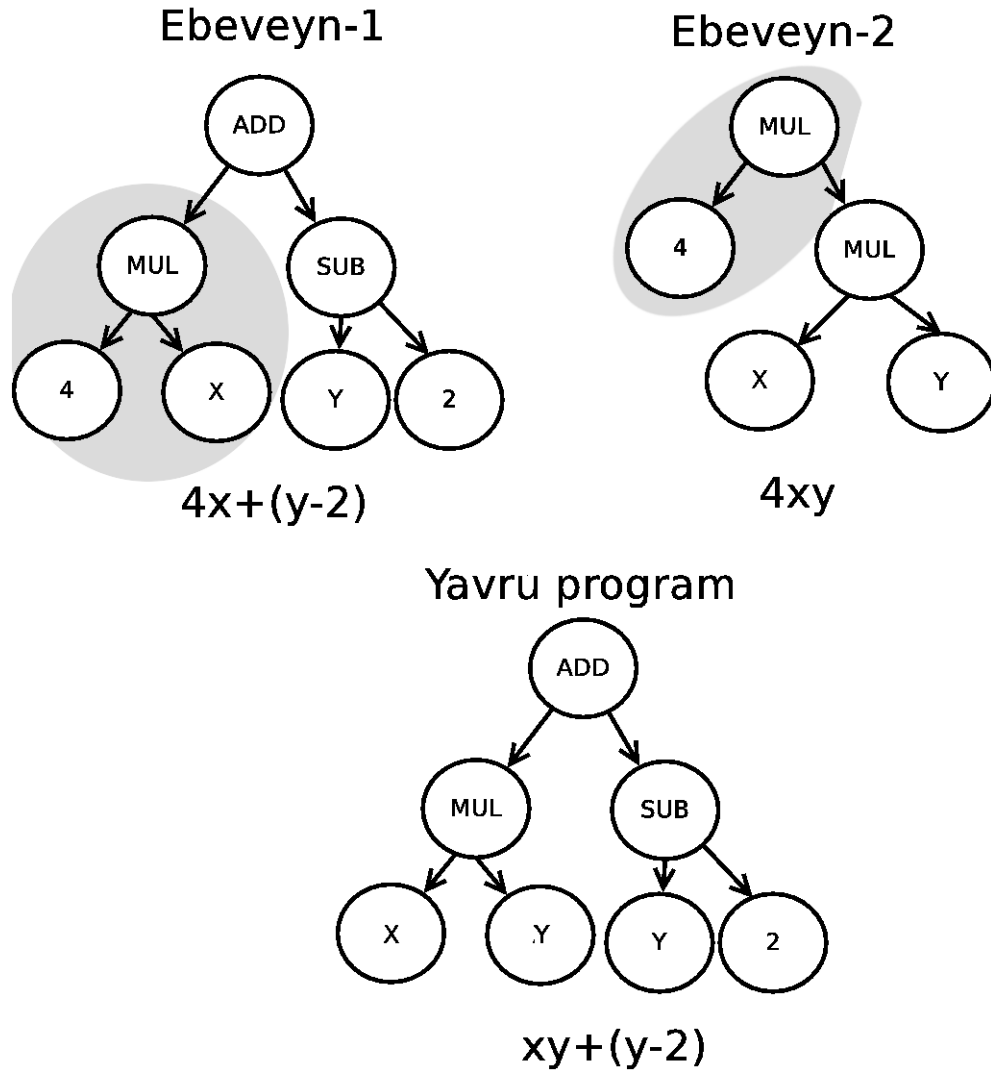
Şekil 2.12: Altağaç Çaprazlaması
