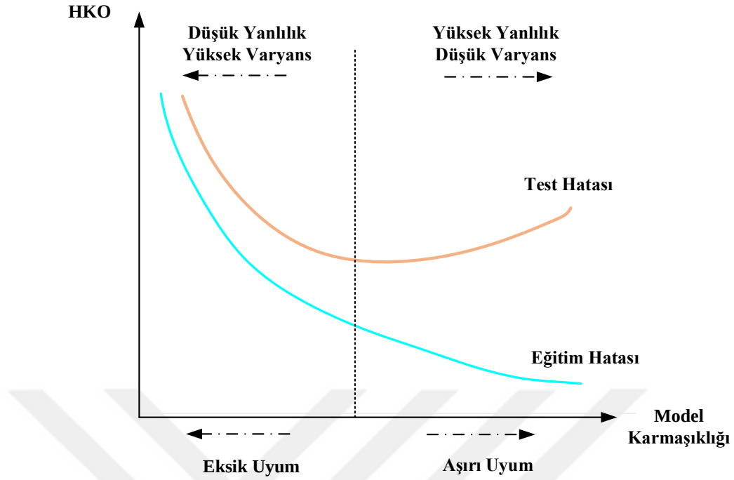
Şekil 1.5. Model karmaşıklığının eğitim ve test hatasına etkisi (Hastie ve diğerleri, 2008)
