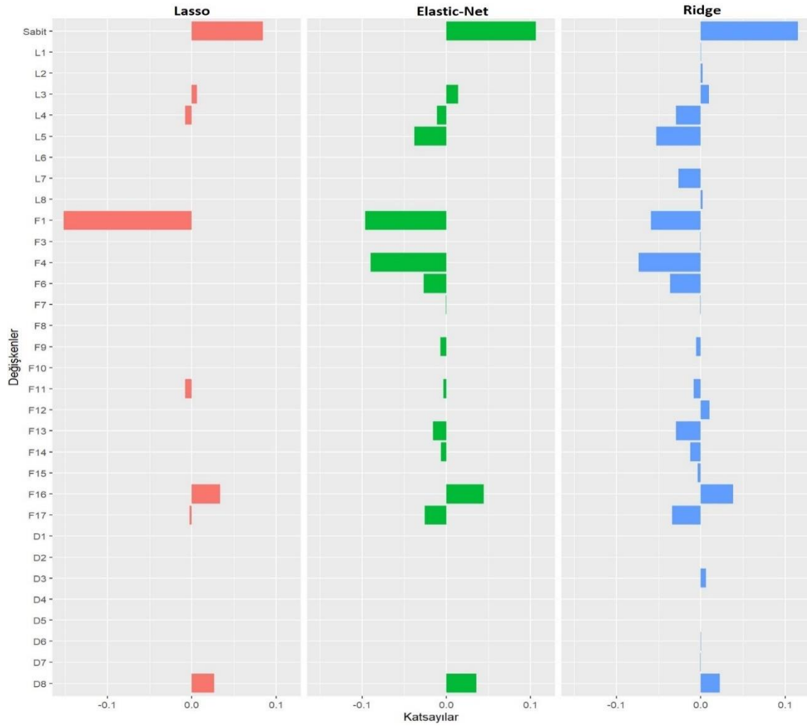
Şekil 4.9. Düzenlileştirici yöntemlerin katsayı tahminlerinin çubuk grafikleri
