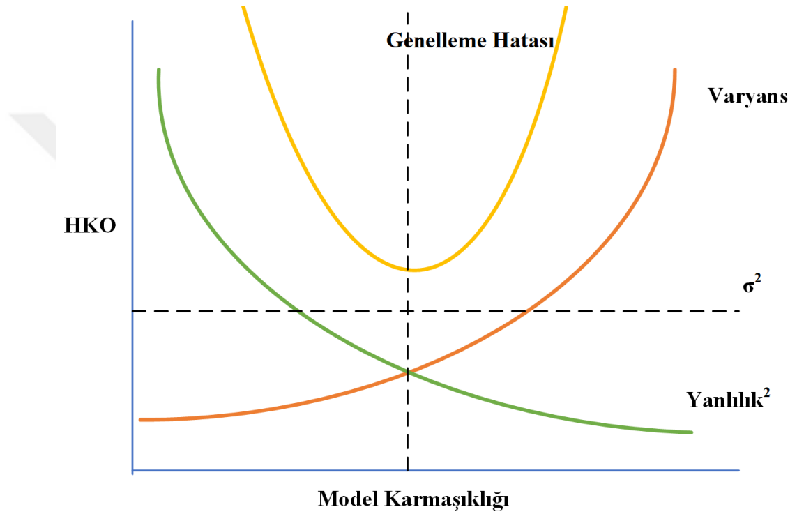
Şekil 1.4. Yanlılık-varyans ilişkisi (Genç, 2020)
