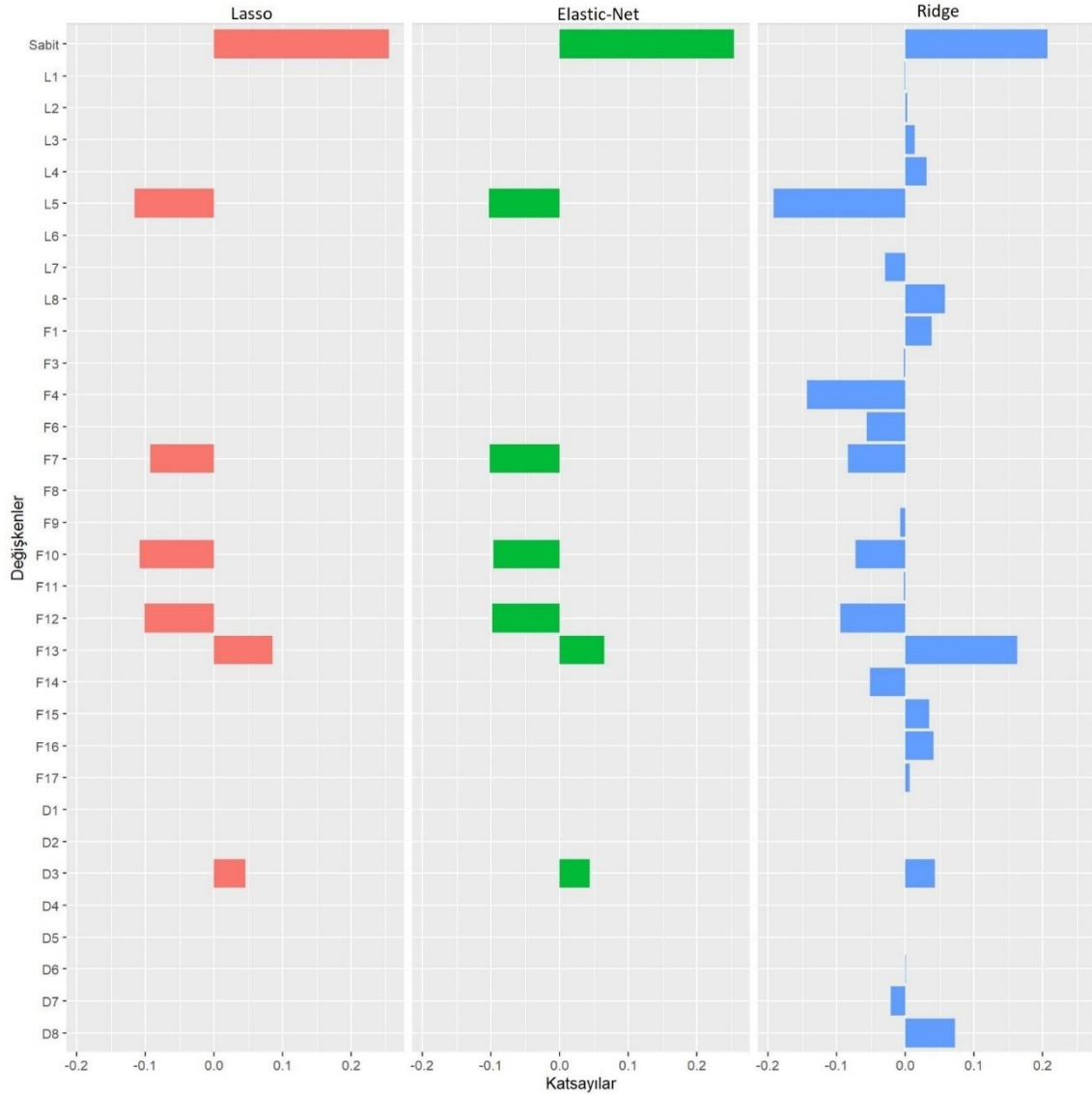
Şekil 4.22. Düzenleyici yöntemlerin katsayı tahminlerinin çubuk grafikleri
