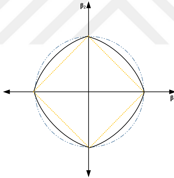
Şekil 3.6. Elastic Net tahmininin gösterimi (Zou ve Hastie, 2003).
