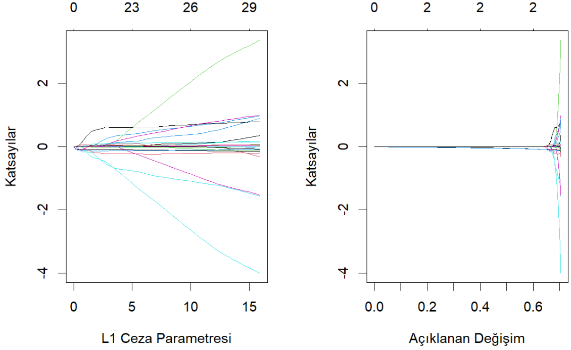
Şekil 4.23. Lasso katsayıların değişimi– Lasso açıklanan değişim
