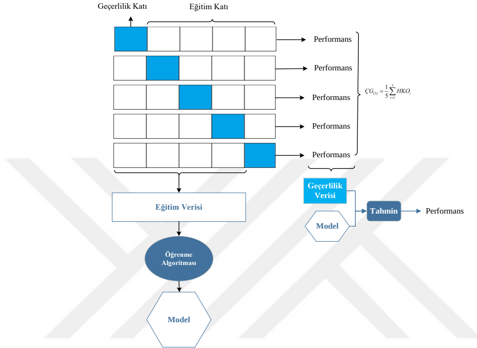
Şekil 1.8. 5-katlı çapraz geçerlilik yöntemi ile model değerlendirme (Raschka, 2018)
