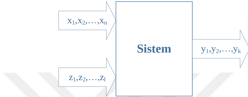
Şekil 1.2. Denetimli öğrenme problemi (Cherkassky ve diğerleri, 2012)
