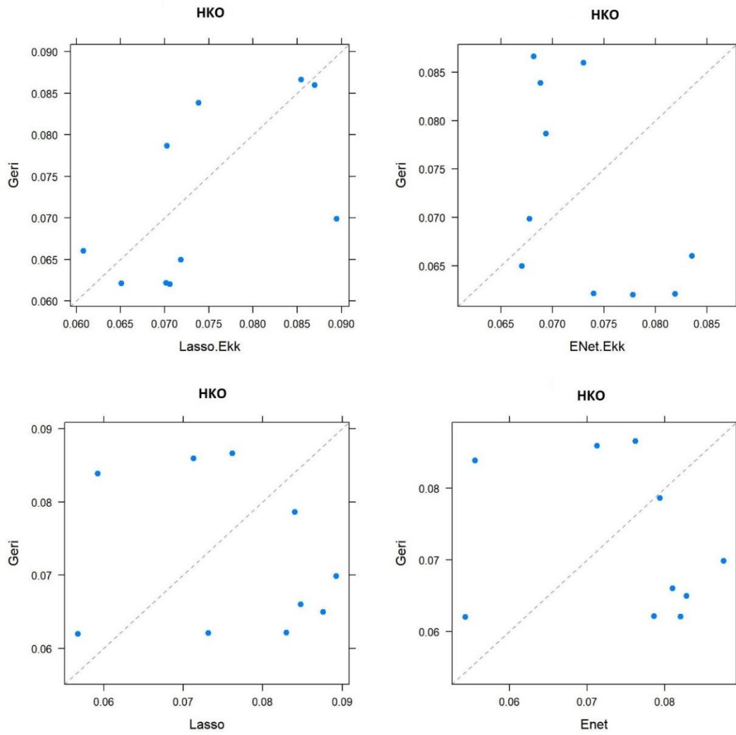
Şekil 4.16. Geriye doğru seçim yöntemi ÇG HKO sonuçlarının düzenlileştirici yöntemler ÇG HKO sonuçları ile karşılaştırılması
