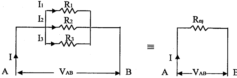
Şekil 2.56: Paralel bağlı dirençler
