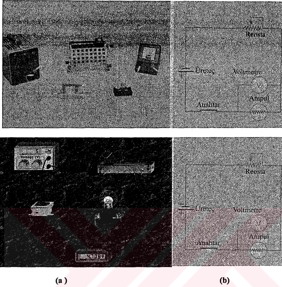
Şekil 4-61-a, b: Potansiyel farkı ölçülmesi ve devre şeması
