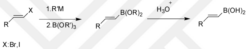
Şekil 2.11. Alkenil boronik asit sentezi
