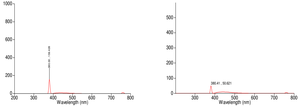
Şekil 4.28. pH 4’de Antrasen oksazon boronik asit, sialik asit ve sialik asit + hemaglutinin ile etkileşmesi sonucunda 380 nm’deki floresans spektrumları
