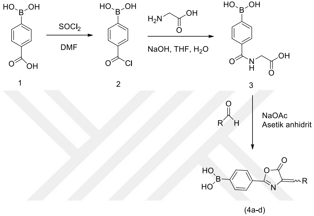
Şekil 3.1. Floresans prob taşıyan oksazolon Boronik asitlerin genel sentezi
