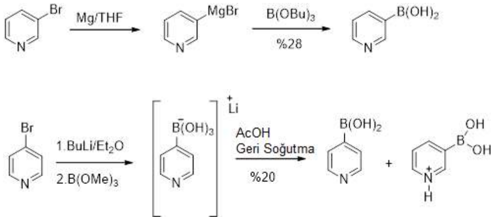
Şekil 2.9. 3- ve 4- piridil boronik asit sentezi
