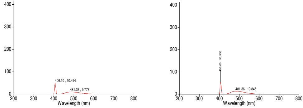
Şekil 4.22. pH 4’de Floren oksazolon boronik asit, sialik asit ve sialik asit + hemaglutinin ile etkileşmesi sonucunda 406 nm’deki floresans spektrumları
