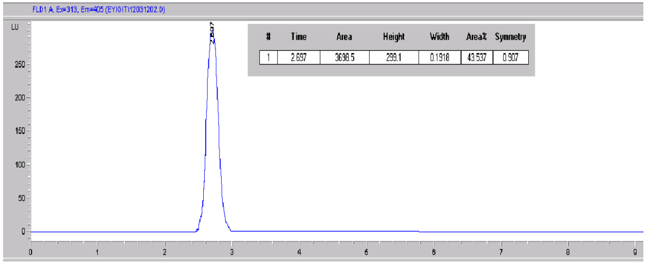
řekil 3.1. SA'nın alıkonma zamanı
