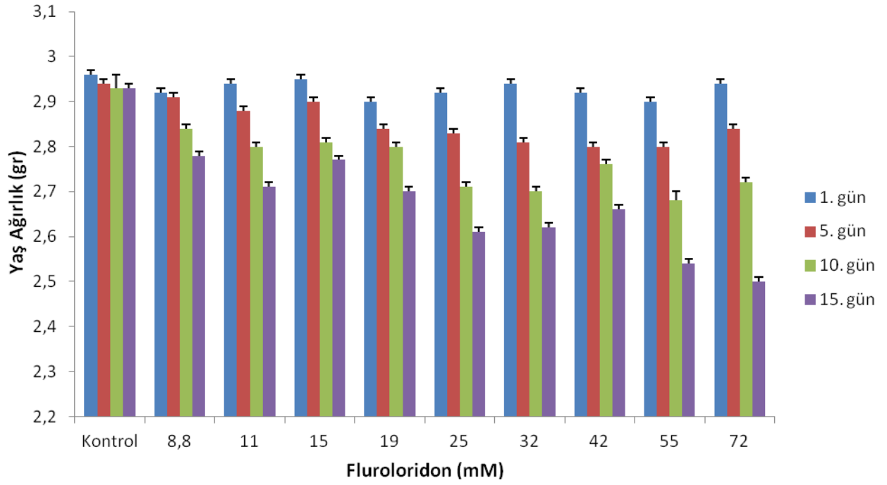
Ek Şekil 52. Çimlenme sonrası flurokloridon uygulanan V. sativa bitkisinde konsantrasyonlara ve günlere bağlı yaprak yaş ağırlığının değişimi
