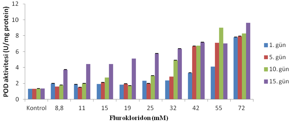
Ek Şekil 24. Çimlenme öncesi SA ve çimlenme sonrası flurokloridon uygulanan H. annuus yapraklarında konsantrasyonlara ve günlere bağlı POD aktivitesinin değişimi
