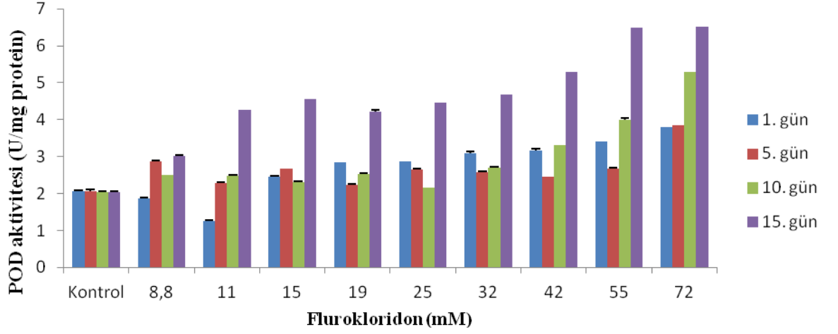
Ek Şekil 23. Çimlenme sonrası flurokloridon uygulanan H. annuus yapraklarında konsantrasyonlara ve günlere bağlı POD aktivitesinin değişimi
