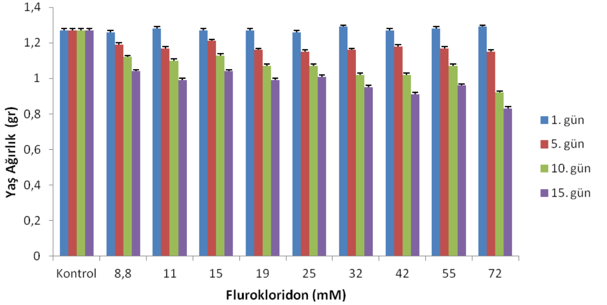
Ek Şekil 57. Çimlenme öncesi SA ve çimlenme sonrası flurokloridon uygulanan V. sativa bitkisinde konsantrasyonlara ve günlere bağlı kök yaş ağırlığının değişimi
