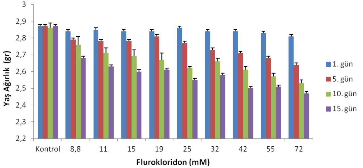
Ek Şekil 55. Çimlenme öncesi SA ve çimlenme sonrası flurokloridon uygulanan V. sativa bitkisinde konsantrasyonlara ve günlere bağlı gövde yaş ağırlığı değişimi
