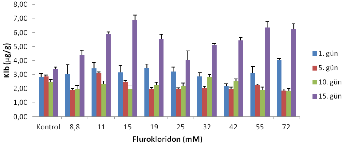
Ek Şekil 4. Çimlenme öncesi SA ve çimlenme sonrası flurokloridon uygulanan H. annuus yapraklarında konsantrasyonlara ve günlere bağlı Kl b miktarlarının değişimi
