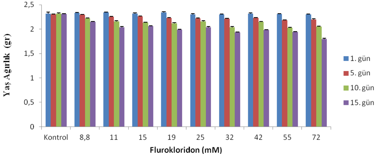
Ek Şekil 53. Çimlenme öncesi SA ve çimlenme sonrası flurokloridon uygulanan V. sativa bitkisinde konsantrasyonlara ve günlere bağlı yaprak yaş ağırlığı değişimi
