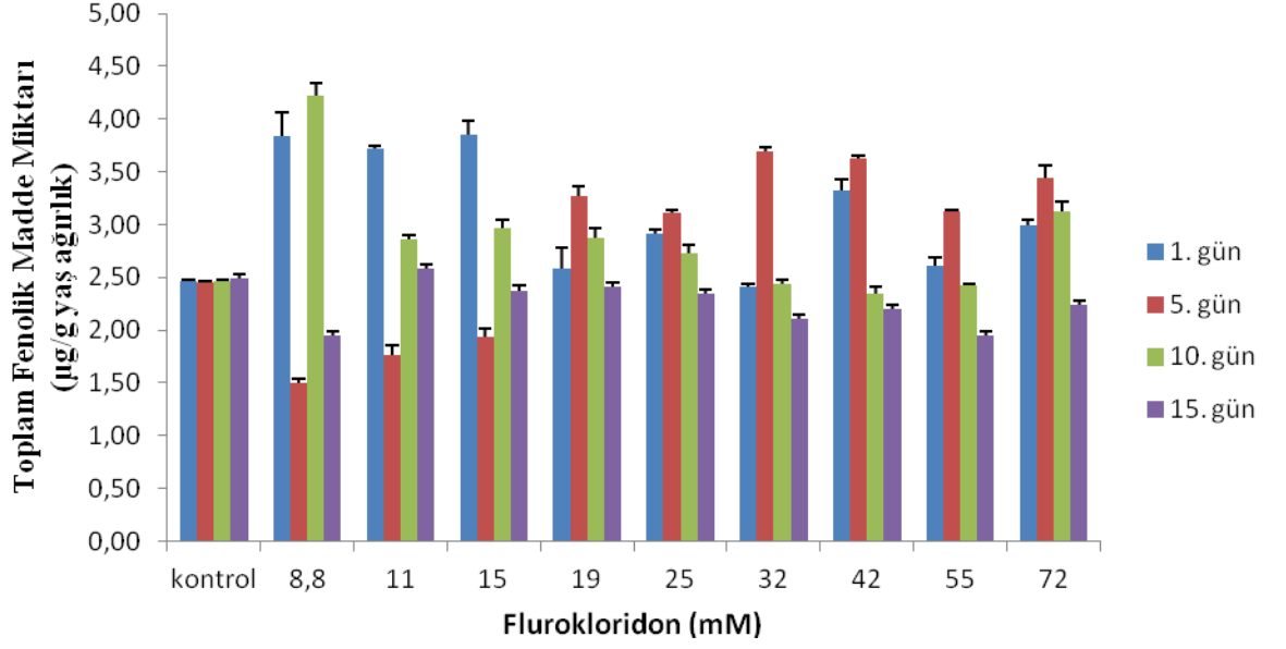
Ek Şekil 39. Çimlenme sonrası flurokloridon uygulanan H. annuus yapraklarında konsantrasyonlara ve günlere bağlı toplam fenolik madde içeriğinin değişimi
