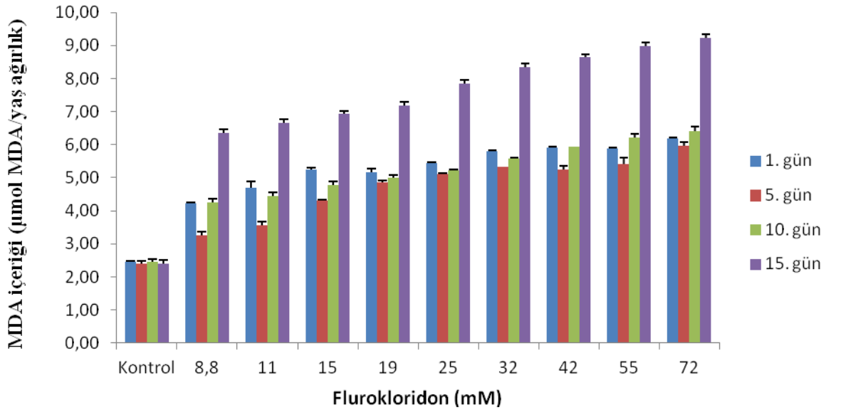
Ek Şekil 38. Çimlenme öncesi SA ve çimlenme sonrası flurokloridon uygulanan H. annuus yapraklarında konsantrasyonlara ve günlere bağlı MDA içeriğinin değişimi
