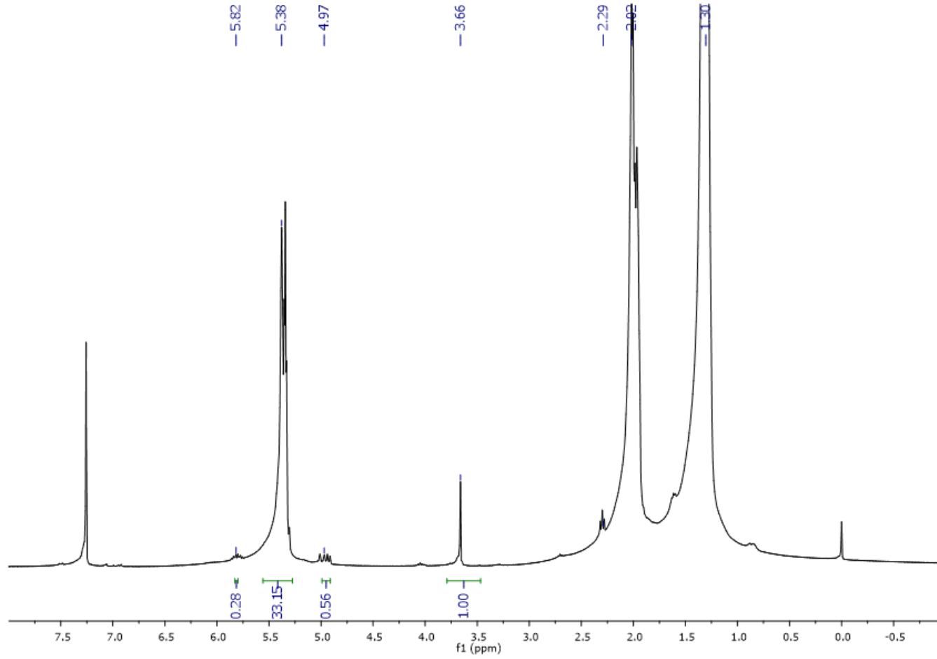
Ek1. COE/MU/G1; 500/5/1 oranı kullanılarak hazırlanan polisikloktan bileşiğinin 1 H NMR (400 MHz, CDCl 3 , 23 °C) spektrumu (Tablo 2, Deney 2, Mn(NMR): 6600 Da, MF %84; DF %16)
