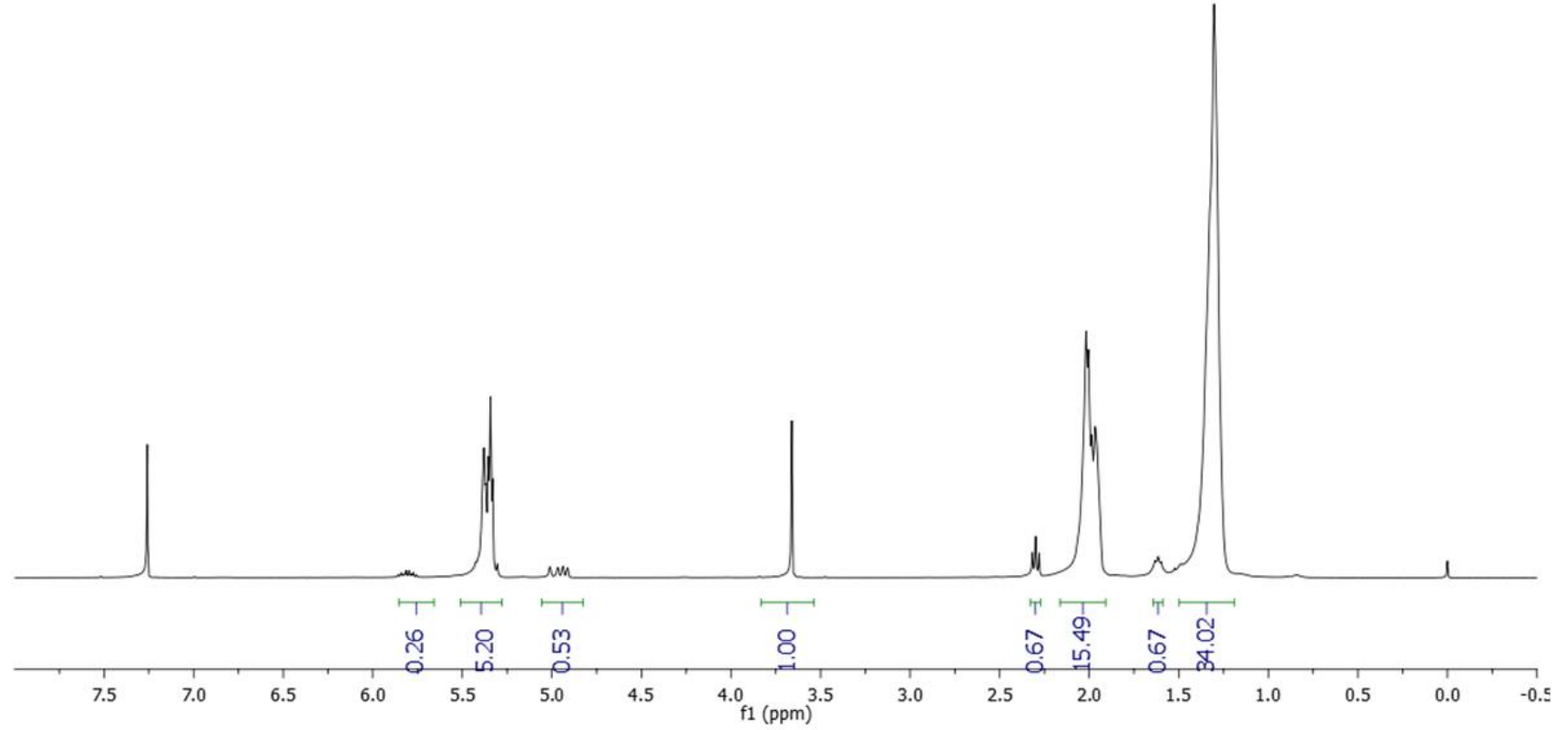
Ek9. COE/MU/G1; 1000/40/1 oranı kullanılarak hazırlanan polisikloktan bileşiğinin ^1\text{H} NMR (400 MHz, \text{CDCl}_3 , 23 °C) spektrumu (Tablo 2, Deney 11, Mn: 1300 Da, MF %75; DF %25)
