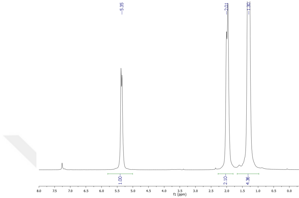
Çizelge 3. COE/MU/G1; 500/2/1, koşullarında elde edilen CNF COE polimerinin ^1\text{H} NMR spektrumu (400 MHz, \text{CDCl}_3 , 23 °C)
