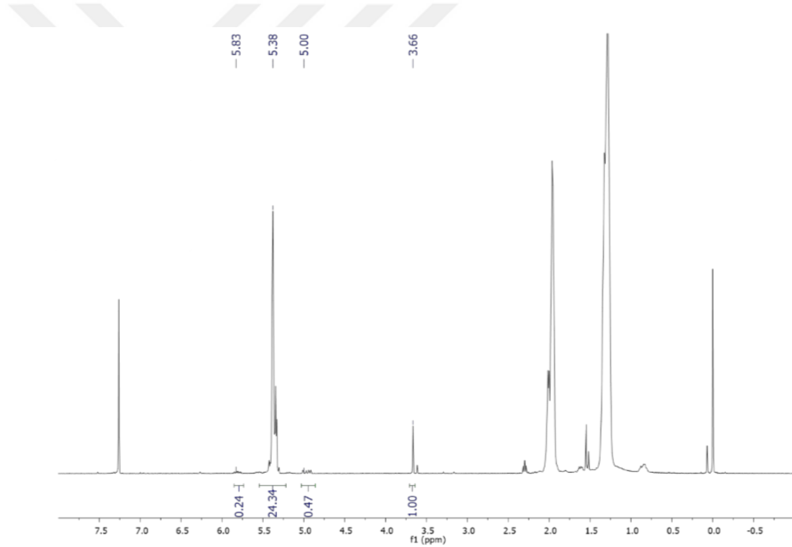
Ek6. COE/MU/G1; 1000/10/1 oranı kullanılarak hazırlanan polisikloktan bileşiğinin 1 H NMR (400 MHz, CDCl 3 , 23 °C) spektrumu (Tablo 2, Deney 8, Mn: 5400 Da, MF %72; DF %28)
