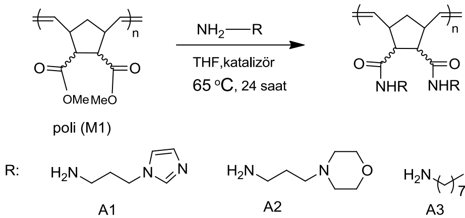
Şekil 15. Sübstitüye amit grupları taşıyan fonksiyonel ROMP polimerleri
