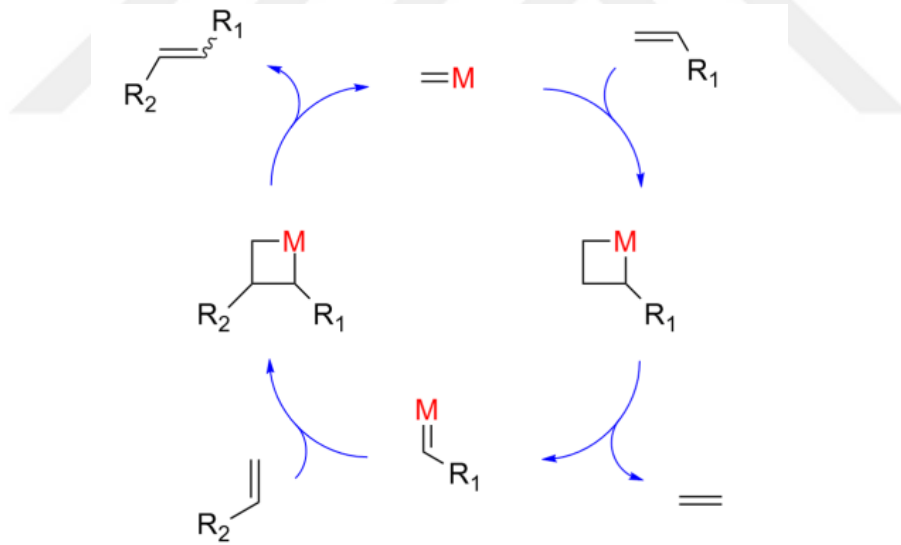
Şekil 4. Chauvin'in olefinin metatez tepkimesinin mekanizması
