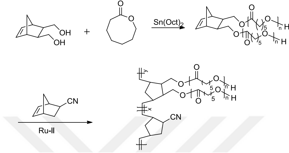
Şekil 20. Kaprolakton ve siyano grubu içeren ROMP polimerleri
