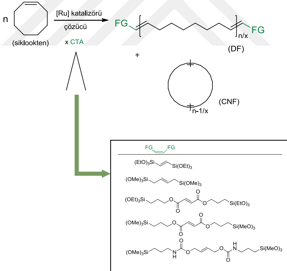
Şekil 24. Siloksan grubu içeren iç olefinler ile COE'nin ROP/CM reaksiyonları
