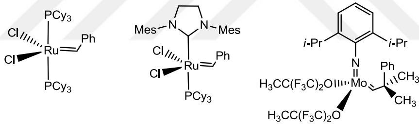
Şekil 6. ROMP/CM reaksiyonlarında kullanılan literatürde iyi tanımlanmış katalizörler
