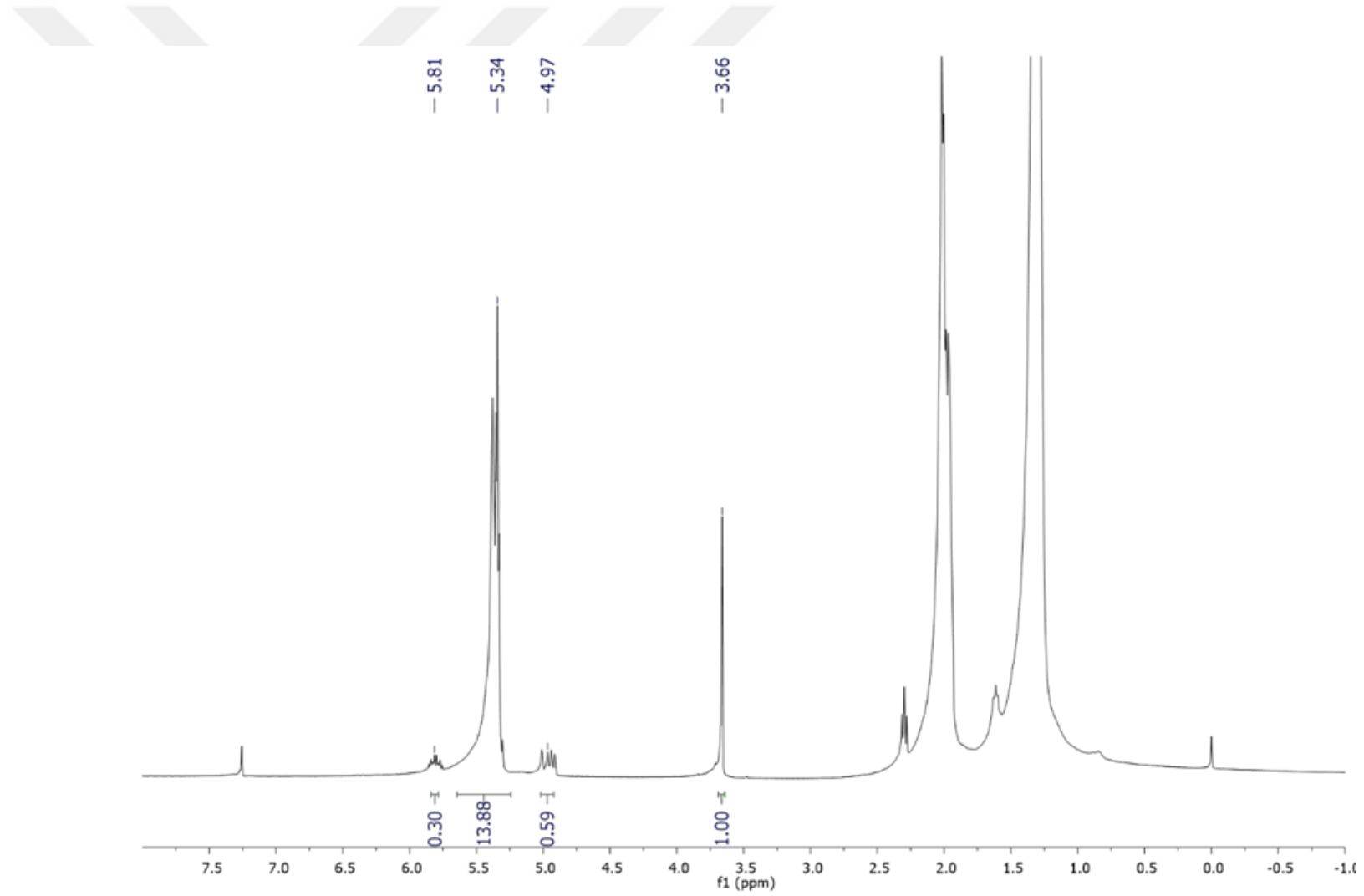
Ek3. COE/MU/G1; 500/20/1 oranı kullanılarak hazırlanan polisikloktan bileşiğinin ^1\text{H} NMR (400 MHz, \text{CDCl}_3 , 23 °C) spektrumu (Tablo 2, Deney 4, Mn: 2800 Da, MF %90; DF %10)
