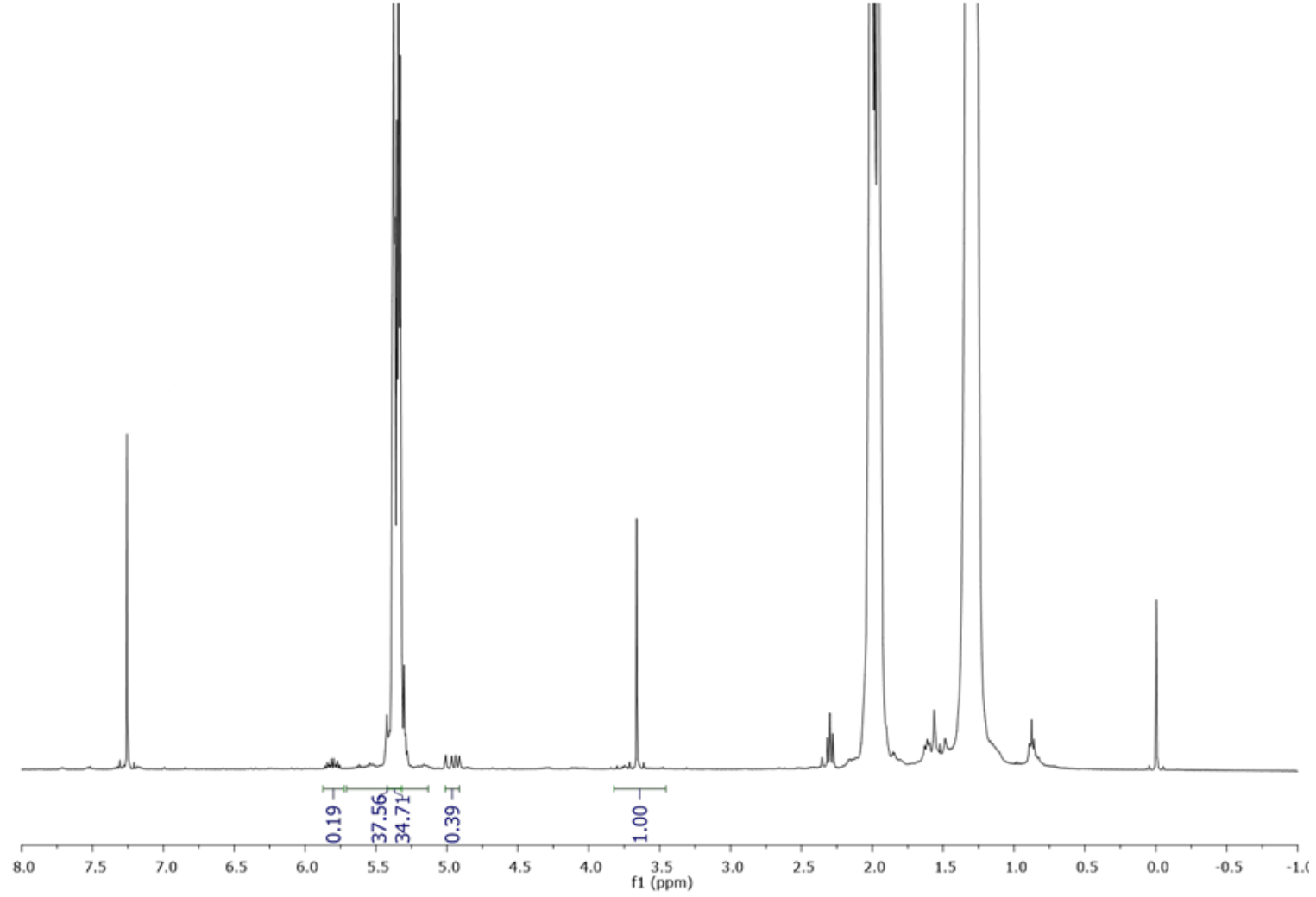
Ek5. COE/MU/G1; 1000/5/1 oranı kullanılarak hazırlanan polisikloktan bileşiğinin ^1\text{H} NMR (400 MHz, \text{CDCl}_3 , 23 °C) spektrumu (Tablo 2, Deney 7, Mn: 17300 Da, MF %57; DF %43)
