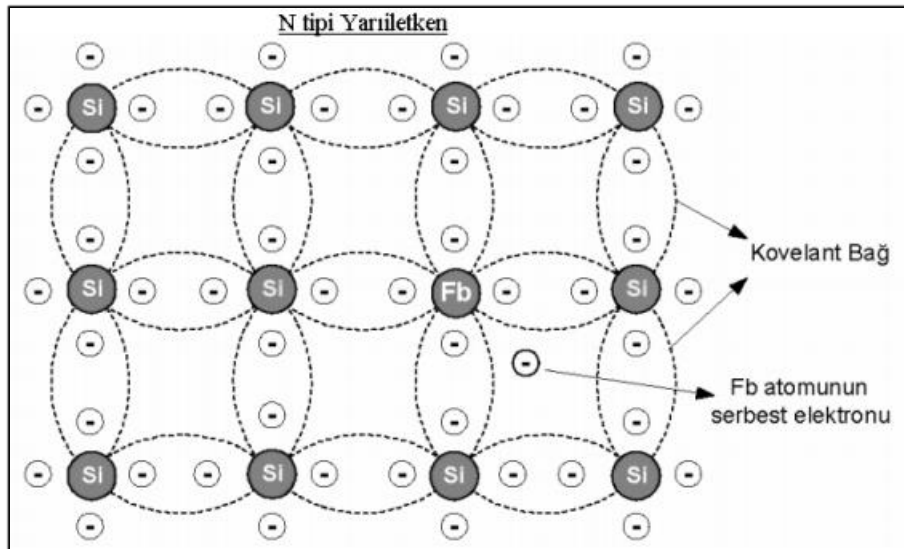
Şekil 3.11. N Tipi Yarıiletkenlerin Oluşturulması
