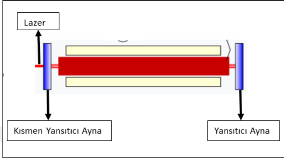
Şekil 3.8. Lazer tüpünün yapısı
