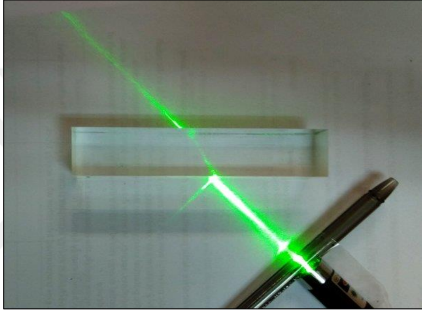
řekil 2.4. Işıhta kırılma
