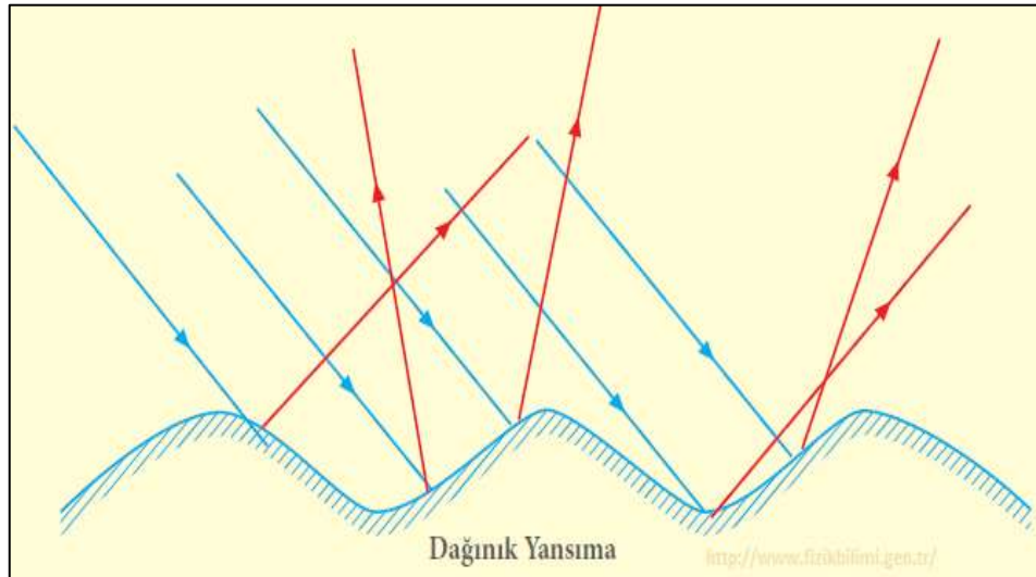
Şekil 2.3. Işıқта dağınık yansımada
