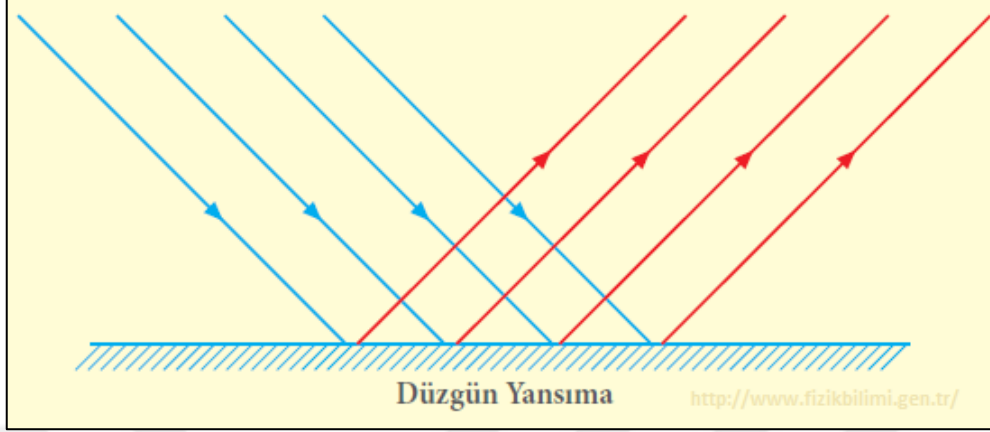
Şekil 2.2. Işıқта düzgün yansımada
